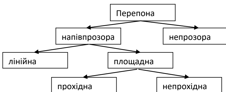
Рис. 1. Класифікація перепон PPX моделі робочої зони RTLS-системи
