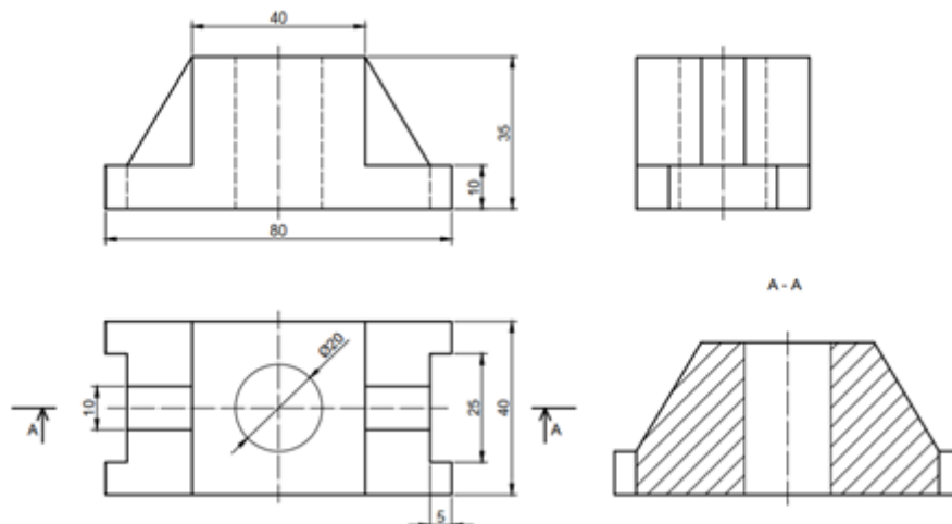
Рис. 1. Креслення деталі в AutoCAD за Методом прямокутних проєкцій
