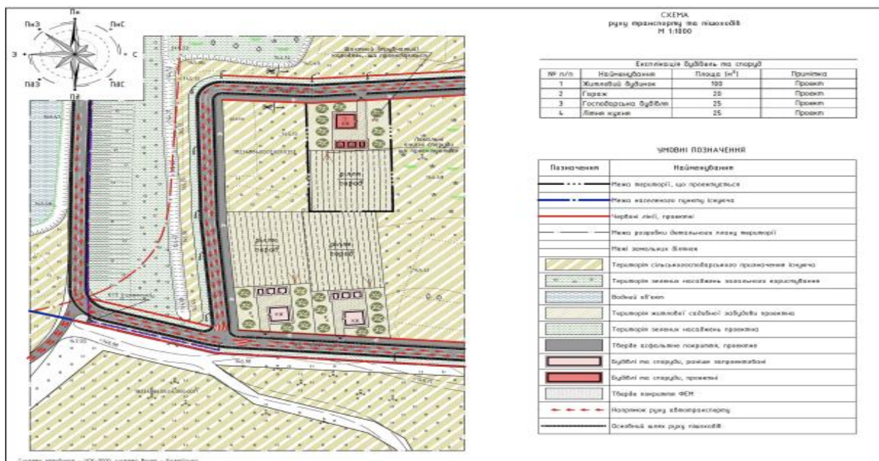
Рис.2. Схема руху транспорту та пішоходів М 1:1000 [8]
