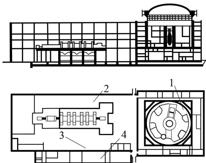
Рисунок 1 – Блок ВВЕР:
