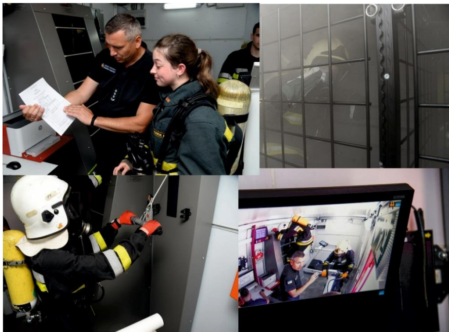
Рисунок 2 – Проведення тренувань газодимозахисників у тренувальному комплексі MAW-Contaneranlage
