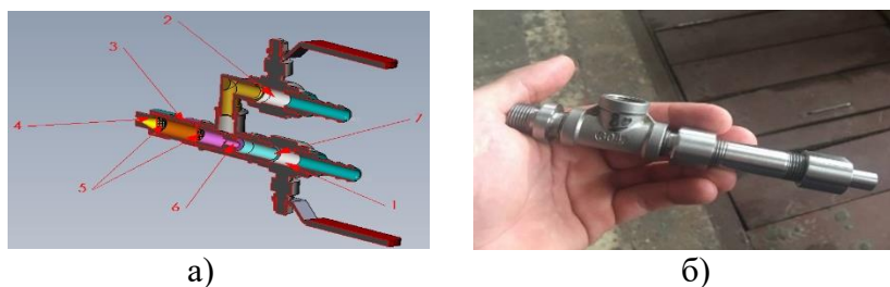
Рисунок 2 – Ствол для генерування та подавання компресійної піни: а) 3D-модель; б) фото зразка ствола у розрізі, де: 1 – дросель регулювання витрати водного розчину піноутворювача; 2 – дросель регулювання витрати стиснутого повітря; 3 – піногенератор; 4 – сопло; 5 – пакети сіток; 6 – змішувач; 7 – втулка
