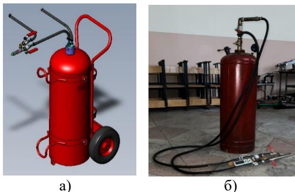
Рисунок 1 – Система генерування та подавання компресійної піни для гасіння лабораторних вогнищ: а) 3D-модель; б) фото зразка
