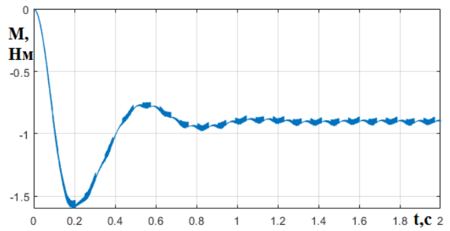
Рисунок 3 – Перехідний процес електромагнітного моменту АГ
