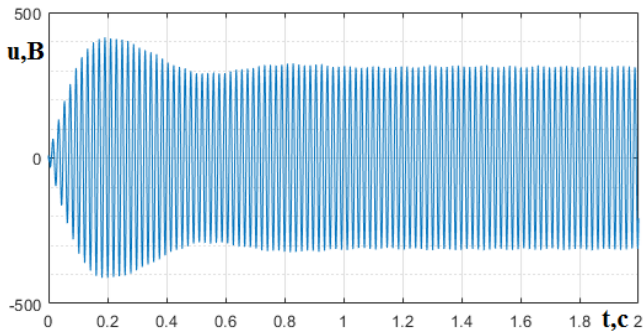
Рисунок 2 – Перехідний процес фазної напруги
