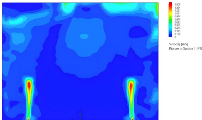
Рисунок 1 – Швидкість пінних струменів
