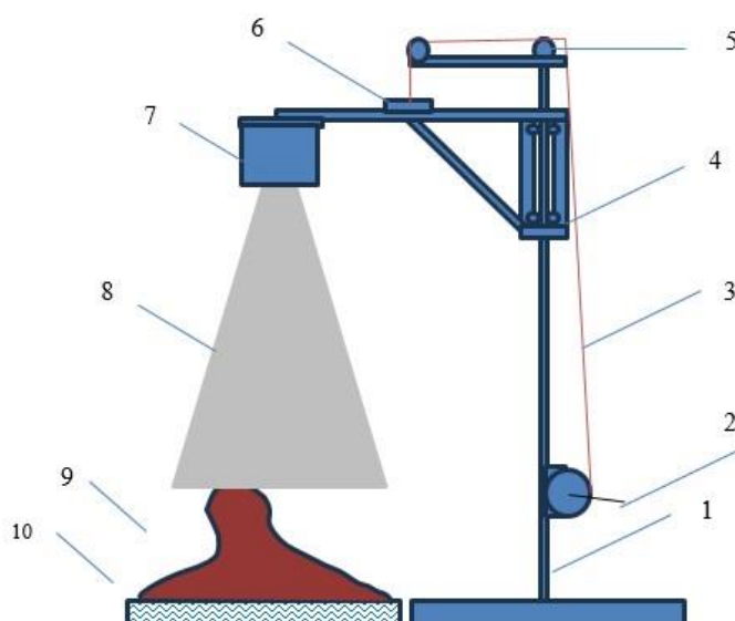
Рисунок 1 – Установка для визначення параметрів гасіння вогнегасним аерозолем горючих рідин на відкритому просторі.
