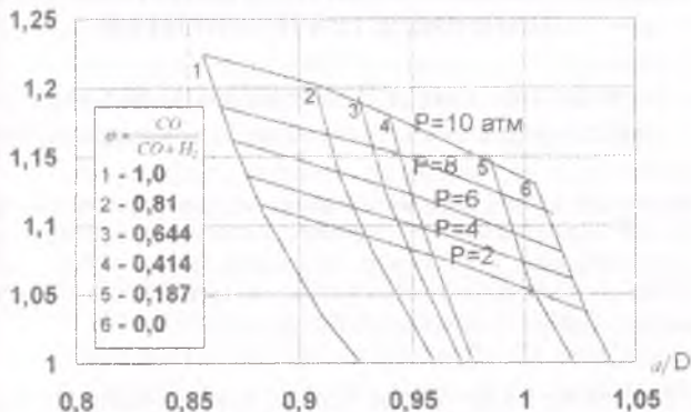
Рисунок 1 – Зависимость относительных нижних КППП ( C''_{отн} ) от отношения коэффициента температуропроводности ( \alpha ) к коэффициенту диффузии ( D ), изменяющихся от начального давления ( P ) и значения ( \phi )
