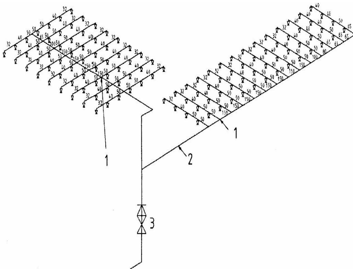
Рисунок 13. Приклад вибору розрахункових точок у секції, яка захищає приміщення класу НН, із розмірами трубопроводів згідно з табл. 13 і 14
