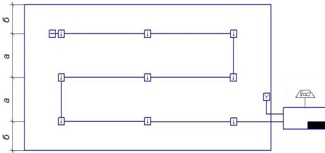
Рисунок 7. Схема розробленої СПС
