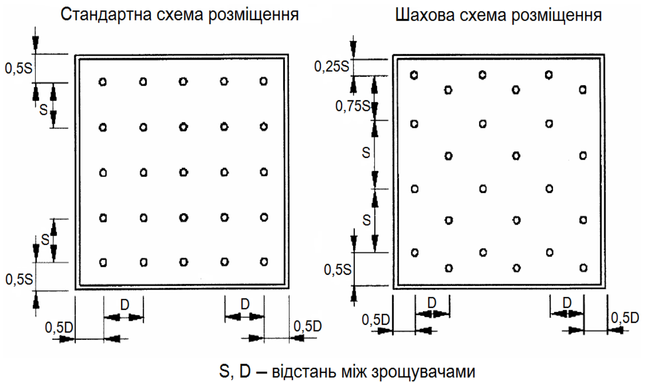
Рисунок 9. Розміщення стельових зрошувачів
