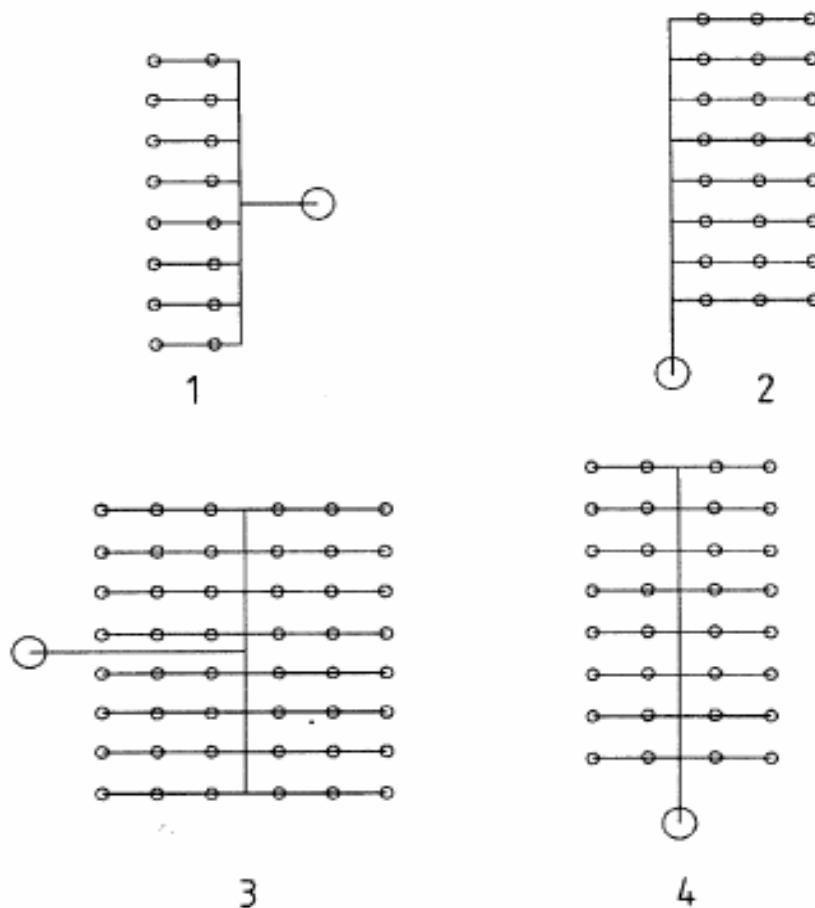
Рисунок 10. Приклади мереж розподільних трубопроводів
