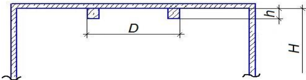
Рисунок 5. Співвідношення щодо висоти приміщення та висоти балки
