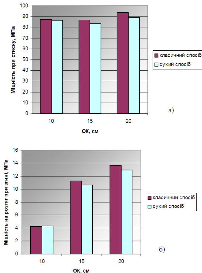
Рисунок 7.9 - Зміна міцності при стиску (а) та міцності на розтяг при згині (б) дрібнозернистого сталевібробетону у віці 28 дів в залежності від способу введення фібри та рухомості суміші
