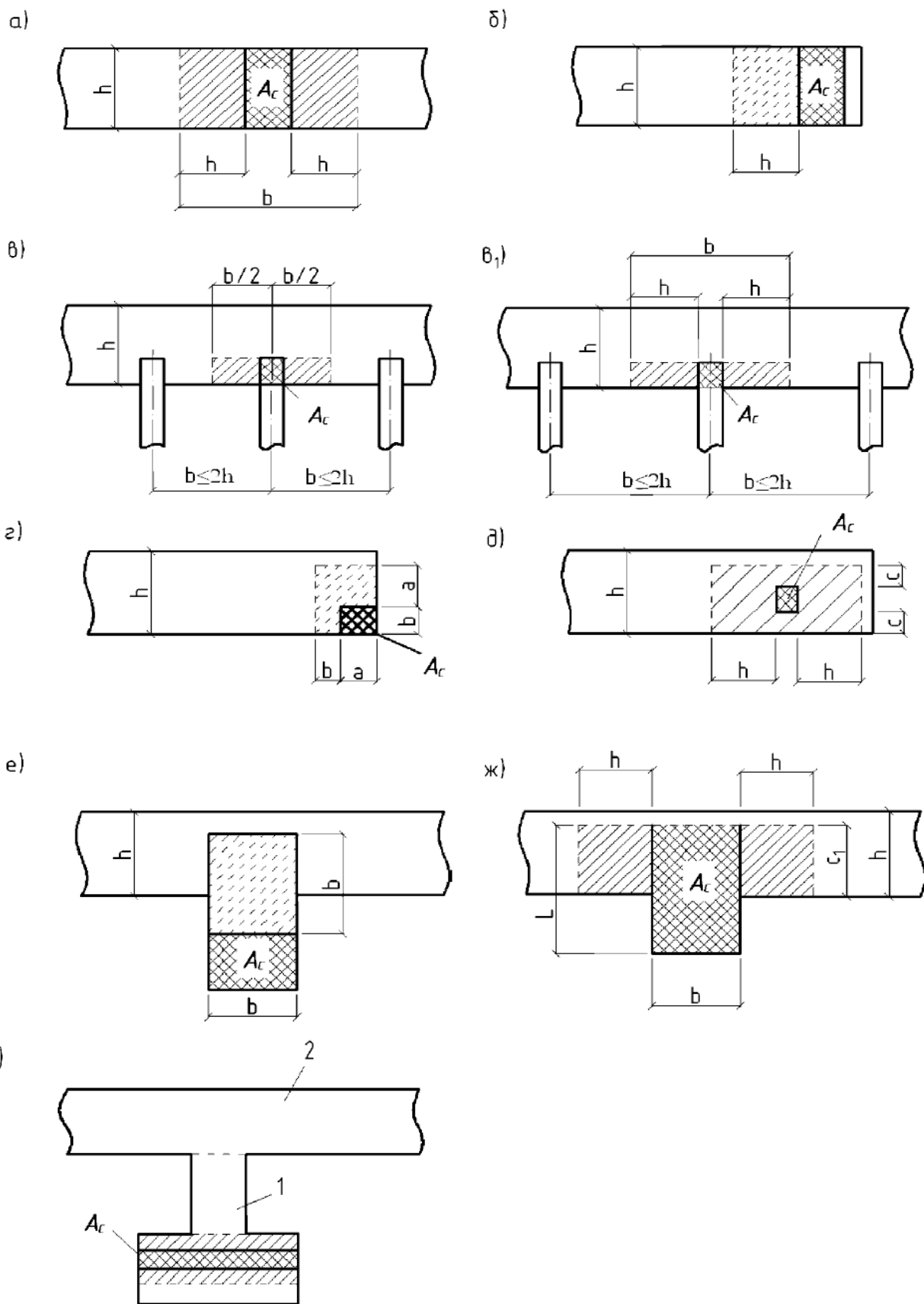
Рисунок 6.2.2 – Визначення розрахункових площ при місцевому стиску.
