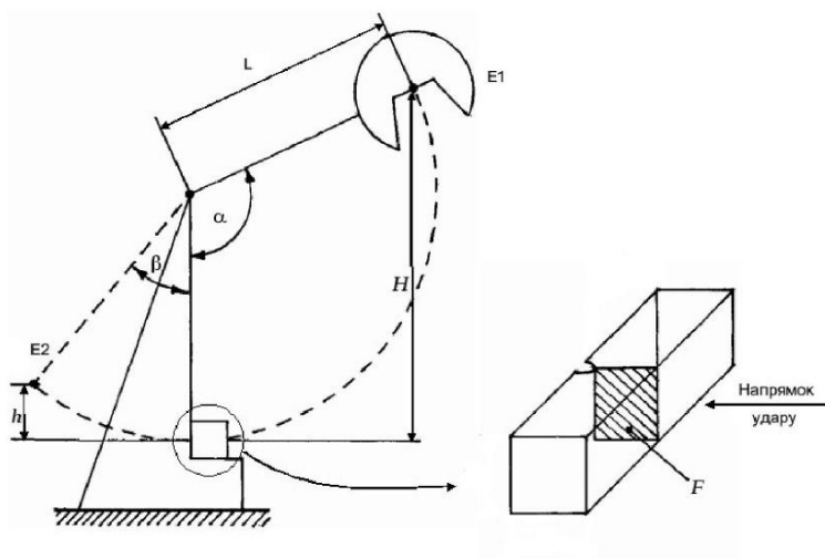
Рис. 7.4 – Загальний вигляд маятникового копра МК-30А (а) та схема випробування на ударну в'язкість (б)
