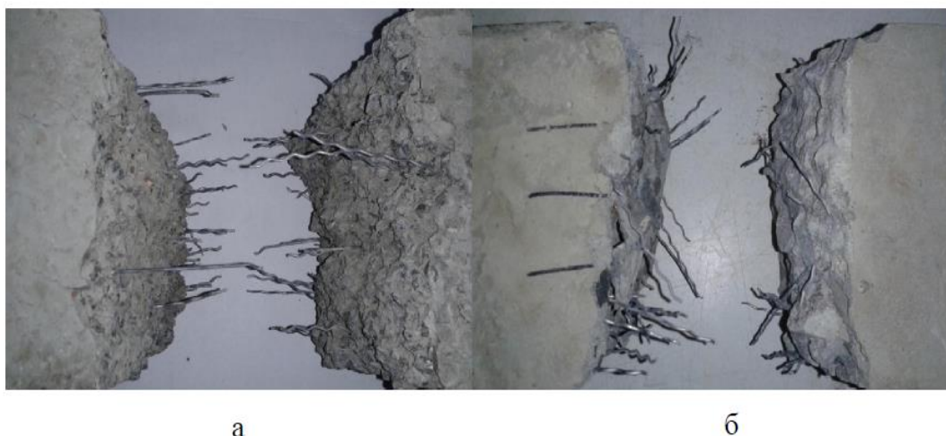
Рисунок 7.10 – Вигляд перерізу зруйнованого зразка із орієнтованою (а) та неорієнтованою (б) фіброю
