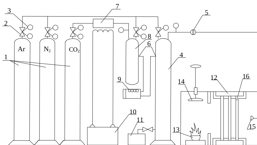
Рис. 1. Принципова схема лабораторного випробувального стенду: 1 – балон з газом; 2 – клапан; 3 – манометр; 4 – змішувач; 5 – пробковий клапан; 6 – термопар; 7 – випаровувач; 8 – накопичувач; 9 – регулювальний прилад; 10 – трансформатор; 11 – блок продувки; 12 – випробувальна камера; 13 – модельне вогнище; 14 – пристрій гасіння; 15 – завихрювач; 16 – зразки.
