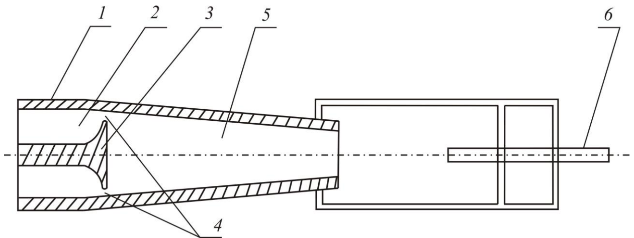
Рис. 1. Ствол з використанням кавітаційних ефектів для розпорощення струменя.
