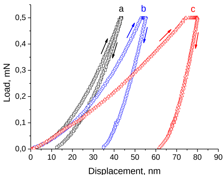
Рис. 1. Криві навантаження для систем \text{Nb}_2\text{O}_5/\text{Nb} з оксидними плівками завтовшки: a – 20 нм; b – 100 нм; c – 300 нм.
