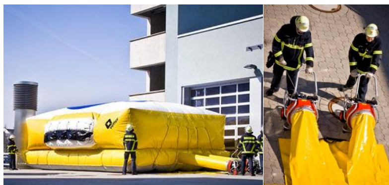
Рис. 2. Пневматична рятувальна подушка VETTER SP 60 вентиляторного типу.
