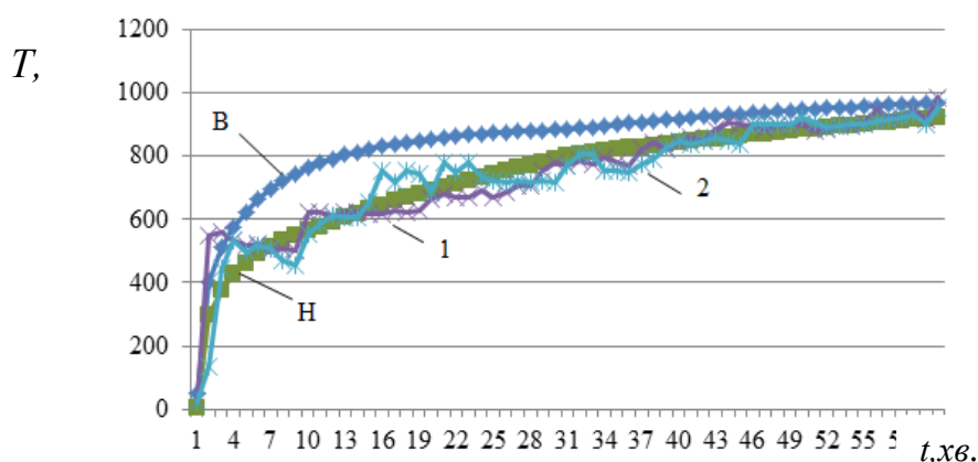
Рис. 2. Середня температура поверхні гофрованого профілю сталезалізобетонної плити: B, H – верхня та нижня межі стандартного температурного режиму; 1 – середня температура поверхні гофрованого профілю горизонтально розміщеної сталезалізобетонної плити; 2 – середня температура поверхні гофрованого профілю вертикально розміщеної сталезалізобетонної плити.
