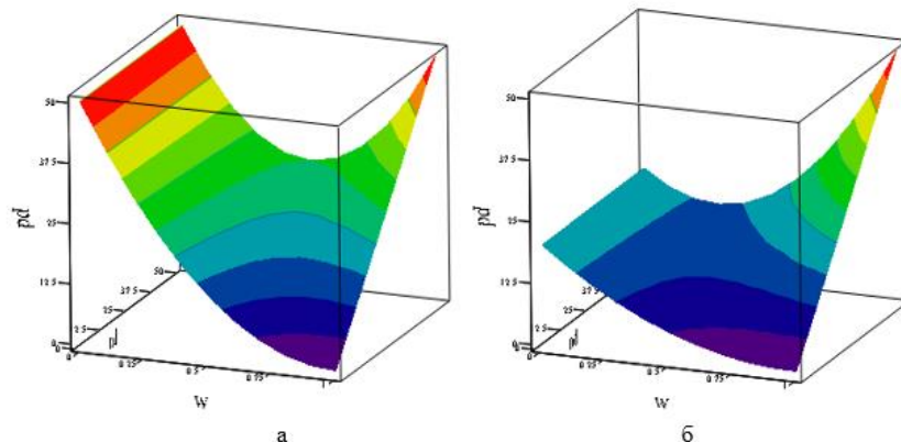
Рис. 1. Поверхні відгуку дисперсійної складової ВПЕ полімерних композитів \gamma_s^d від \omega та \gamma_p^d наповнювачів для полімерів з а – \gamma_p^d = 50 мДж/м 2 ; б – \gamma_p^d = 20 мДж/м 2 .
