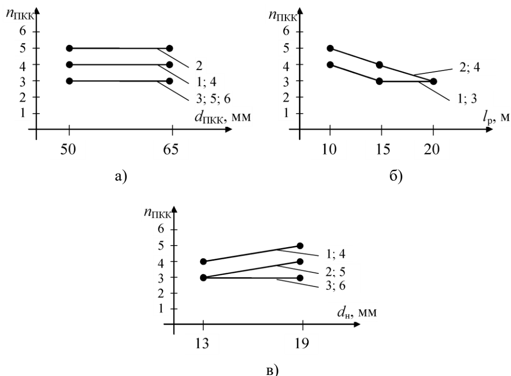
Рис. 1. Кількість ПКК n_{\text{ПКК}} на одному поверсі при проведенні розрахунків для графіків 1–6 в залежності від: а) діаметра ПКК d_{\text{н}} ; б) довжини рукава l_p ; в) діаметра насадка ствола d_{\text{н}} .
