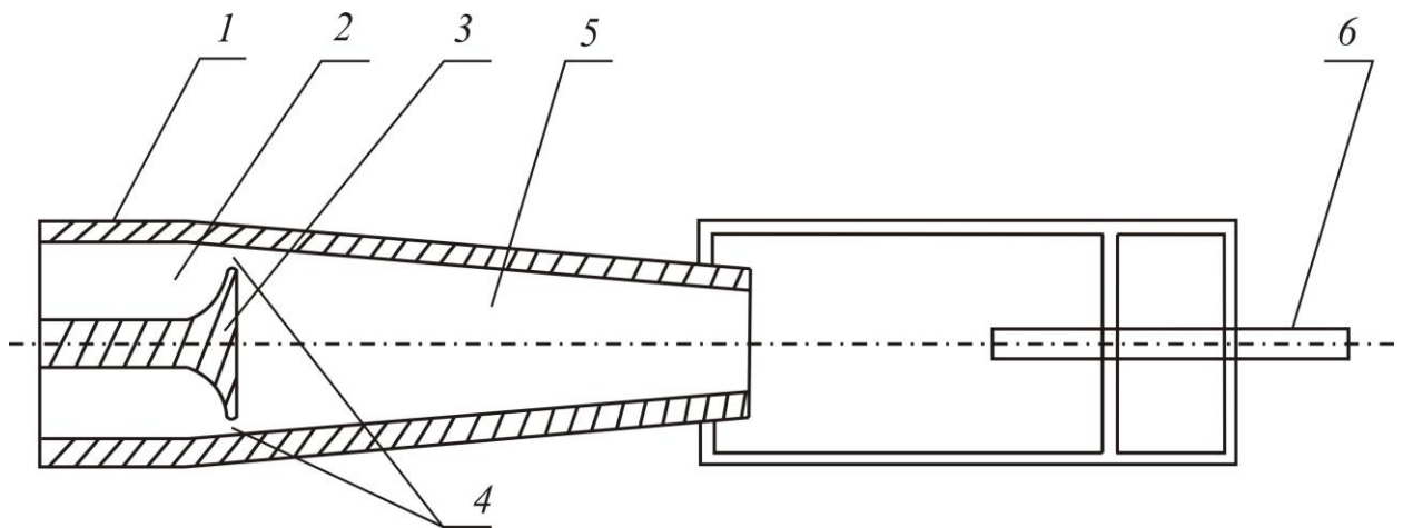
Рис. 1. Ствол з використанням кавітаційних ефектів для розпорошення струменя.
