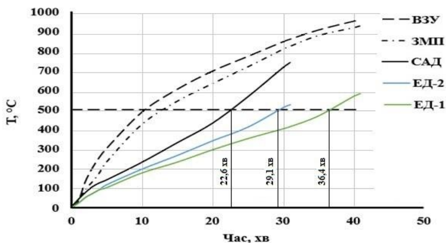
Рис. 1. Залежність зміни температури всередині дослідної установки (ВЗУ), на зовнішній стороні металеві пластина (ЗМП), а також на зовнішній стороні металеві пластина, захищеної вогнезахисними покриттями: САД, ЕД-1 та ЕД-2.
