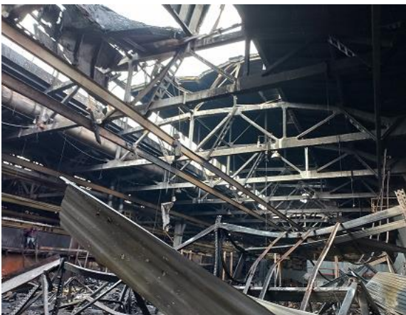
Рис. 1. Багатопролітна одноповерхова будівля, обрушення конструкції світлового ліхтаря.
