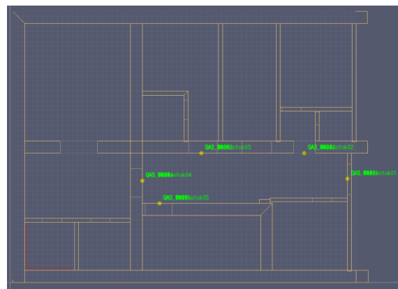
Рис. 1. План поверху та місце розташування датчиків, що вимірюють НЧП.
