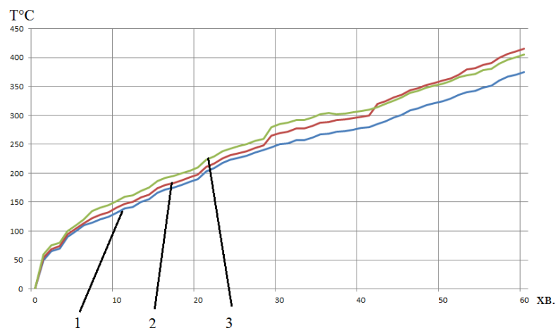
Рис. 3. Графік зміни температури в приарматурному шарі залізобетонної плити: 1, 2, 3 – показники температури в різних частинах залізобетонної плити
