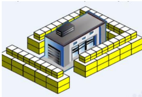
Для захисту 6 компресорних та 3 насосних передбачено використання 174 кліток» Mil7 та 348 « кліток» Mil1. Це складає 14 комплектів «кліток» Mil7 та 39 комплектів « кліток» Mil1. Тривалість улаштування захисту складає не менше 3-х днів (за наявності не менше 15 працівників, 3 навантажувача, 1 вантажівка).
