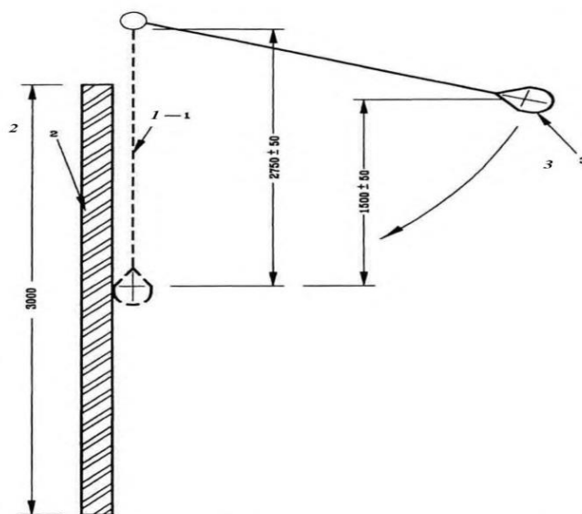
Рис. 2. Випробувальний стенд для випробування на удар
