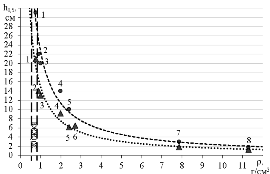
Рис. 1. Глибина половинного проникнення за густиною матеріалу та енергією \gamma -квантів: \blacktriangle \cdots – 1 MeB, \bullet \cdots – 5 MeB; 1 – деревина, 2 – поліетилен, 3 – вода, 4 – ґрунт, 5 – бетон, 6 – алюміній, 7 – сталь, 8 – свинець
