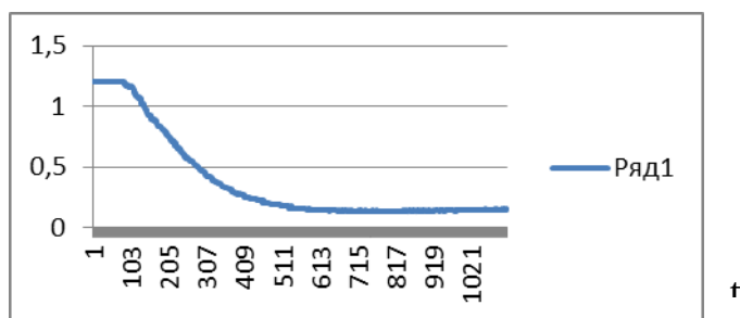
Рис. 4. Графік залежності падіння напруги на фотоеlementі від часу за рахунок задимленості камери
