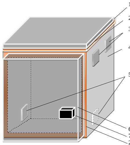
Рис. 1. Схема встановлення зразка для випробувань:
