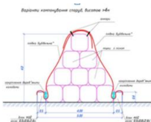
Для захисту одного трансформатора передбачається зведення валу із мішків заповнених піском середньою висотою 1,5 метра у кількості 500 мішків.
