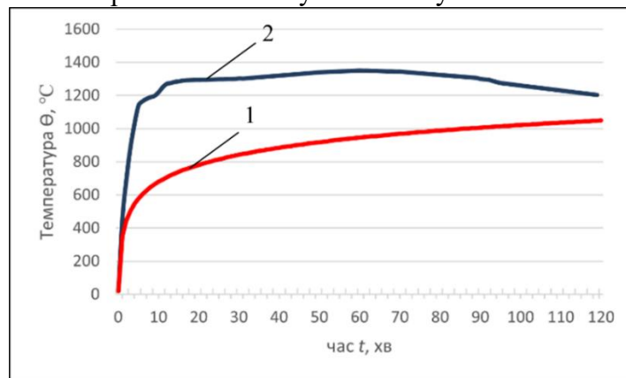
Рис. 2 – Температурні режими пожежі: 1 – стандартний температурний режим пожежі; 2 – температурна пожежна крива RWS.
