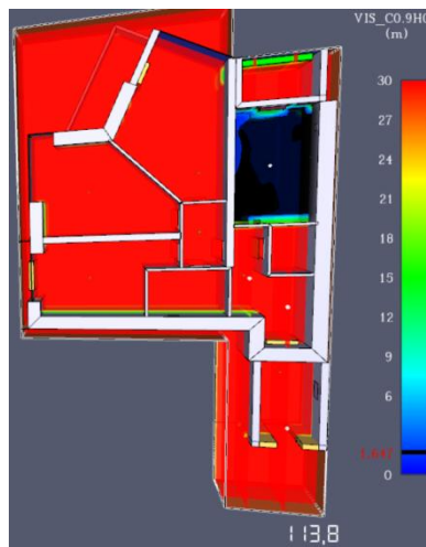
Рисунок 2 – Видимість на висоті 1,7 м під час пожежі
