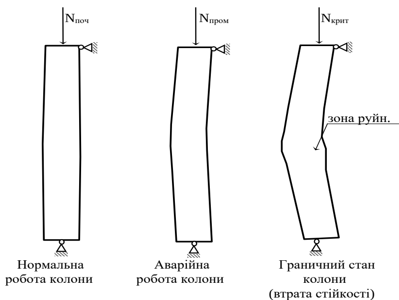
Рисунок 3 – Визначення несучої здатності колони протягом часу оцінювання вогнестійкості.
