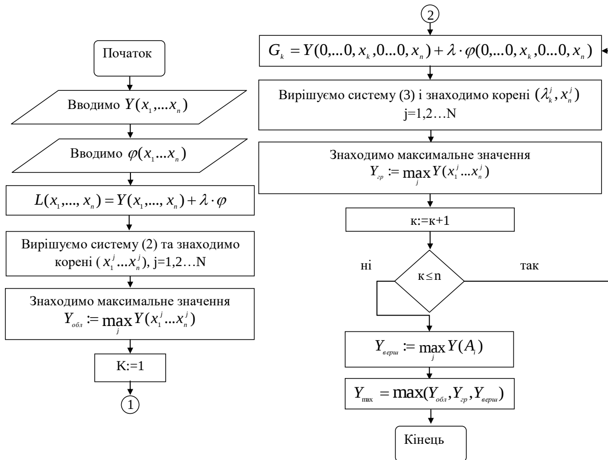
Рис. 3. Структурна схема алгоритму пошуку максимального значення функції відклику
