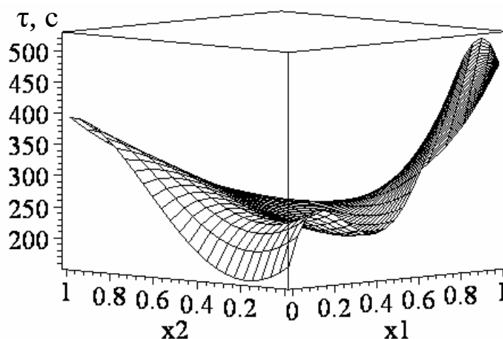
Рис. 2. Поверхня відклику часу теплоізолюючої дії ( \tau ) гелеутворюючого складу \text{Na}_2\text{O} \cdot 2,95\text{SiO}_2\text{-CaCl}_2 в залежності від масового вмісту \text{CaCl}_2 ( x_1 ) та \text{Na}_2\text{O} \cdot 2,95\text{SiO}_2 ( x_2 )
