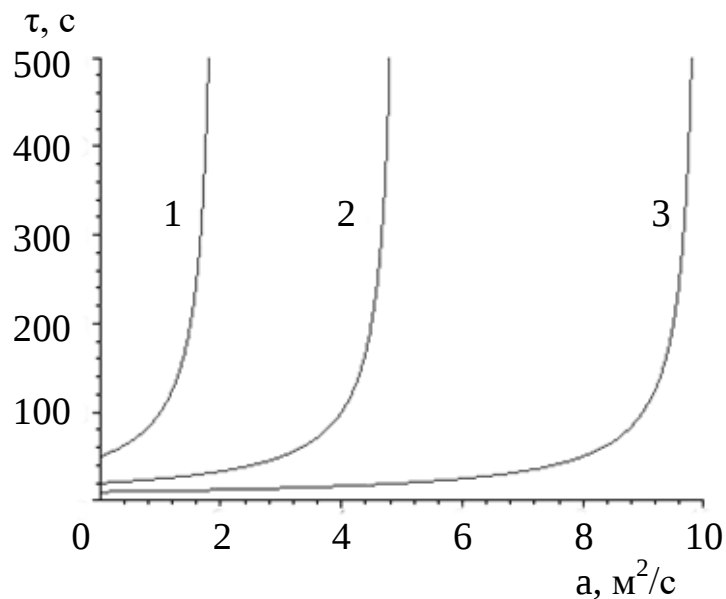
Рис. 6. Залежність часу гасіння ( \tau ) від швидкості розповсюдження пожежі ( a ): 1 – гасіння компактним струменем; 2 – гасіння тонкорозпиленним струменем; 3 – гасіння гелеутворюючим складом
