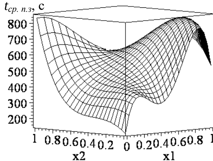
Рис. 7. Поверхня відклику середньозваженого часу повторного займання ( t_{cp. п.з} ) квартири з середньостатистичним горючим завантаженням при його обробці ГУС \text{Na}_2\text{O} \cdot 2,95\text{SiO}_2 - \text{CaCl}_2 в залежності від масового вмісту \text{CaCl}_2 ( x_1 ) та \text{Na}_2\text{O} \cdot 2,95\text{SiO}_2 ( x_2 )
