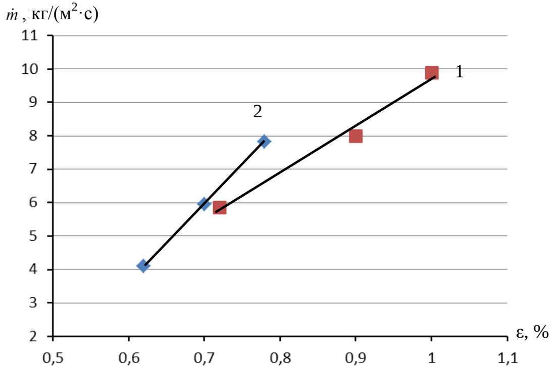
Рисунок 3.10. Залежність «ефективної» масової швидкості горіння від ступеня вигорання (коксового залишку) для склопластиків на основі: 1 – бромвмісної епоксидної системи; 1 – епоксидованого дінафтолу
