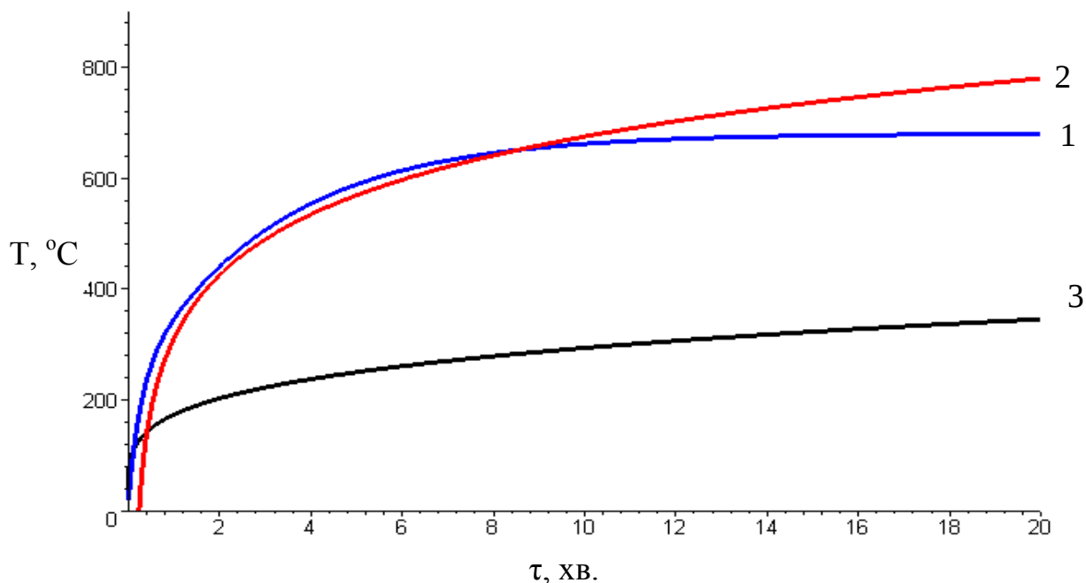
Рисунок 4.1. Температурні режими пожежу: 1 – стандартний режим; 2 – режим відкритої пожежі; 3 – режим пожежі, що повільно розвивається
