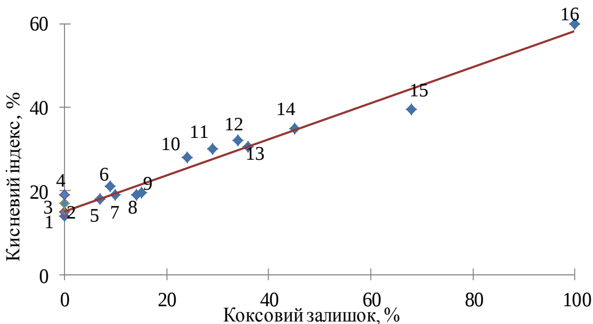
Рисунок 1.6. Залежність кисневого індексу полімерів від виходу коксового залишку при піролізі: 1 – поліформальдегід; 2 – поліетилен, поліпропілен; 3 – полістирол, поліізопрен; 4 – поліамід; 5 – целюлоза; 6 – полівініловий спирт; 7 – поліетилентерефталат; 8 – поліакрилонітрил; 9 – епоксидна смола (ЕД-20); 10 – поліфеніленоксид вогнезахисний; 11 – полікарбонат; 12 – номекс вогнезахисний; 13 – полісульфон; 14 – кінол (фенолформальдегідний полімер); 15 – поліімід; 16 – вуглець
