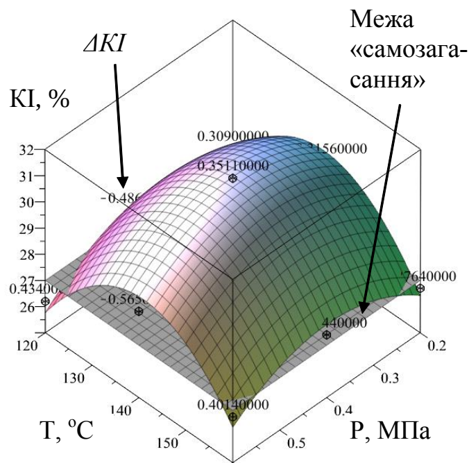
Рисунок 3.8. Залежність кисневого індексу склопластику від умов формування: P – тиск формування композиційного матеріалу,
