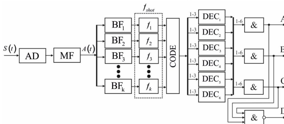
Рис. 1. Функціональна схема ідентифікації вогнепальної зброї за спектральними властивостями прийнятого акустичного сигналу: S(t) – вхідний акустичний сигнал, амплітуда якого змінюється у часі t ; AD – акустичний датчик; MF – медіанний фільтр; BF_k – смугові фільтри, де k – кількість смугових фільтрів; f_{shot} – блок характеристикних частот пострілів; DEC – декодер; & – логічний елемент «Кон'юнкція»
