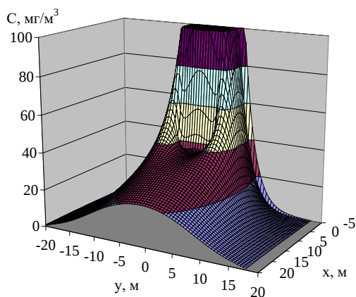
Рис. 2. Просторовий розподіл концентрації хлору при осадженні дрібнодисперсним потоком води
