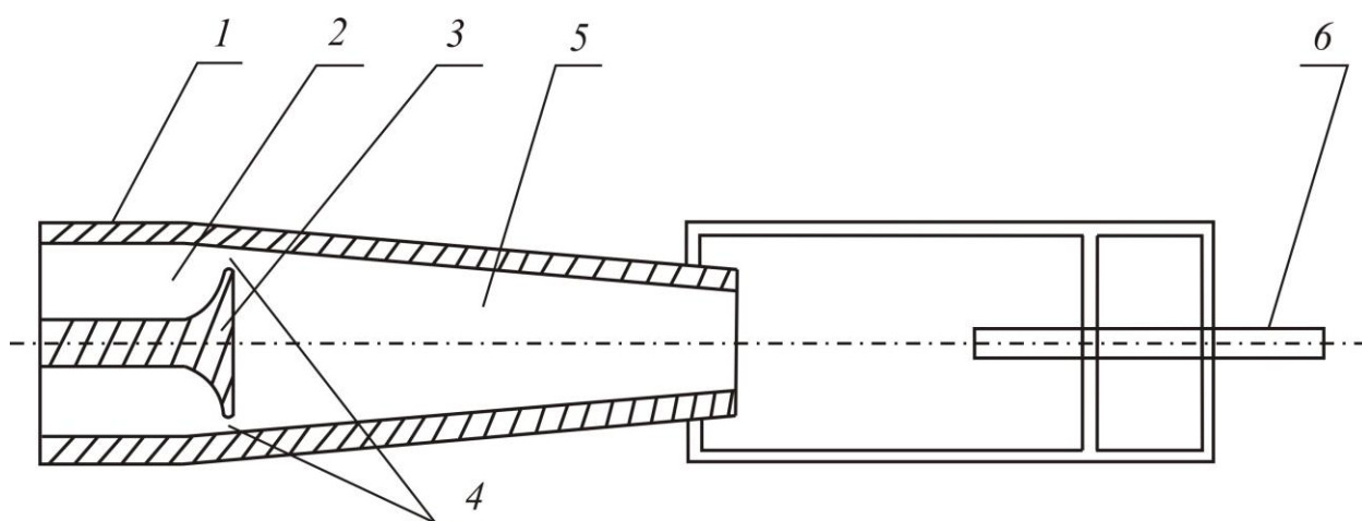
Рис. 1. Ствол з використанням кавітаційних ефектів для розпорощення струменя.
