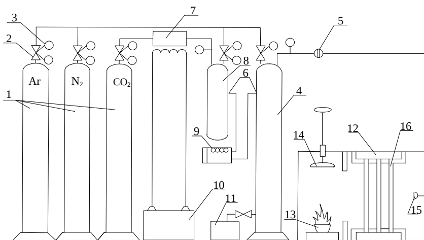
Рис. 1. Принципова схема лабораторного випробувального стенду: 1 – балон з газом; 2 – вентиль; 3 – манометр; 4 – змішувач; 5 – пробковий вентиль; 6 – термopар; 7 – випаровувач; 8 – накопичувач; 9 – регулювальний прилад; 10 – трансформатор; 11 – блок продувки; 12 – випробувальна камера; 13 – модельне вогнище; 14 – пристрій гасіння; 15 – завихрювач; 16 – зразки.
