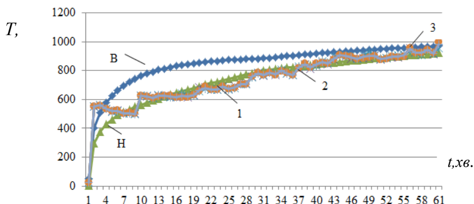
Рис. 1. Дані прогрівання поверхні гофрованого профілю: 1 – середня температура у верхній частині; 2 – середня температура у середній частині; 3 – середня температура у нижній частині; B, H – верхня та нижня межі стандартного температурного режиму.
