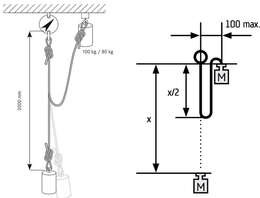
Рис. 2. Випробування динамічної міцності з підрахунком кількості витриманих ривків із фактором 1 за стандартом EN 1891-1998.
