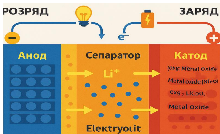
Рис. 2. Схема розряду та заряду літій-іонного акумулятора.
