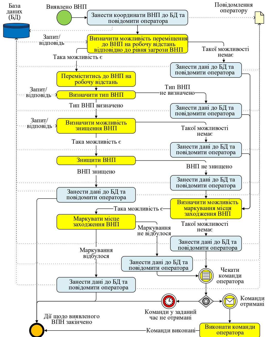
Рис. 1. Символічна модель представлення процедурального знання в ІСУ.
