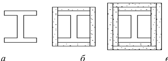
Рис. 1. Переріз зразків колон: а – без вогнезахисного облицювання; б – шар гіпсокартонної плити у 12,5 мм; в – шар гіпсокартонної плити у 25 мм.
