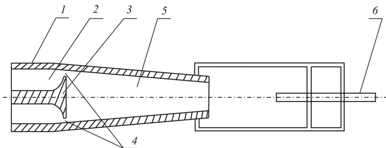
Рис. 1. Ствол з використанням кавітаційних ефектів для розпорошення струменя.
