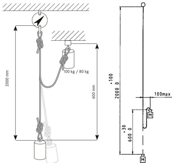
Рис. 1. Визначення максимальної сили ривка за стандартом EN 1891 - 1998.
