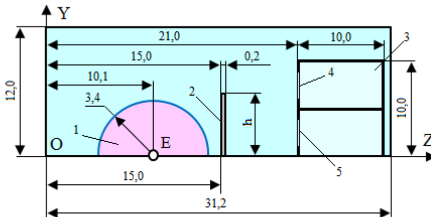
Рис. 1. Схема об'єктів: 1 – хмара водню; 2 – захисна стіна; 3 – будинок; 4 і 5 – вікна другого і першого поверху.
