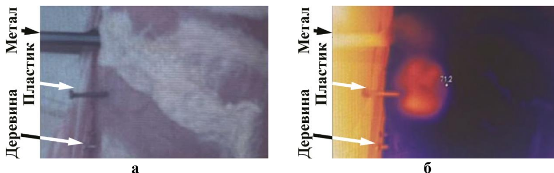
Рис. 2. Результати обробки отриманих під час вимірювань з використанням методів кореляційної НВЧ гіпертермії та проекційної динамічної теплової томографії даних: а – у видимому діапазоні; б – в ІЧ-діапазоні.
