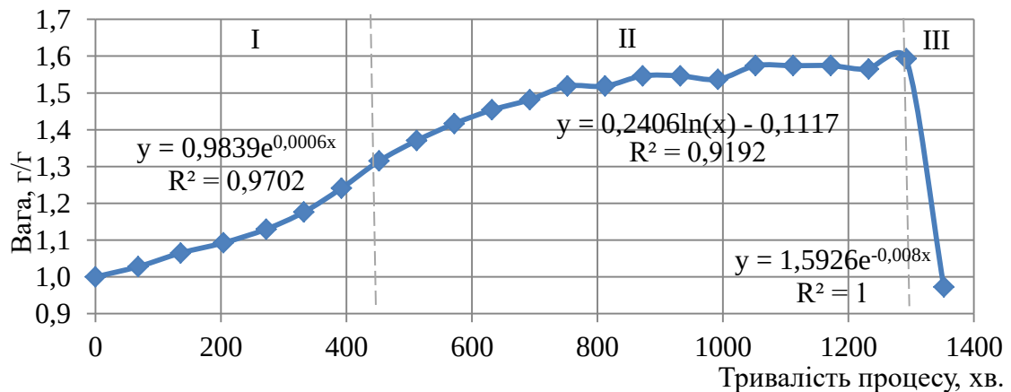
Рис. 1. Динаміка зміни ваги зразків в процесі гідратації-дегідратації: I – ділянка швидкого зростання ступеня насичення; II – ділянка уповільненого насичення; III – ділянка дегідратації деревини.
