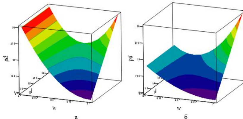
Рис. 1. Поверхні відгуку дисперсійної складової ВПЕ полімерних композитів \gamma_s^d від \omega та \gamma_f^d наповнювачів для полімерів з а – \gamma_p^d=50 мДж/м 2 ; б – \gamma_p^d=20 мДж/м 2 .
