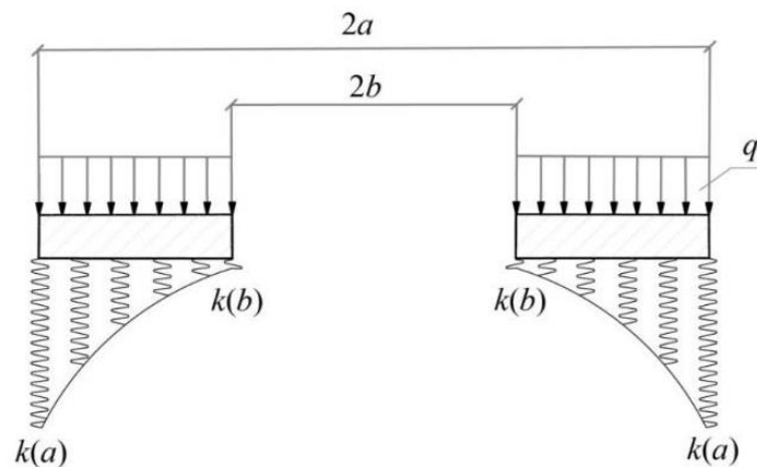
Рис. 1. Кільцева пластина на степенево-змінній пружній основі.
