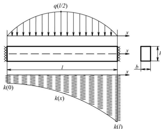
Рис. 1. Балка на змінній пружній основі.
