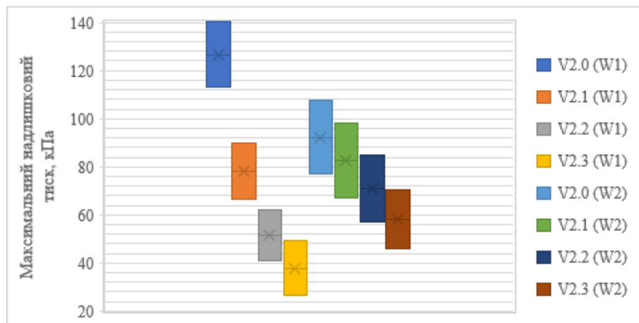
Рис. 3. Діапазони максимального надлишкового тиску на вікнах W1 і W2.
