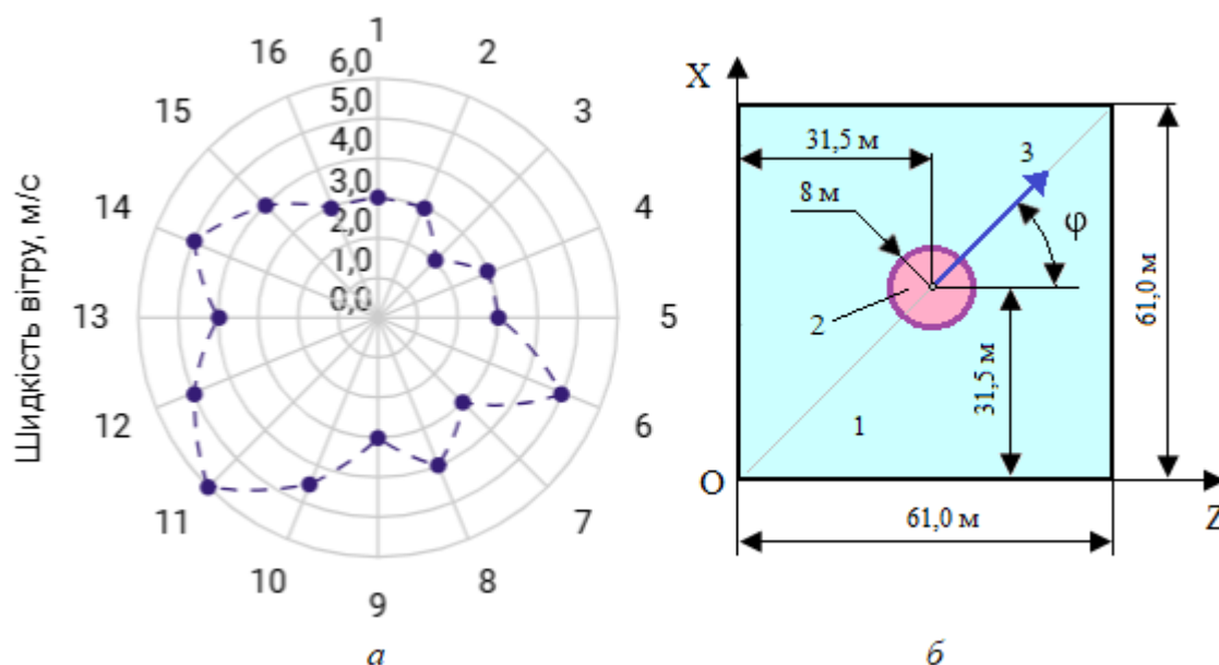
Рис. 1. Розрахункова схема: а) троянда вітрів у епіцентрі можливої аварії; б) мапа об'єктів (1 – промисловий майданчик; 2 – пляма пролиття рідини; 3 – вектор швидкості вітру).
