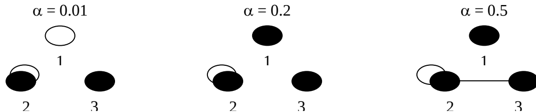
Рис. 1. Зміна зв'язку між факторами при різному рівні значущості для моделі, що характеризує час оперативного розгортання особового складу пожежно-рятувального автомобіля з установкою на пожежний гідрант.
