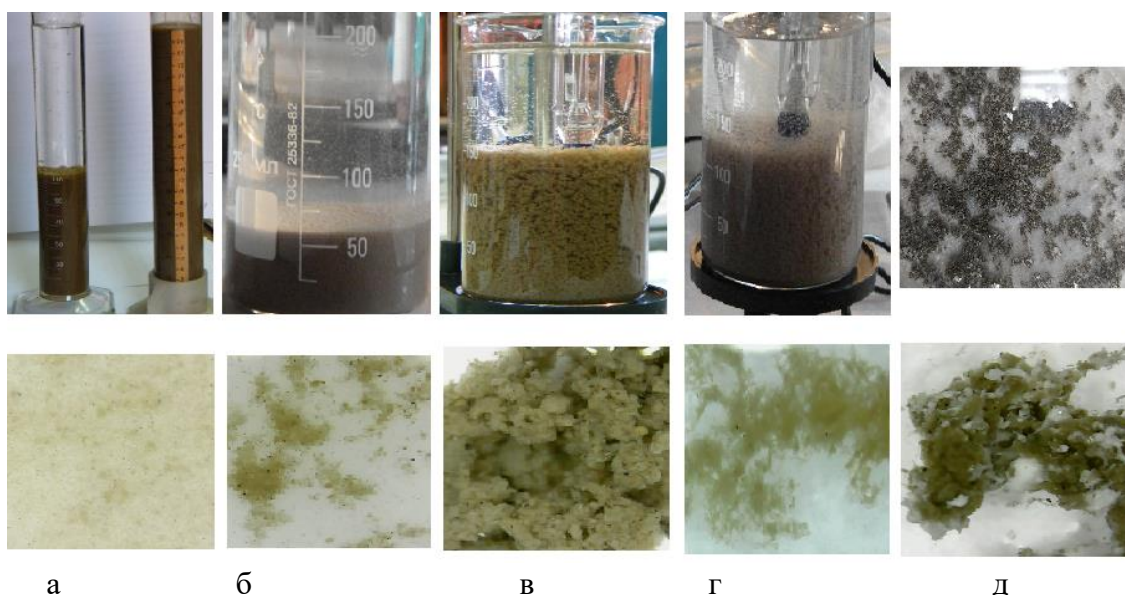
Рис. 2. Результати дослідження зразку глини та мікрофотографії агрегатів (знизу): а – кінетика осадження; б – коагуляція; в – коагуляція з флокуляцією, г – руйнування флокул механічним впливом; д – введення мінеральних часток та мікропіску.
