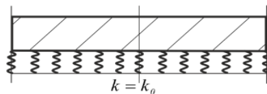
Рис. 3. Закон зміни коефіцієнту постелі для бетонної плити.
