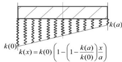
Рис. 2. Закон зміни коефіцієнту постелі для сталевій плити.
