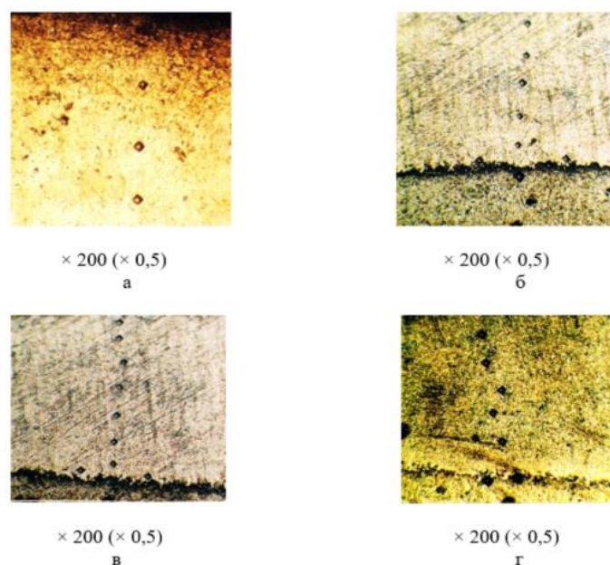
Рис. 1. Вплив ДФДЗ на структуру вуглецевих сталей з різним вмістом вуглецю після попереднього гартування. Режим ДФДЗ: S = 30 мм/с; t = 0,7 мм: а – сталь 20; б – сталь 45; в – сталь У7; г – сталь У12.
