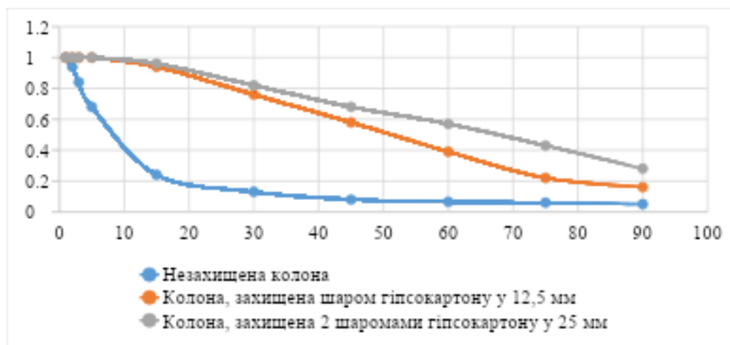
Рис. 2. Зниження коефіцієнта несучої здатності сталевих колон з вогнезахисним облицюванням.
