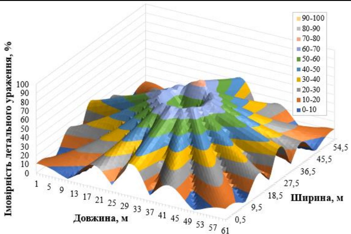
Рис. 2. Сумарне поле ймовірності летальних наслідків людини в зоні аварії.
