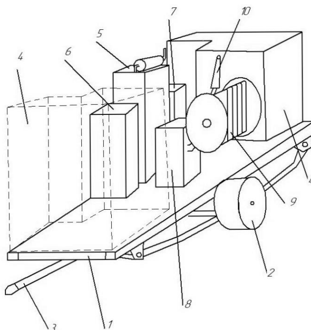
Рис. 1. Мобільна установка для гасіння пожеж тонкорозпиленою водою.
