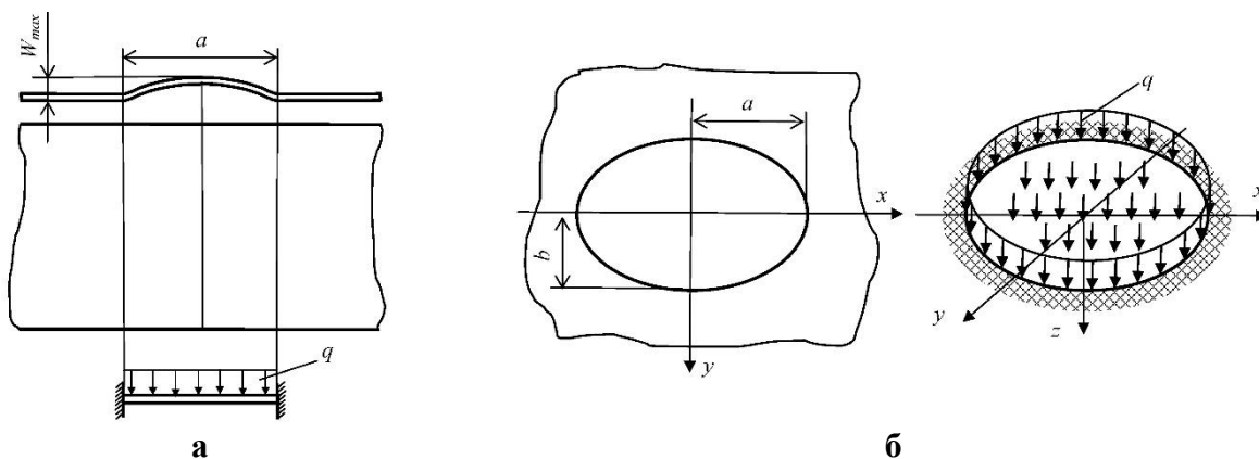
Рис. 1. Розглянуті типи дефектів несучих обшивок та їх рохрахункові схеми: а – безперервна хвилястість; б – вм'ятини (випуклості).
