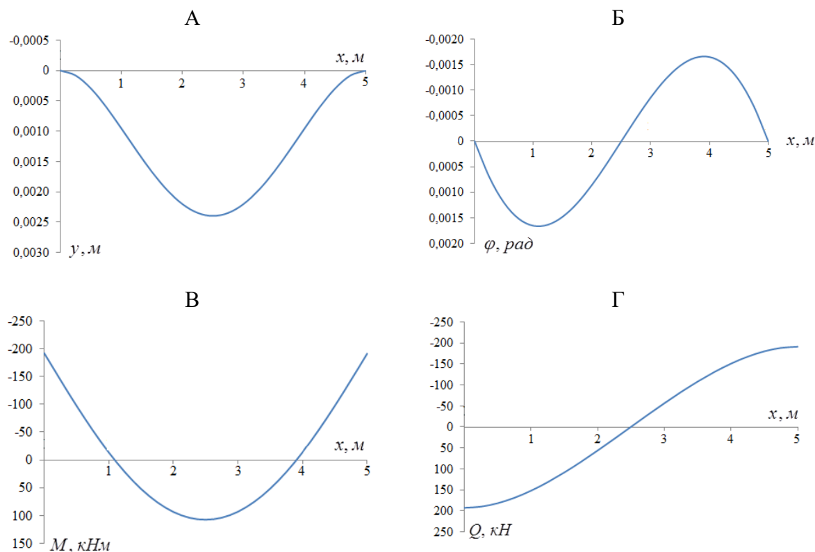
Рис. 2. Графіки параметрів стану балки.
