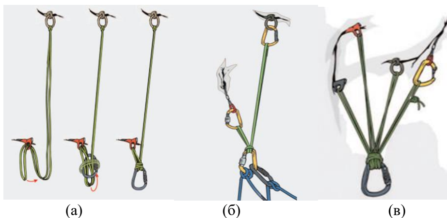
Рис. 1. Різні варіанти побудови південно-тірольської станції: а) петля, протягнута через дві фіксовані точки, з шістьма нитками в анкерному вузлі на центральній точці; б) анкерний вузол із лише чотирма нитками у центральній точці є достатньо
