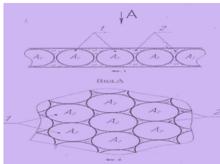
Рис. 3. Схема захисту Li-іон акумулятора: 1– кульки з Ar-аргоном; 2 – пори сепаратора.
