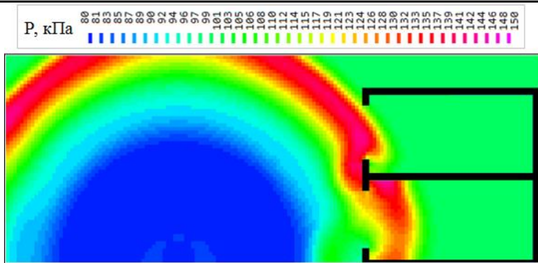
Рис. 2. Поширення вибухової хвилі у випадку руйнування скла вікон.
