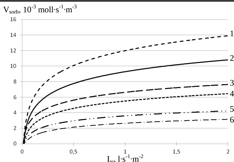
Рис. 1. Залежність інтенсивності осадження V_{\text{sorb}} небезпечних газів від інтенсивності I_w подачі дрібнодисперсного потоку води ( 1 – аміак, 2 – соляна кислота, 3 – фосген, 4 – синильна кислота, 5 – диоксид сірки, 6 – хлор).
