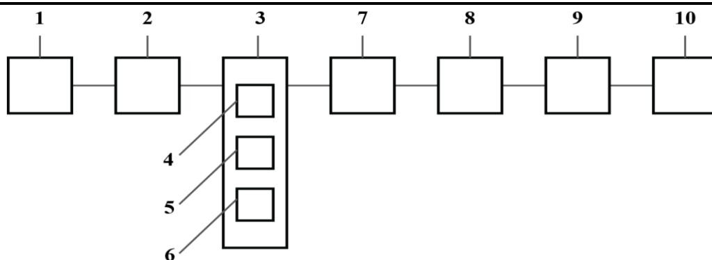
Рис. 1. Структурна схема пристрою для візуалізації сторонніх предметів у м'яких тканинах за допомогою методів мікрохвильової гіпертермії: 1 – НВЧ-генератор; 2 – гнучкий аплікатор; 3 – м'які тканини; 4 – сторонні металеві предмети; 5 – сторонні пластикові предмети; 6 – сторонні дерев'яні предмети; 7 – ІЧ-випромінювач; 8 – ІЧ-оптична система; 9 – матриця ІЧ-приймачів; 10 – програмне забезпечення.
