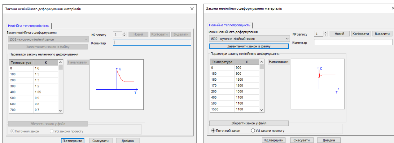
Рисунок 4.7 – Призначення властивостей бетону за підвищених температур:
