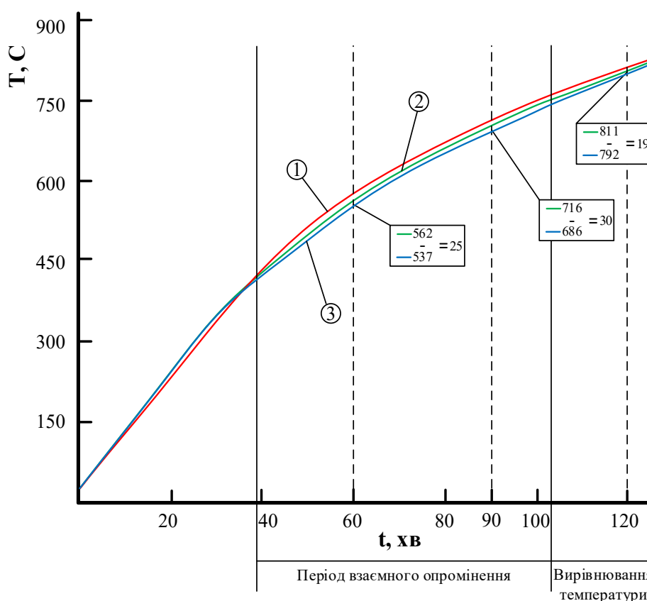
Рисунок 4.22 – Графіки різниці значень температури шару бетону на глибині 30 мм на різних відрізках часу у відповідних зонах: червона лінія – зона ділянки балки на відстані 200 мм від колони; зелена лінія – зона ділянки колони на
