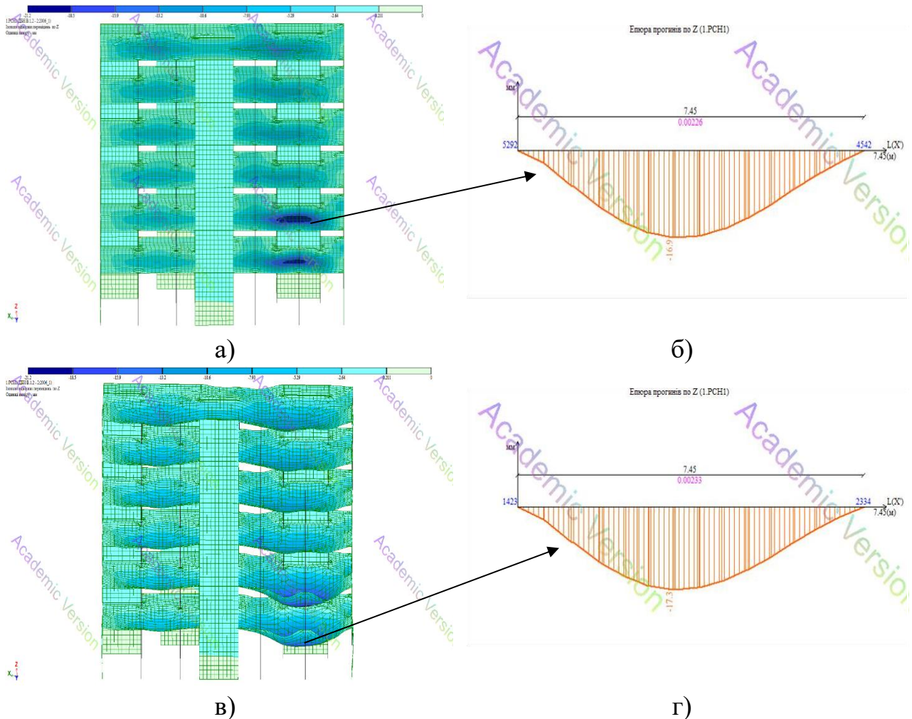
Рисунок 3.8 – Напружено–деформований стан конструкцій та переміщення при пожежі тривалістю 60 хв.: а) – ізополя відносних переміщень по Z; б) – епюра прогинів верхньої плити перекриття (16,9 мм); в) – ізополя переміщень по Z збільшені у 20 разів; г) – епюра прогинів нижньої плити перекриття (17,3 мм)
