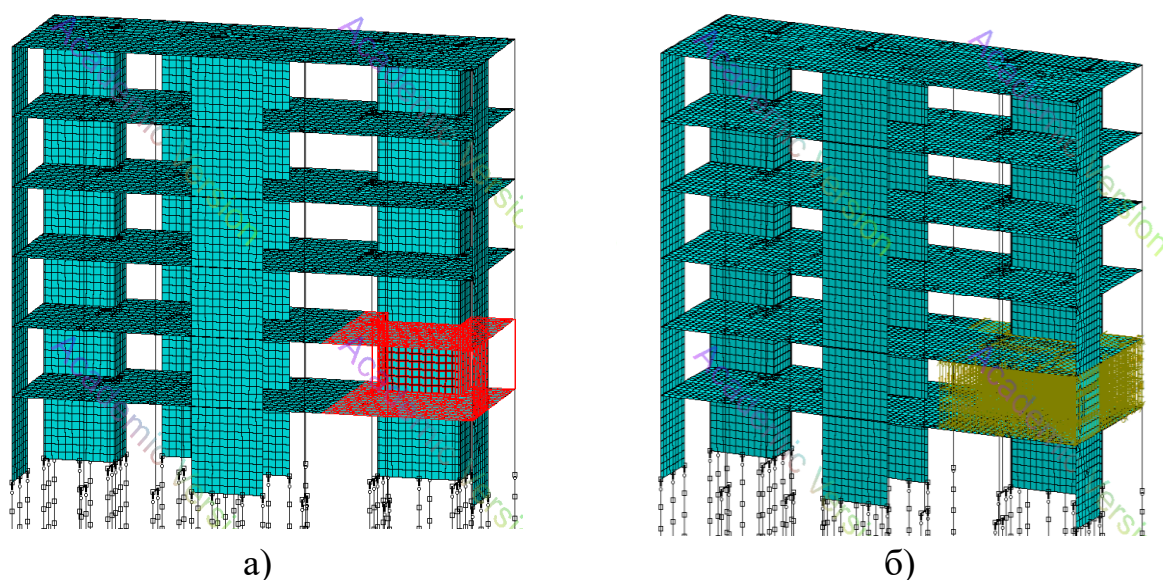
Рисунок 3.5 – Місця дії аварійного навантаження в скінченно–елементній моделі будівлі: а) – ділянка пожежі; б) – зона вибухового навантаження.
