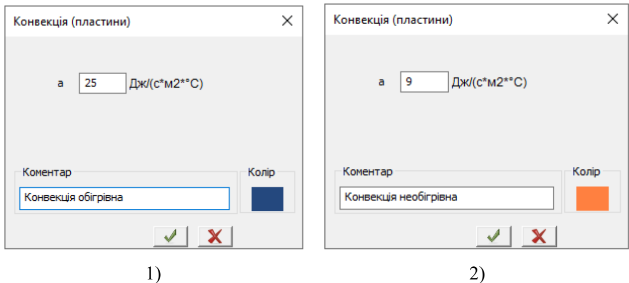
Рисунок 4.8 – Призначення коефіцієнта конвекційного теплообміну: 1) обігрівна частина конструкції; 2) необігрівна частина конструкції
