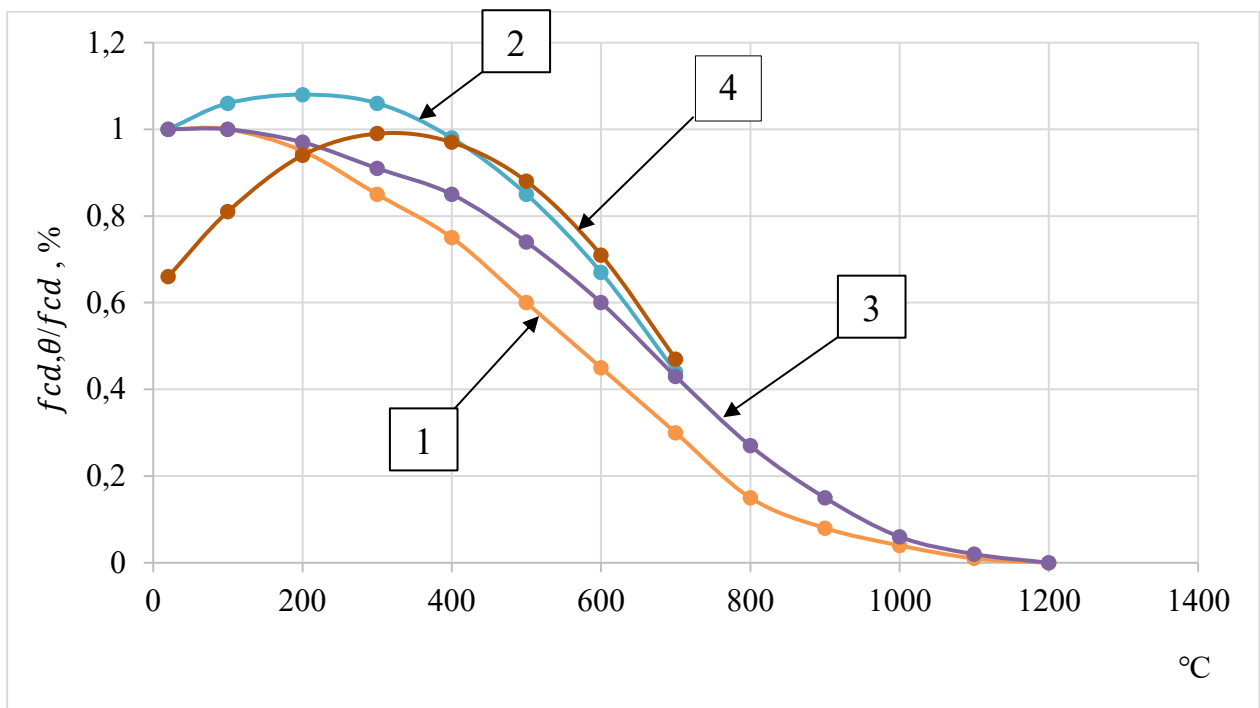
Рисунок 2.3 – Порівняльний графік зменшення міцності бетону при підвищенні температури: 1) керамзитобетон за EN 1992–1–2; 2) керамзитобетон за результатами натурних випробувань; 3) важкий бетон за EN 1992–1–2; 4) важкий бетон за результатами натурних випробувань
