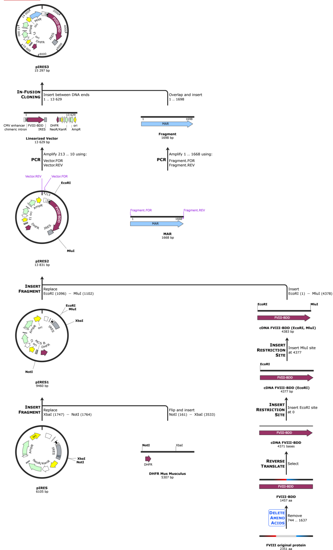
Мал. 1. Схема процесу отримання рекомбінантної плазміді pIRES3
