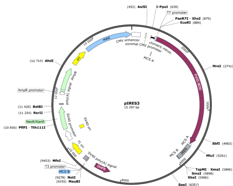
Мал. 2. Генетична карта плазмиди pIRES3
