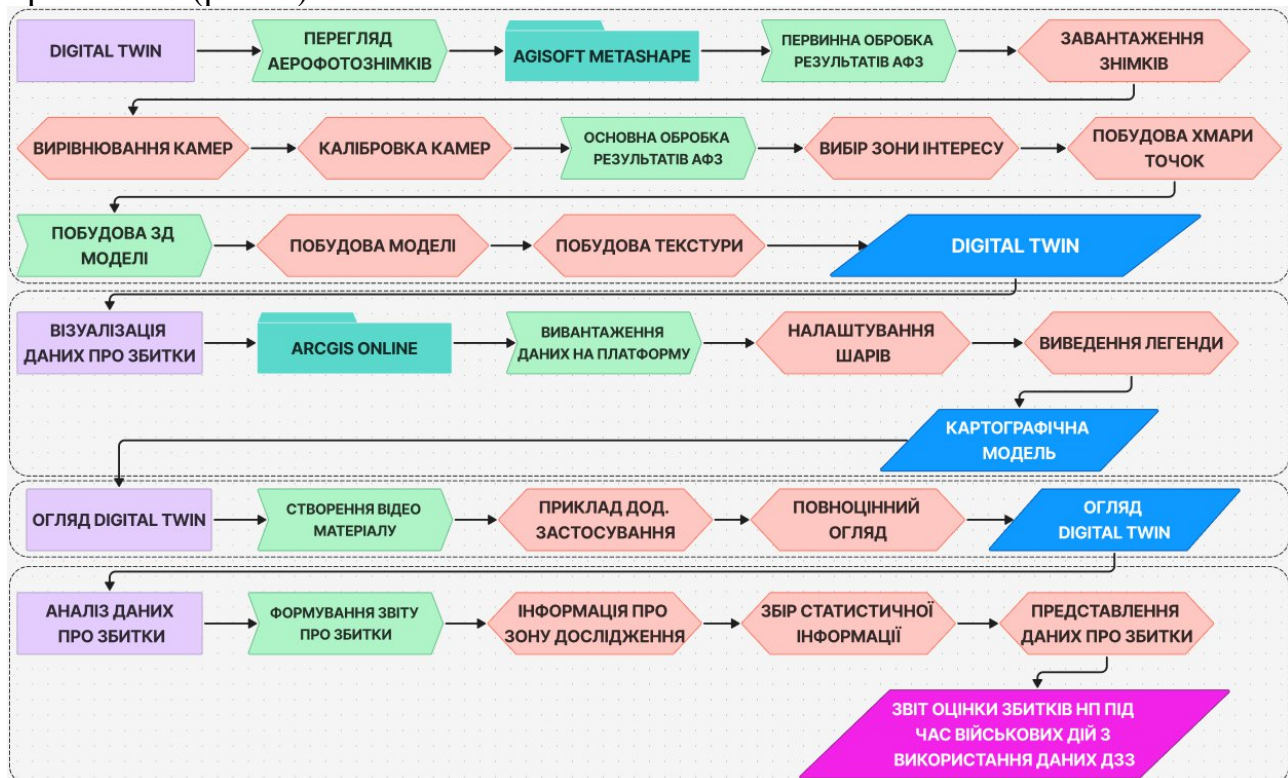
Рисунок 1. Методика побудови цифрових тривимірних двійників населених пунктів для представлення даних про збитки
