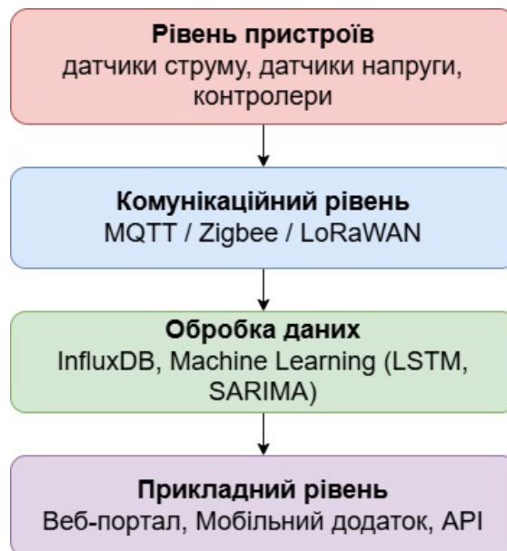
Рисунок 1. Архітектура IoT-системи енергомоніторингу
