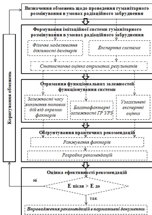
Рисунок 1 – Керуючий алгоритм розв'язання математичної моделі гуманітарного розмінування в умовах радіаційного забруднення
