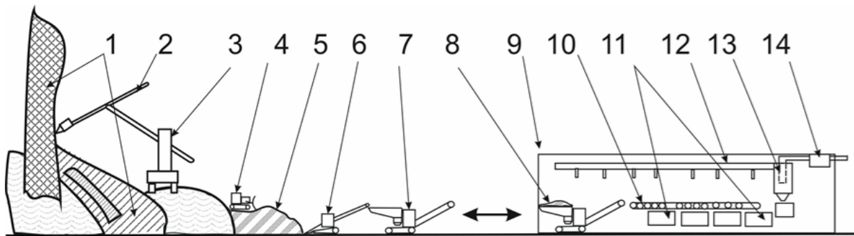
Рисунок 1 – Схема технології мобільної інтенсивної розборки зруйнованих споруд з переробкою уламків задля подальшого використання у будівництві: 1 – початковий стан руїн, 2 – навісне обладнання екскаватора, 3 – екскаватор, 4 – бульдозер, 5 – кагат, 6 – породонавантажувальна машина, 7, 8 – пересувна дробарка, відповідно, під час завантаження кузова та при подрібненні породи, 9 – пункт сепарації, 10 – дисковий сепаратор, 11 – контейнери для відсортованого матеріалу, 12 – жорсткий трубопровід з відростками, 13 – фільтруючий елемент, 14 – вентилятор
