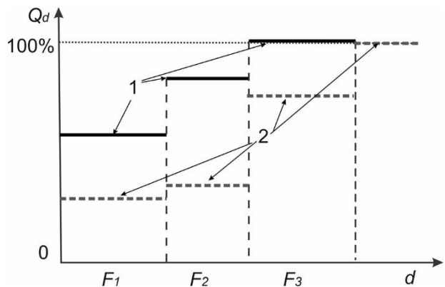
Рисунок 3 – Гранулометрична діаграма подрібненого матеріалу після сепарації:
