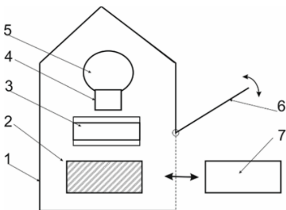
Рисунок 2 – Схема поперечного перерізу пункту сепарації матеріалу: 1 – каркасна тимчасова споруда; 2 – контейнер для збору відсіяного матеріалу; 3 – дисковий сепаратор; 4 – патрубок вентиляційного всмоктувального трубопроводу; 5 – трубопровід; 6 – двері для обміну контейнерів; 7 – порожній контейнер
