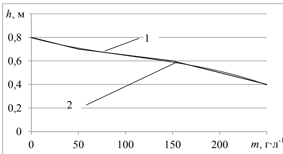
Рис. 1. Зависимость ударпрочности от содержания вермикулита в огнезащитном покрытии: 1 – экспериментальная ломаная; 2 – аппроксимирующая кривая
