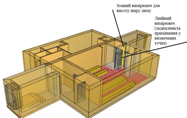
Рис. 1. Розміщення лінійного та зонного вимірювачів
