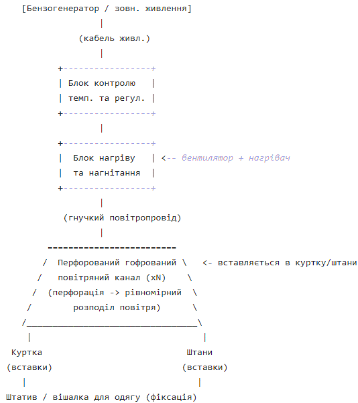
Рисунок 1 – Примітивна схема установки для сушіння захисного одягу пожежника в умовах ліквідації надзвичайної ситуації
