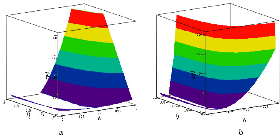
Рисунок 1 – Поверхні відгуку залежностей полярної (кисотно-лужної) складової ВПЕ наповнених полімерних матеріалів ( \gamma^{ab}_s ) від \omega наповнювачів та величини Q для зв'язуючих з \gamma^a_c = 1 мДж/м 2 ; \gamma^b_c = 25 мДж/м 2 і наповнювачів з: а – \gamma^b_n = 50 мДж/м 2 ; б – \gamma^b_n = 1000 мДж/м 2
