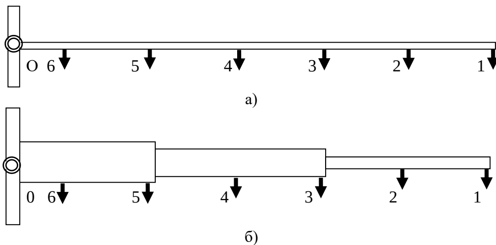
Рисунок 1 – Розрахункова схема рядка розподільчої мережі:
