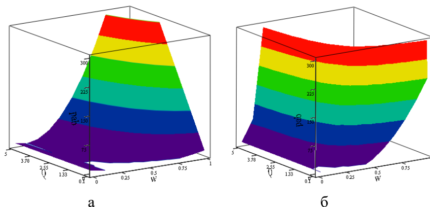
Рисунок 2 – Поверхні відгуку залежностей полярної (кисотно-основної) складової ВПЕ наповнених полімерних матеріалів ( \gamma^{ab}_s ) від \omega наповнювачів та величини Q для зв'язуючих з \gamma^a_c = 7 мДж/м 2 ; \gamma^b_c = 1 мДж/м 2 і наповнювачів з: а – \gamma^b_n = 50 мДж/м 2 ; б – \gamma^b_n = 1000 мДж/м 2
