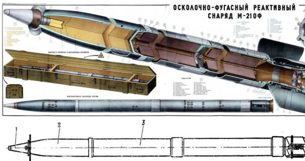
Рисунок 1 – Компонувочна схема 122-мм НКРС М-21ОФ індексу 9М22У = 66,85 кг:
