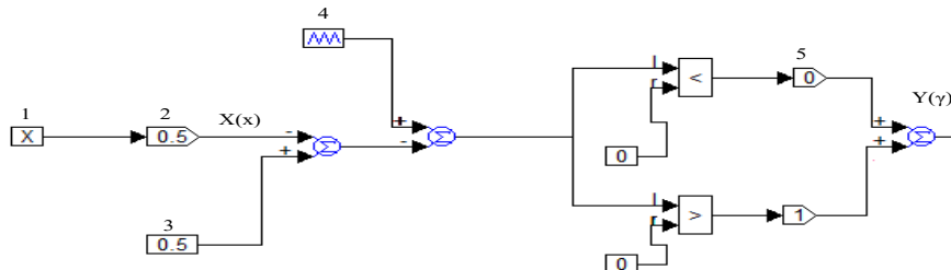
Рисунок 1 – Функціональна модель приладу формування вхідного сигналу:
