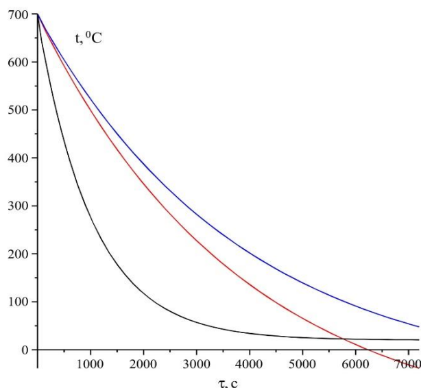
Рисунок 2 – Математичне моделювання швидкості охолодження ЛІАБ: порівняння ЛПЕЖ з використанням вогнегасної речовини з різною початковою температурою: чорна – 20 °С; червона – -80 °С; синя – -190 °С
