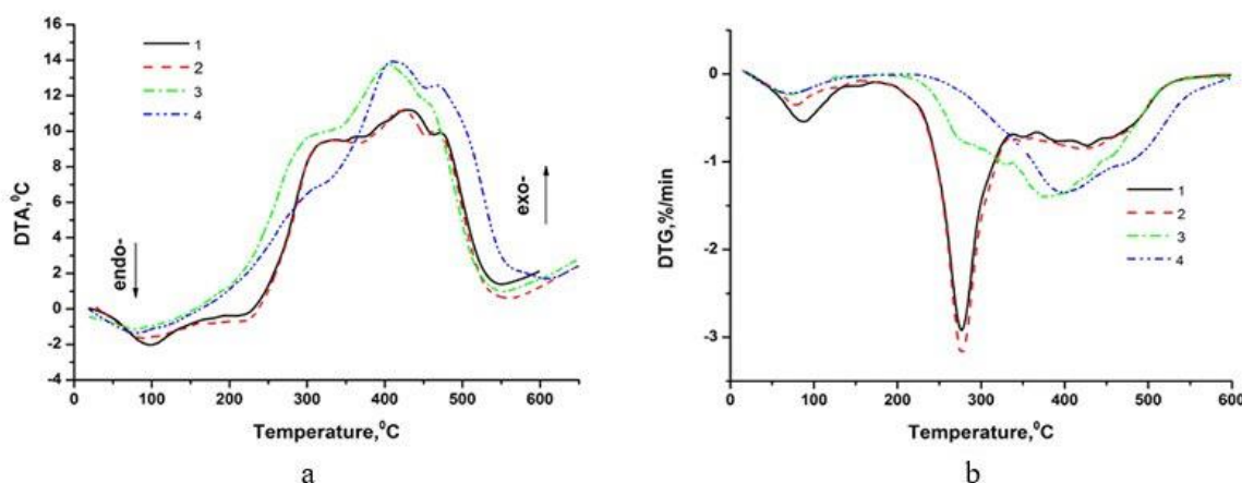
Рисунок 1 – Порівняння кривих DTA досліджених зразків
