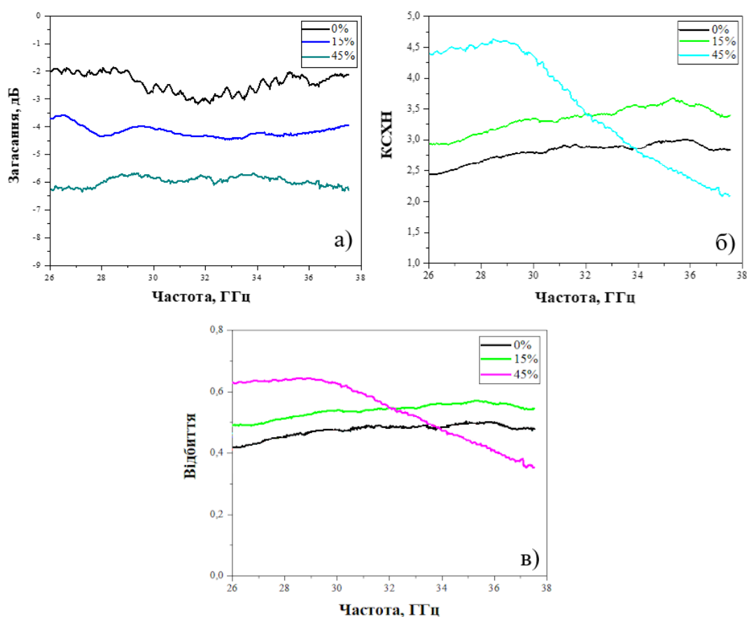
Рисунок 2 – Спектри загасання (а), коефіцієнта стоячої хвилі по напрузі (КСХН) (б) та відбиття (в) досліджуваних зразків з різною концентрацією \text{Fe}_3\text{O}_4
