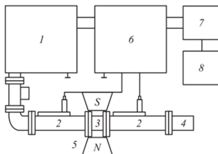
Рисунок 1 – Блок-схема експериментальної установки: 1 – генератор; 2 - напрямлені відгалужувачі падаючої та відбитої хвилі, відповідно; 3 – хвилевод зі зразком; 4 – узгоджене навантаження; 5 – магніт; 6 – індикатор; 7 – АЦП; 8 – комп'ютер
