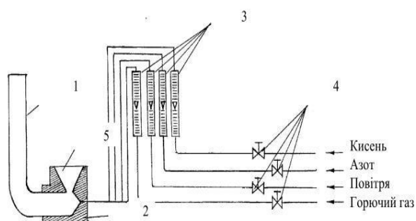
Рисунок – 1. Схема та фото лабораторної установки для визначення вогнегасної ефективності порошків при гасінні полум'я із змінною концентрацією кисню в газоповітряному середовищі: 1 – циліндричний пальник Бунзена; 2 – ежектор; 3 – ротаметри; 4 – регулювальні крани; 5 – лійка ежектора
