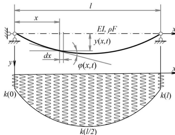
Рисунок 1 – Розрахункова схема вільних коливань балки
