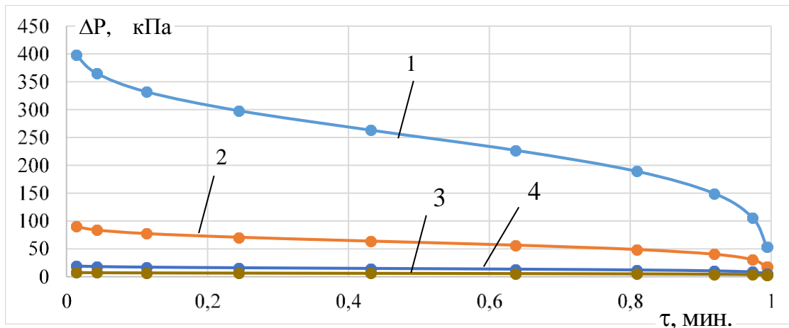
Рис. 3. – Залежність збиткового тиску: 1- r=10 м; 2 – r=20 м; 3 - r=50 м; 4 – r=100 м
