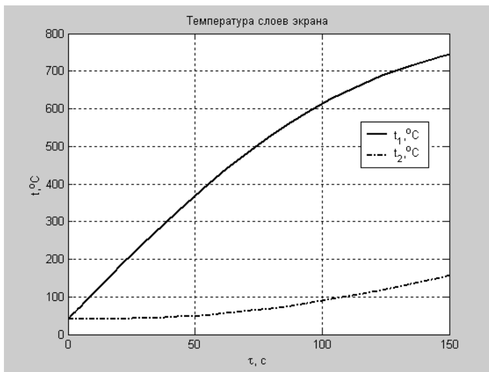
Рис. 2 – Графики зависимости температур ( t_1 и t_2 ) слоев двухслойного экрана от времени теплового воздействия \tau .
