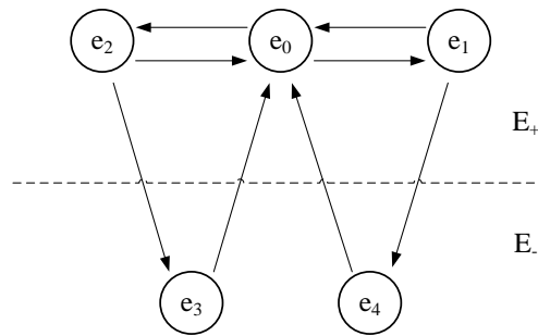
Рисунок 1. Діаграма переходів і станів процесу X(t) функціонування транспортного засобу із періодичним ТО
