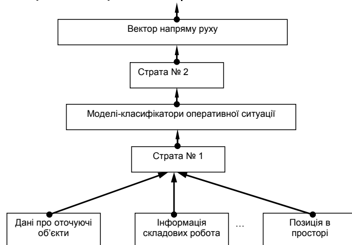
Рис. 2. Структура підсистеми перетворення інформації
