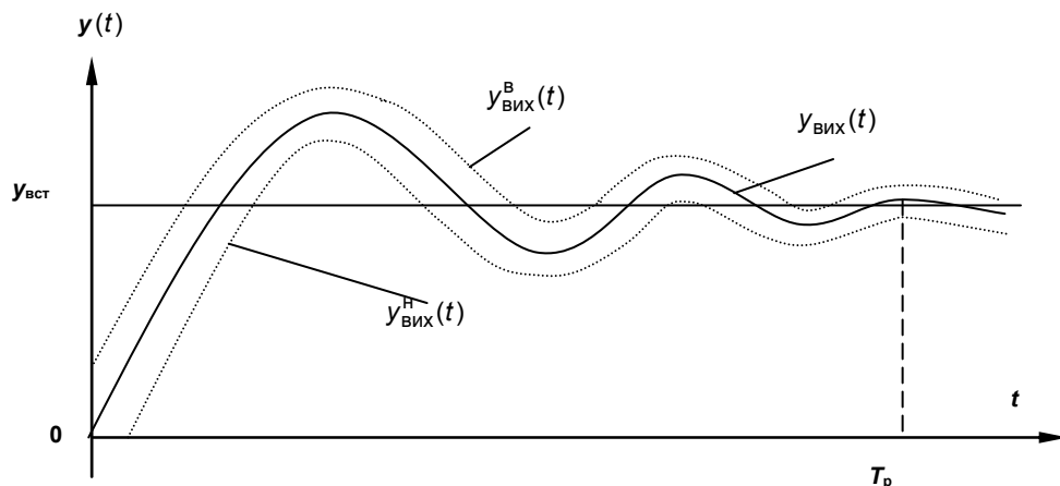
Рис. 1. Граничні криві функції працездатності аналогового пристрою в динамічному режимі
