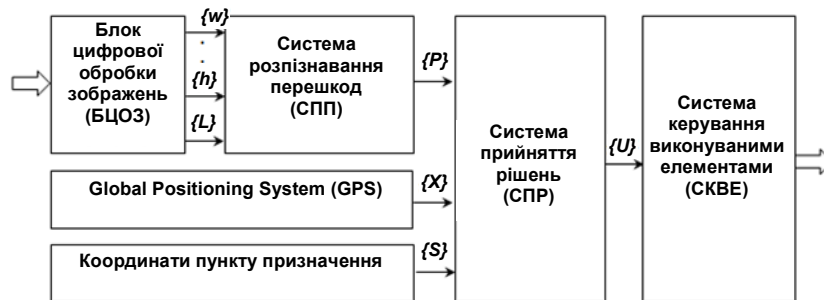
Рис. 1. Структурна схема системи керування АМБ
