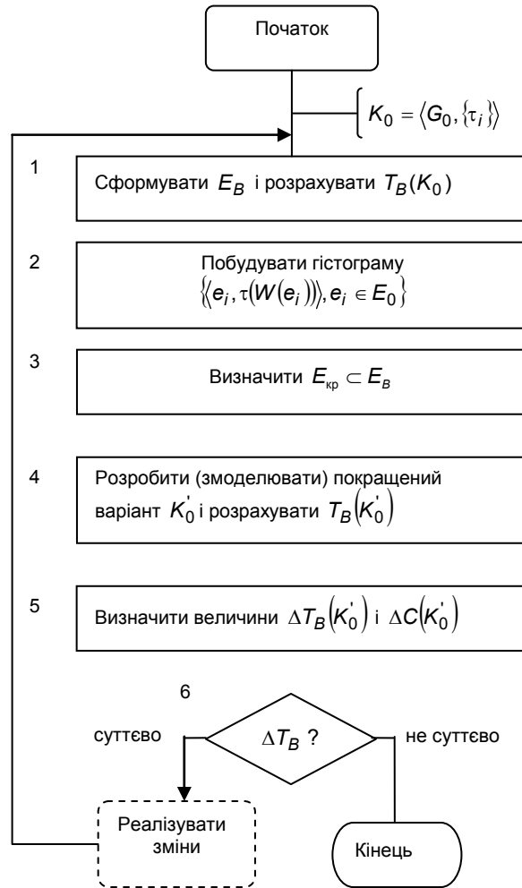
Рис. 2. Алгоритм оптимізації конструкції за критерієм
