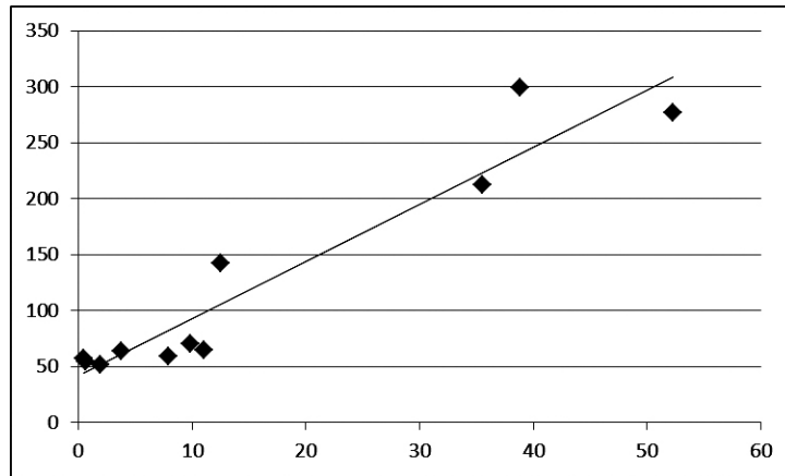
Рис. 1. Лінія тренду
