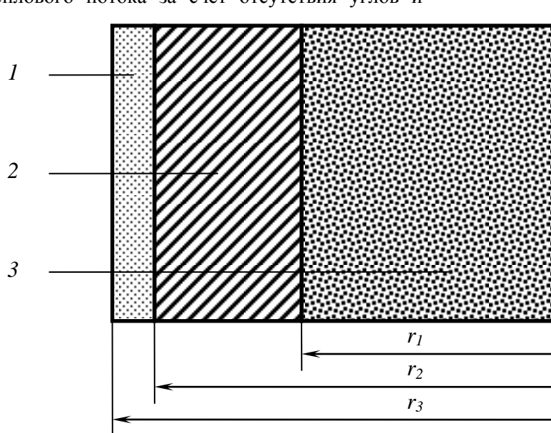
Рис. 1. Схема трехслойной тепловой системы экспериментального образца: 1 - реактивное покрытие, которое испытывается, 2 - стальной цилиндрический образец, 3 - теплоизоляция; r_1 - радиус внешней поверхности теплоизоляции полости образца, м; r_2 - радиус внешней поверхности стального цилиндра, м; r_3 - радиус внешней поверхности защитного покрытия, принятый начальному радиусу защитного покрытия до нагревания, м
