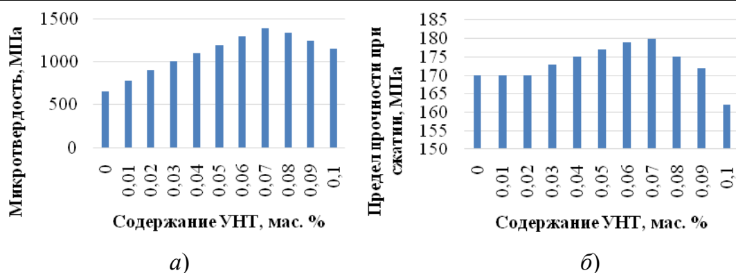
Рис. 1. Зависимость микротвердости (а) и предела прочности при сжатии (б) порошковых нанонаполненных металлополимерных композитов, полученных из порошковых систем медь – УНТ – омедненный ПТФЭ (6 мас. %), от содержания УНТ
