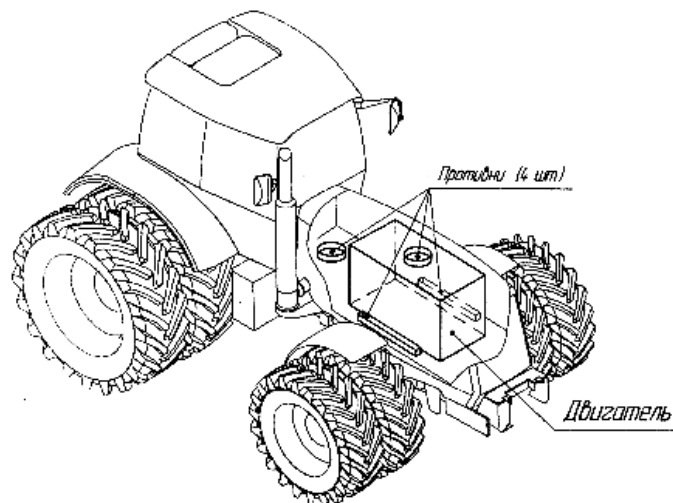
Рис. 1. Схема размещения противней в моторном отсеке трактора «Беларус» серии 3022
