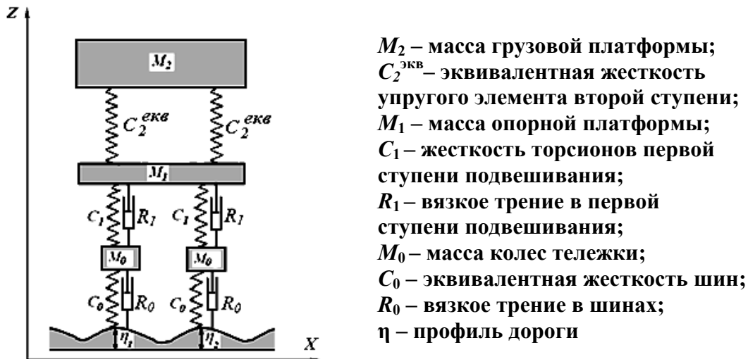
Рис.1. Плоская вертикальная механическая модель тележки
