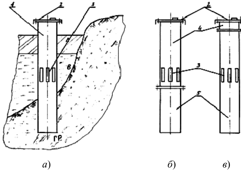
Рис. 1. Модификация зимнего колодца водоема № 2: а – фигура 1; б – фигура 2; в – фигура 3
