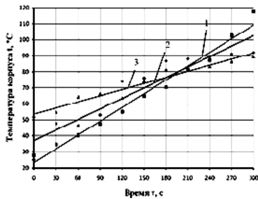
Рис. 1. Графические зависимости температуры корпуса для установки сетчатого материала с шагом плетения 1000 мкм по времени: 1 – корпус без сетчатого материала; 2 – установка сетчатого материала под углом 90°; 3 – установка сетчатого материала под углом 60°
