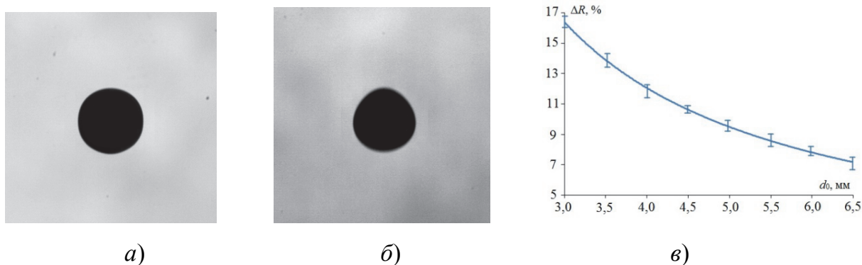
Рис. 1. Видеogramмы с изображениями капли воды ( d_0 \approx 6,5 мм) после прохождения расстояния 1 м в воздушной (а) и высокотемпературной (б) газовой среде; зависимость параметра \Delta R от начального размера d_0 каплей воды при прохождении каплями расстояния около 1 м в высокотемпературных продуктах сгорания модельного очага (в)
