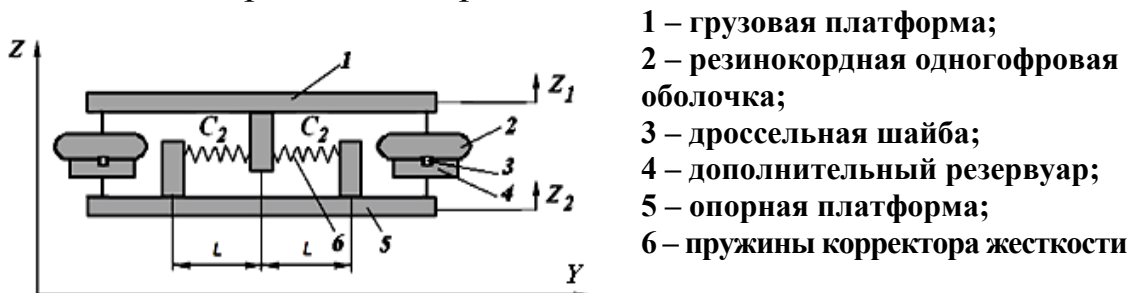
Рис. 1. Схема модифицированного упругого элемента второй ступени подвешивания с корректором жесткости
