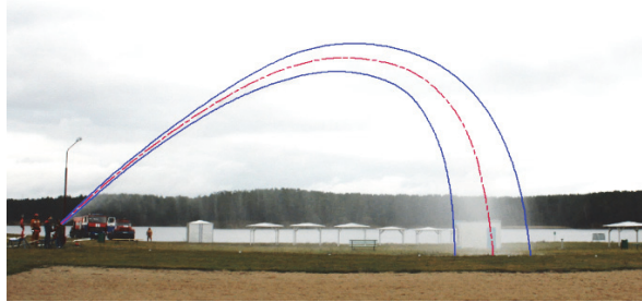
Рис. 1. Кривые, ограничивающие верхнюю и нижнюю части гидравлической осесимметричной струи
