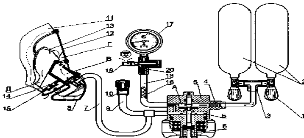
Рис. 1. Принципиальная схема дыхательного аппарата ПТС «Базис»
