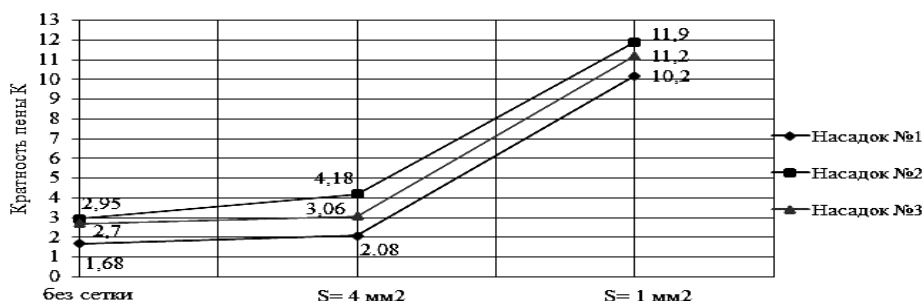
Рис. 1. Зависимость кратности воздушно-механической пены от дополнительного механического сопротивления
