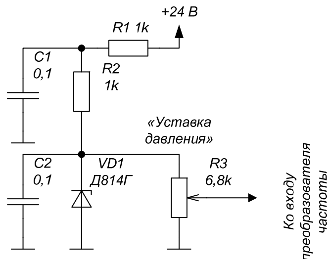
Рис. 1. Схема управления частотой ПЧ на базе потенциометра
