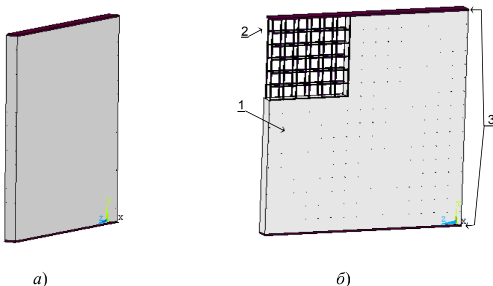
Рис. 1. Схема расчетной области железобетонной несущей стены для проведения расчета предела огнестойкости: а – общий вид, который используют для вычислительного эксперимента; б – схема армирования: 1 – бетон; 2 – рабочий арматурный каркас: d = 16 мм; 3 – траверсы нагрузочной рамы
