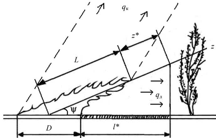
Рис. 1. Схема воздействия тепловых потоков от пламени низового пожара на ЛГМ: L – длина пламени; \psi – угол наклона пламени ветром; D – ширина кромки горения; z^* – предельное расстояние от пламени, на котором происходит воспламенение ЛГМ; l^* – ширина минерализованной полосы; q_k – конвекционный тепловой поток от пламени; q_l – лучистый тепловой поток от пламени
