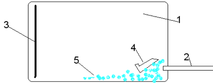
Рис. 1. Схема лабораторной установки: 1 – полимерный резервуар с плоским дном; 2 – впускной патрубок; 3 – выявляющая бумага; 4 – загрузочное устройство; 5 – углеводородная жидкость
