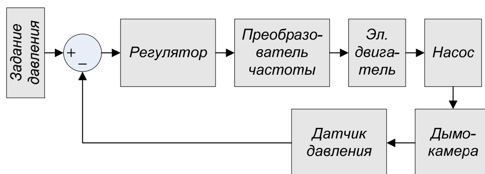
Рис. 1. Система автоматического регулирования давления в дымокамере
