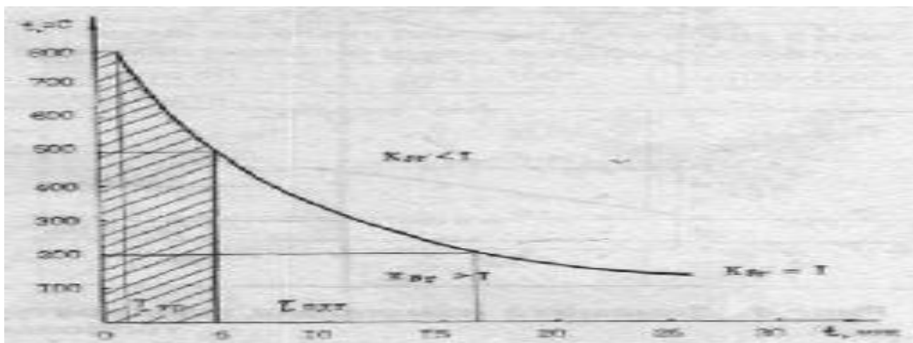
Рисунок 3 - Время прогрева теплозащитного костюма в зависимости от температуры газовой среды при условии естественной конвекции:
