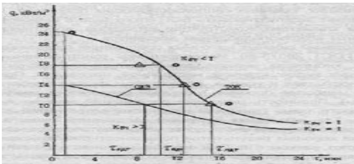
Рисунок 1 - Значения t_{ПДТ} для ТОК и СЛЗ в зависимости от плотности потока теплового излучения:
