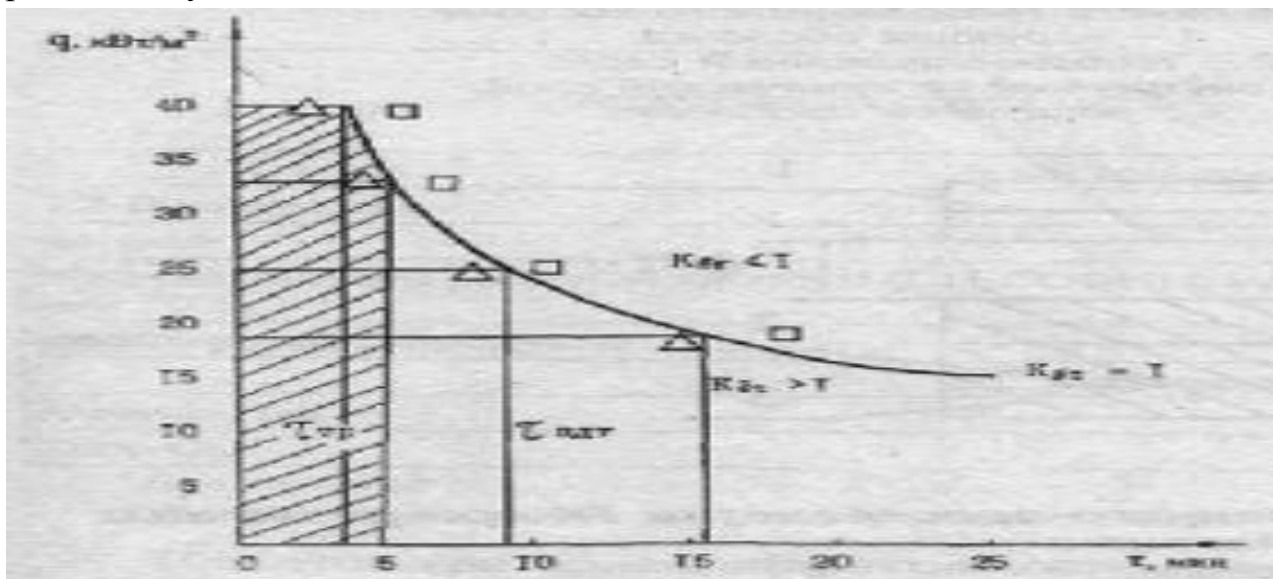
Рисунок 2 - Значения t_{ПДТ} для ТК в зависимости от плотности потока теплового излучения:
