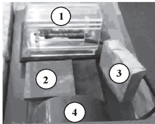
Рис. 5. Лабораторная установка по определению среднего коэффициента качества гамма-излучения: 1 – блок детектирования с детектором СБМ-20; 2 – свинцовый фильтр; 3 – алюминиевый фильтр; 4 – коллиматор с источником гамма-излучения
