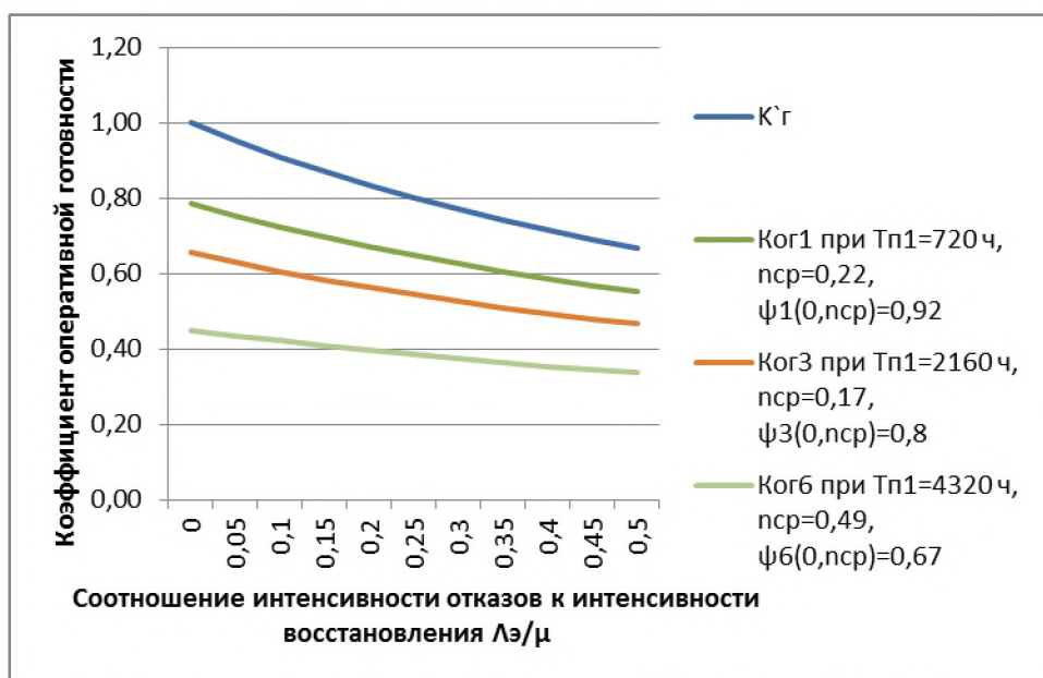
Рис. 1. График коэффициента оперативной готовности K_{ог} в дежурном режиме ( K_{р} = 1 ) в условиях ЧС, при N=100; T_{п} = 720 \text{ ч}, 2160, 4329 \text{ ч}; \lambda_6 = 10^{-6} \text{ ч}^{-1}
