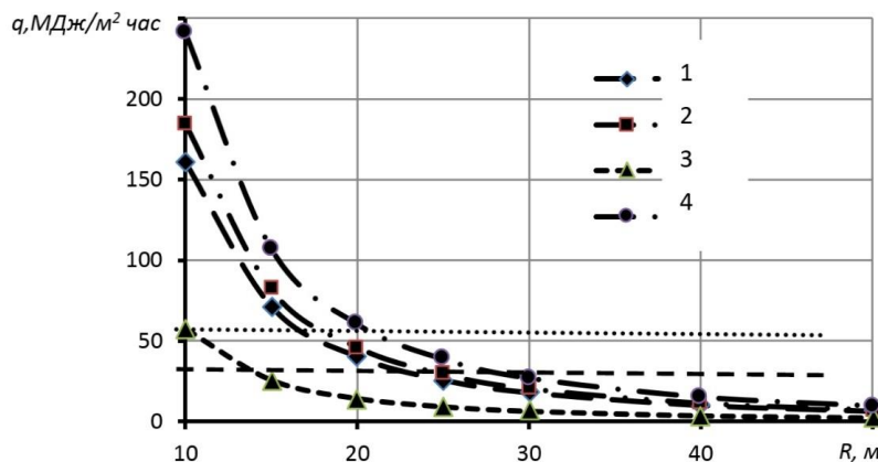
Рисунок 1 Інтенсивність тепловиділення ( q , \text{МДж/м}^2 \cdot \text{год} ) на відстані ( R , \text{м} ) від центру факела палаючих вуглеводнів: 1 бензин; 2 - газ; 3 - метан; 4 - пропан; ліній штрихова і пунктирна, відповідають рівням теплових потоків 5,6 і 40 , \text{МДж/м}^2 \cdot \text{год}
