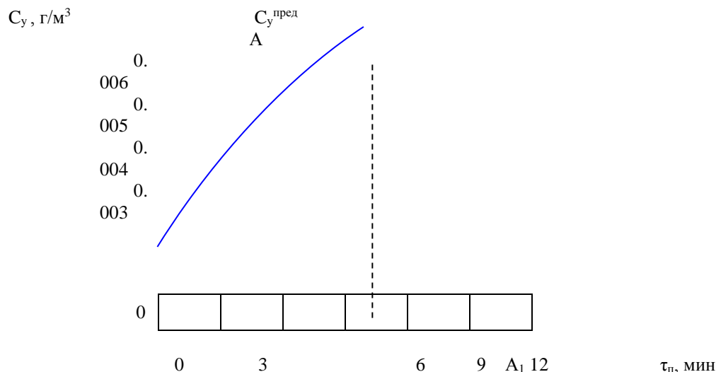
Рис. Изменение концентрации окиси углерода (CO) в горящем помещении: A-A 1 – момент наступления смертельной концентрации окиси углерода в помещении; C y пред – предельная концентрация токсичного газа на уровне рабочей зоны спасателя.
