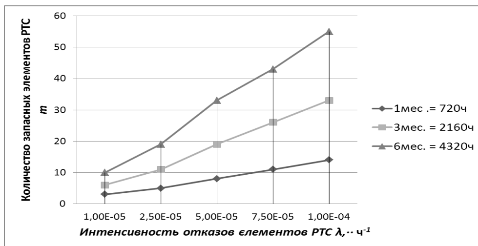
Рис. 1. График функции m = f(N, \lambda, t_n) , при N=100 ; T_n=720ч; 2160ч; 4320ч, \lambda=10^{-5} - 10^{-4} ч^{-1}
