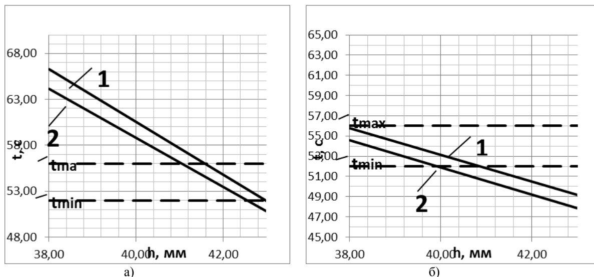
Рисунок 3 – Залежності часу підвищення температури мідного блоку в інтервалі від 98 °С до 703 °С (залежність 1) та від 102 °С до 697 °С (залежність 2) від висоти полум'я для пальника потужністю 500 Вт на газі метані (а) та на газі пропан-бутані (б)
