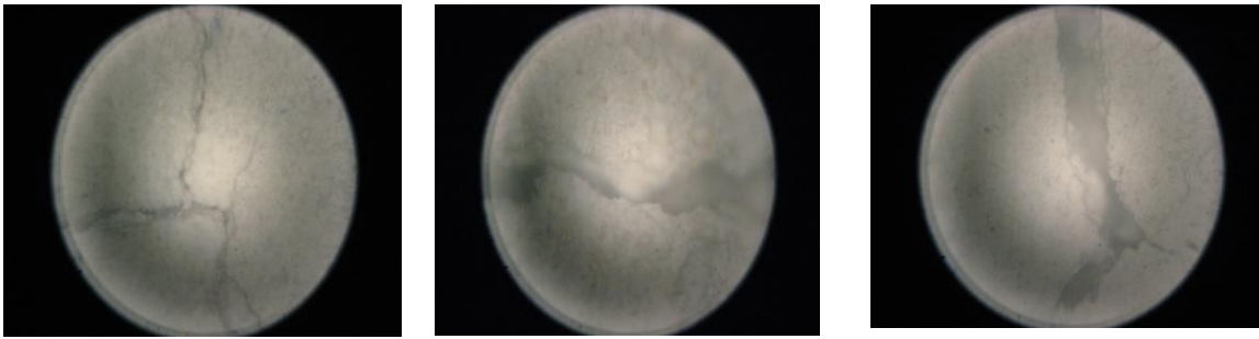
Рисунок 1 – Фотоснимки изменения структуры образцов ячеистого газобетона после температурных воздействий зафиксированные на микроскопе МЕТАМ ЛВ - 32: а – 100°С; б – 200°С; в – 300°С; г – 400°С; д – 500°С; е – 600°С; ж – 700°С; з – 800°С; и – 900°С; к – 1000°С.
