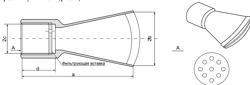
Рисунок 1. Насадок на пожежний лафетний ствол для створення плоскорадіального водяного струменя-екрана.
