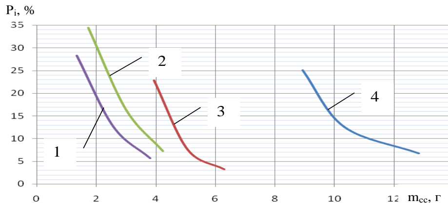
Рисунок 1 - Влияние Екосепт на разные сорта древесины: 1 - ясень; 2 - дуб; 3 - ольха; 4 - липа
