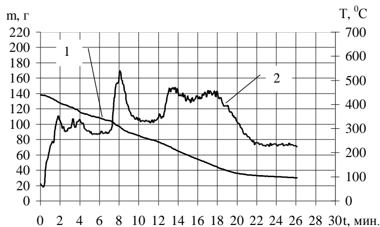
Рисунок 2. - Зависимость массы и ТДГ образца древесины после удаления ксерогелевого слоя ГОС Na_2O-2,95SiO_2 - K_2CO_3 при его сгорании: 1 - масса образца; 2 – температура
