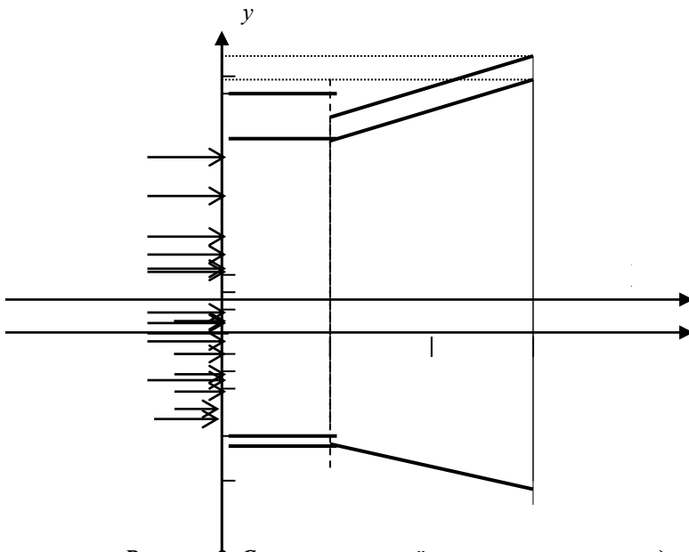
Рисунок 2. Схема проточної частини каналу насадки на пожежній лафетній ствол для створення плоскорадіального водяного струменя-екрана.
