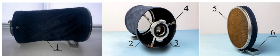
Рис. Будова ППГ: 1 – гнучкий циліндричний корпус; 2 – з'єднувальна головка; 3 – розпилувач; 4 – опорна вставка; 5 – набір латунних сіток; 6 – ручка для утримування.
