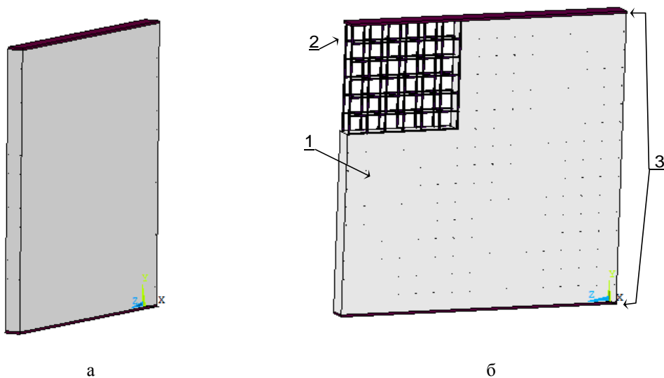
Рисунок 1 - Схема расчетной области железобетонной несущей стены для проведения расчета предела огнестойкости (а - общий вид, который используют для
