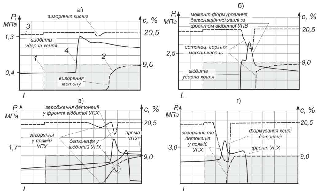
Рис. 3. Профілі тисків і концентрацій газів при різних ефектах ініціювання локальних скупчень метану: а) спалах у відбитій хвилі, б) займання та детонація у відбитій хвилі, в) запалення в падаючій і детонація у відбитій хвилі, г) займання та детонація в падаючій хвилі; 1 – профіль початкової концентрації метану у локальному скупченні, 2 – концентрація метану при проходженні УПХ, 3 – концентрація кисню, 4 – тиск у відбитій хвилі
