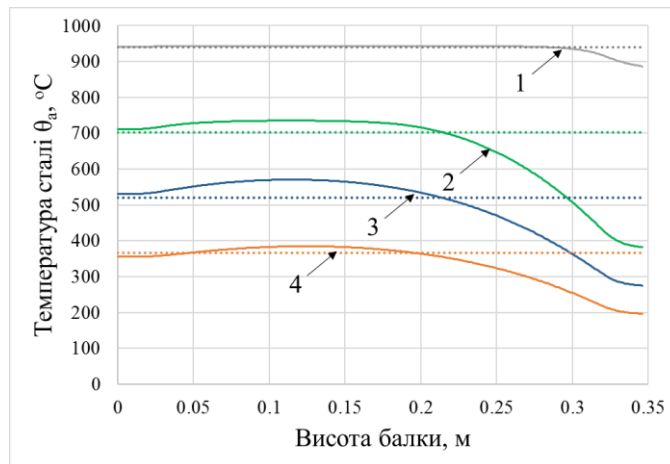
Рисунок – Зміння температури сталі по висоті балки для часу 60 хв вогневого впливу для рівномірного (пунктирні лінії) і нерівномірного (суцільні лінії) розподілів температури для таких варіантів: 1 – незахищена сталева балка; 2, 3, 4 – захищена сталева балка з покриттям завтовшки 10 мм, 15 мм та 20 мм
