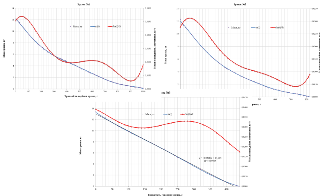
Рисунок 2 – Залежності зміни маси зразків та масової швидкості вигорання від тривалості горіння
