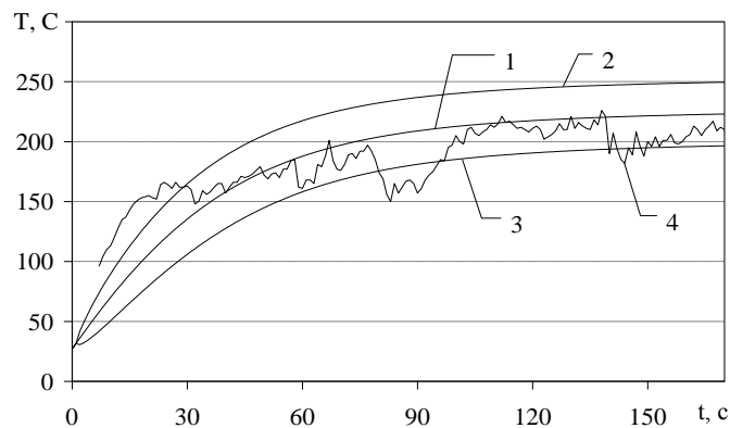
Рис. 2. Динаміка зміни температури термомпари на стінці моделі резервуара, оберненої в бік полум'я: 1 – математичне очікування; 2, 3 – верхня і нижня межі інтервалу \pm 3\sigma ; 4 – результати експерименту
