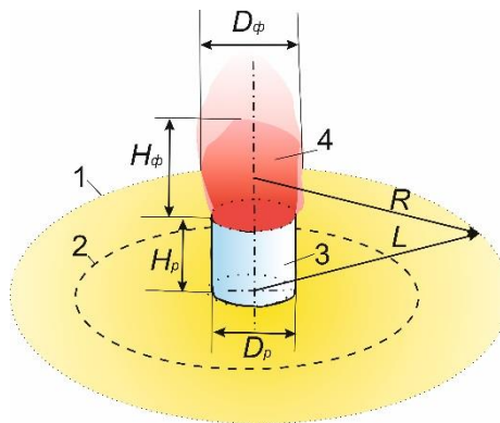
Рисунок 1 Параметри обстановки при горінні нафтопродуктів в резервуарі:
