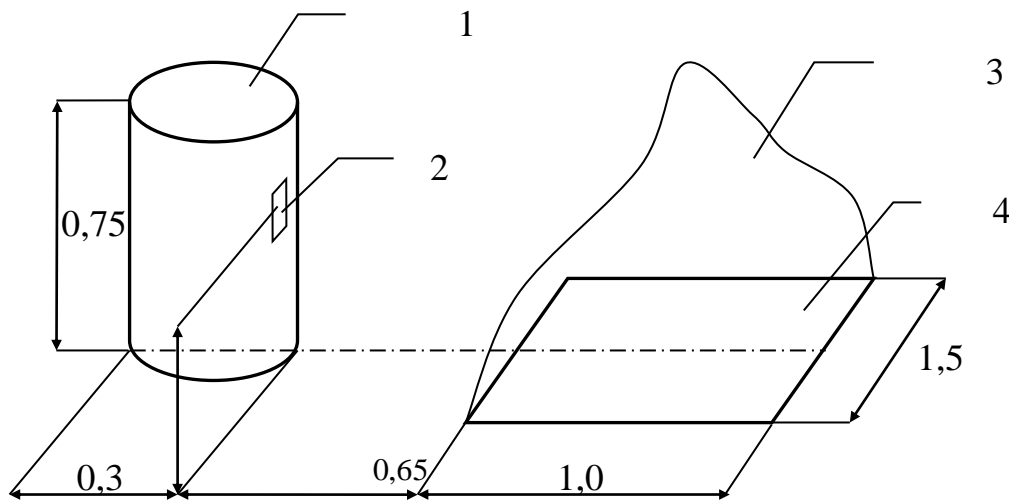
Рис. 1. Схема експерименту: 1 – модель резервуара; 2 – термopар; 3 – полум'я; 4 – піддон з нафтопродуктом
