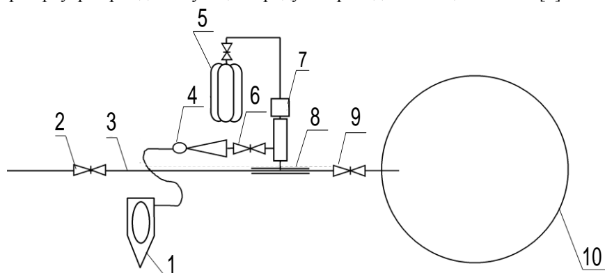
1 – пожарный аварийно-спасательный автомобиль; 2, 6, 9 – шаровый кран (завдвижка); 3 – действующий продуктопровод; 4 – высоконапорный генератор пены; 5 – источник сжатого воздуха; 7 – устройство врезки; 8 – бандаж; 10 – резервуар Рисунок 1 – Принципиальная схема реализации способа подачи воздушно-механической огнетушащей пены в резервуар через действующий продуктопровод
