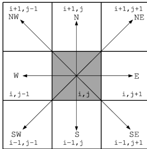
Рис.1 – Moore-подібне прилягання
