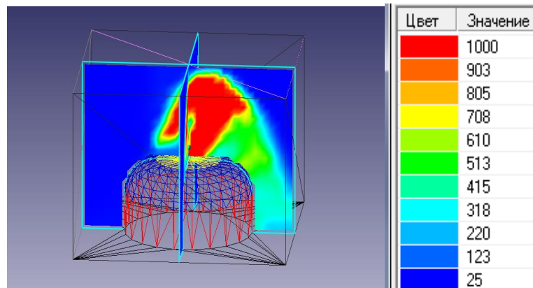
Рис. 1. Факел полум'я.
