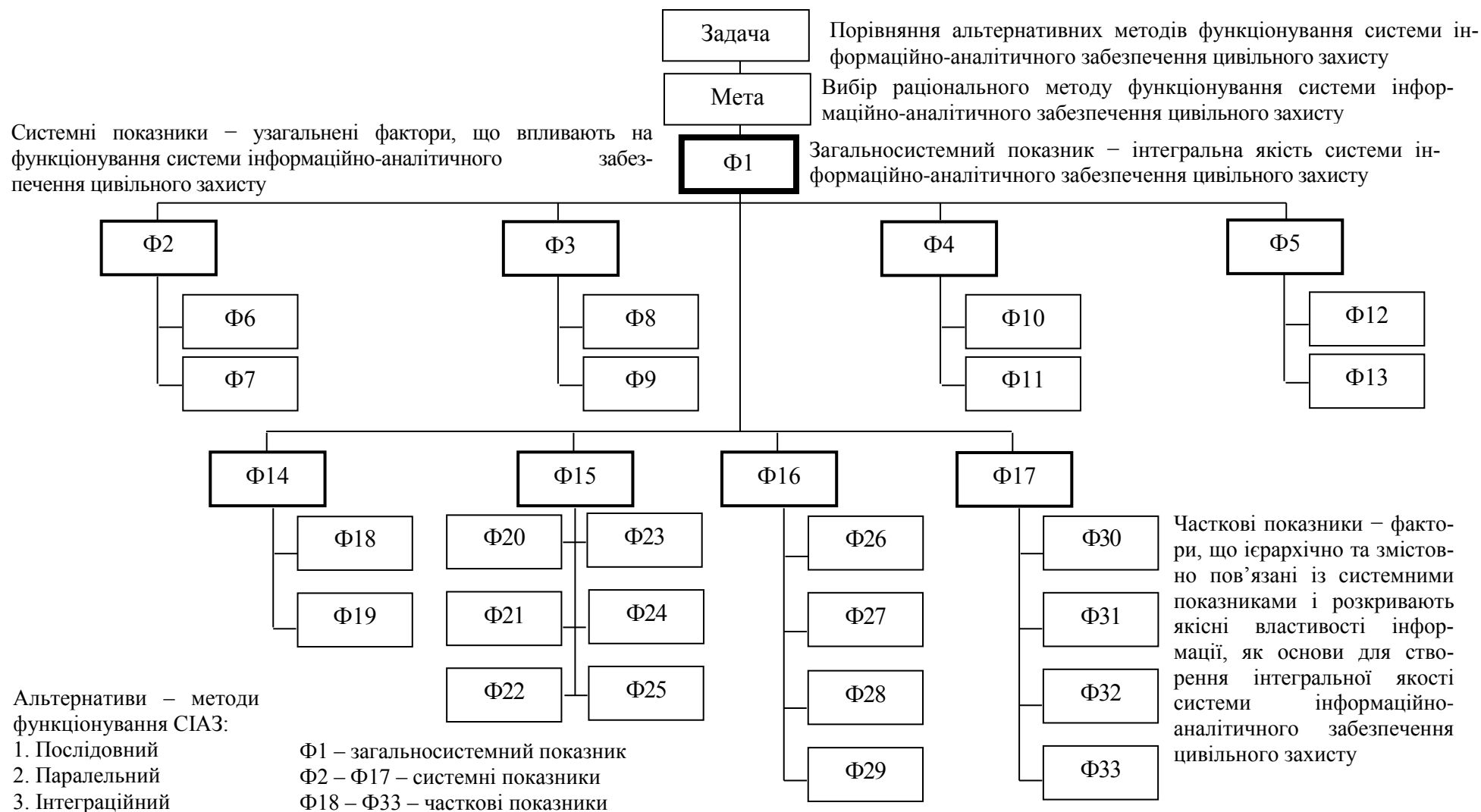
Рис. 2. Ієрархичний та змістовний взаємозв'язок в системі показників для побудови ієрархічної моделі порівняння альтернативних методів функціонування CIA3 ЦЗ
