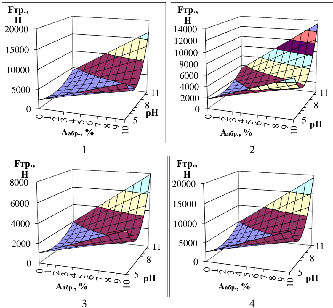
Рис. 4.5. Розрахункові значення сили тертя натурної трібосистеми екструдера ЕВ-350, «наконечник – філь’єра №5»:
