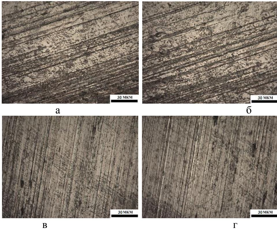
Рис. 5.4 – Мікрофотографії поверхонь тертя сталей при використанні слаболужного середовища, рН 8 та 10% абразиву (x600): а – сталь 40Х; б – чавун ЧХ22Н2; в – сталь 95Х18; г – чавун ЧХ32
