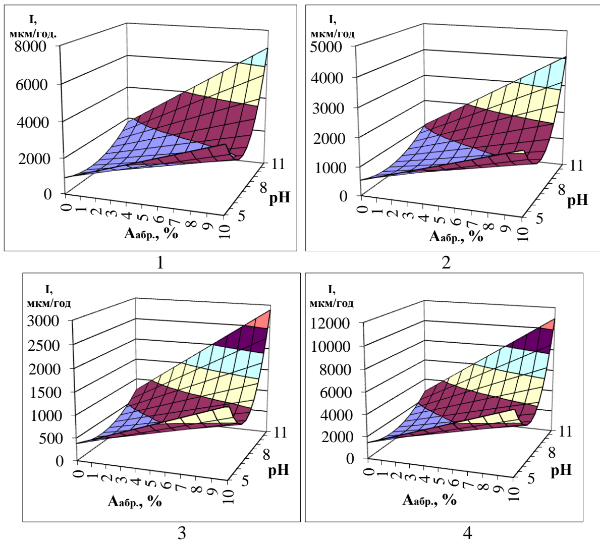
Рис. 4.2. Розрахункові значення швидкості зношування натурної трібосистеми екструдера ЕВ-350, «хвостовик – філь'єра №4»:
