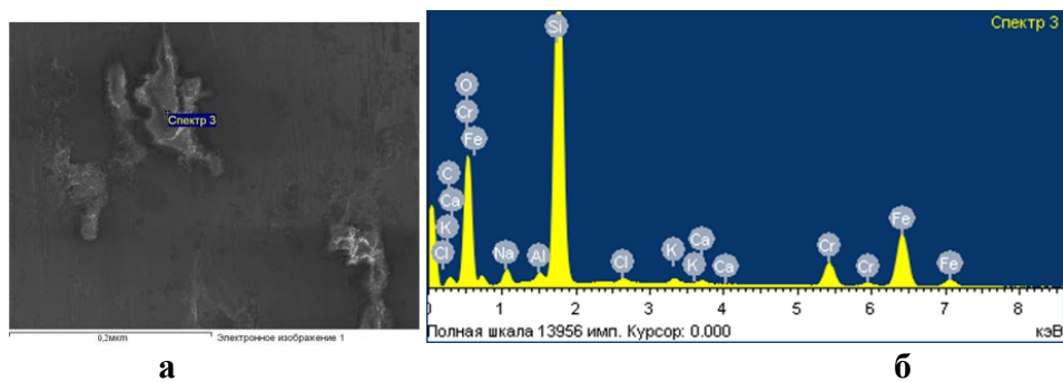
Рис. Б.43 – Хімічний аналіз поверхні тертя чавуна ЧХ32 при рН 11 та абразивності 10% спектр 3:
