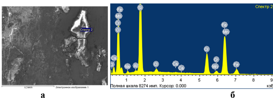
Рис. Б.31 – Хімічний аналіз поверхні тертя чавуна ЧХ32 при рН 8 та абразивності 10% спектр 2: а – мікрофотографія поверхні тертя при збільшенні 0,2 мкм; б – металографічна діаграма
