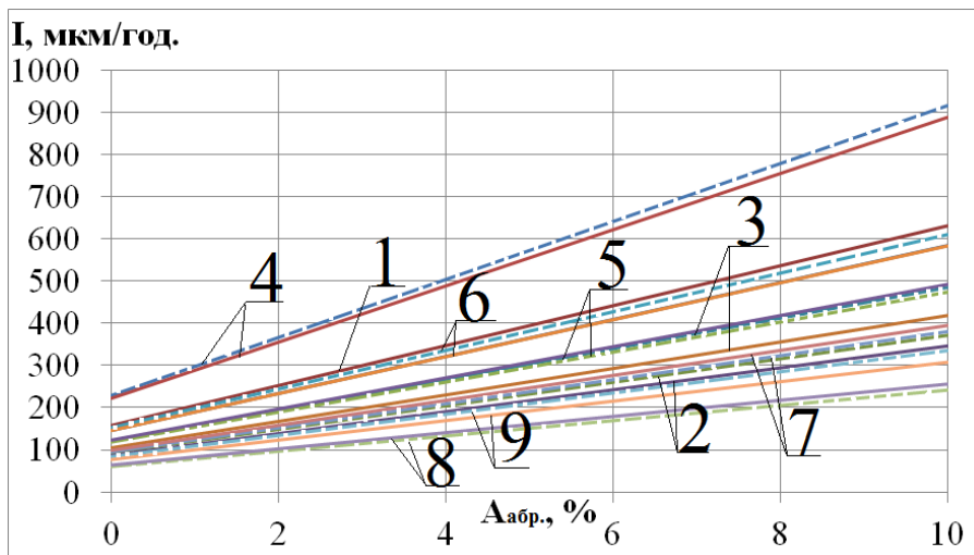
Рис. 3.11 – Теоретичні та експериментальні залежності швидкості зношування трібо-систем від абразивності при постійній активній кислотності та навантаженню:
