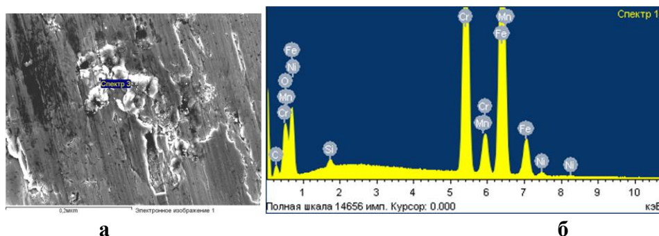
Рис. Б.38 – Хімічний аналіз поверхні тертя базового чавуна ЧХ22Н2 при рН 11 та абразивності 10% спектр 1:
