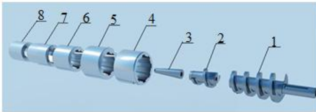
Рис. 2.1 – Зовнішній вигляд основних трібосистем EB-350:
