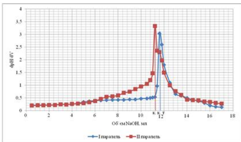
Рис. 3.2 – Диференціальна крива титрування I порядку деревинної жишки 0,1 нормальним розчином гідроксиду натрію
