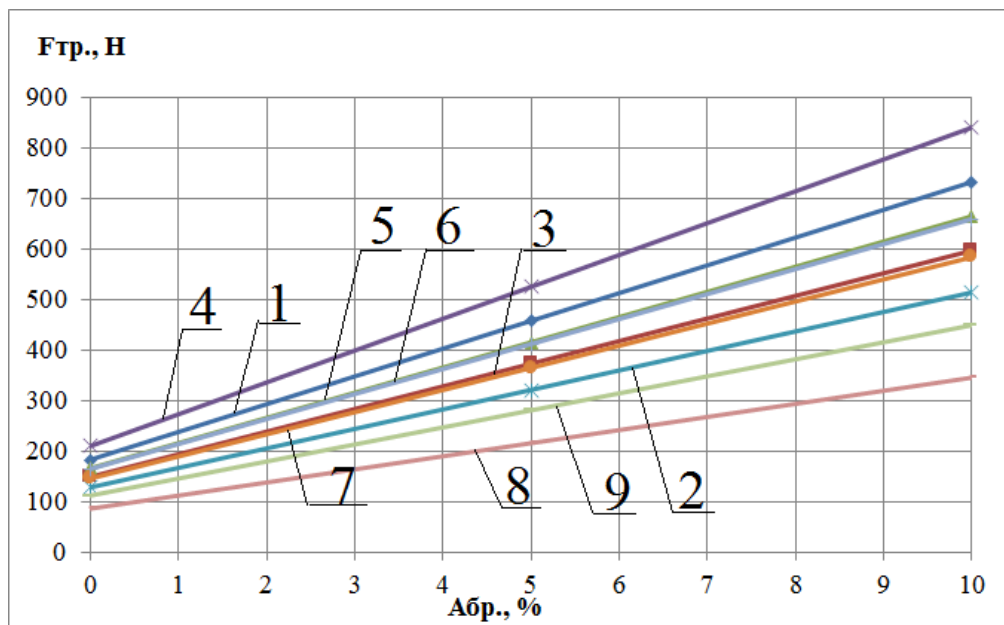
Рис. 3.12 – Залежності сили тертя трібо-систем від рівня абразивності при постійному навантаженні та рівня активної кислотності:
