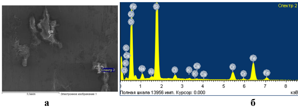
Рис. Б.42 – Хімічний аналіз поверхні тертя чавуна ЧХ32 при рН 11 та абразивності 10% спектр 2:
