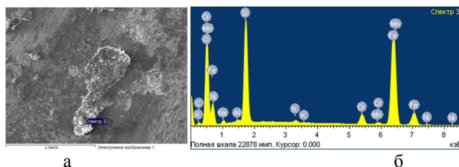
Рис. Б.3 – Хімічний аналіз поверхні тертя базового чавуна ЧХ22Н2 при рН 5 та абразивності 10% спектр 3:
