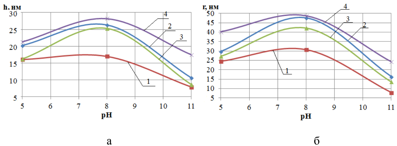
Рис. 5.7 – Залежності товщини захисних плівок h та глибини подряпин r поверхень тертя зразків модельних трібосистем екструдера EB-350 та EB-350M від рівня активної кислотності з вмістом абразиву 10 % в масі:
