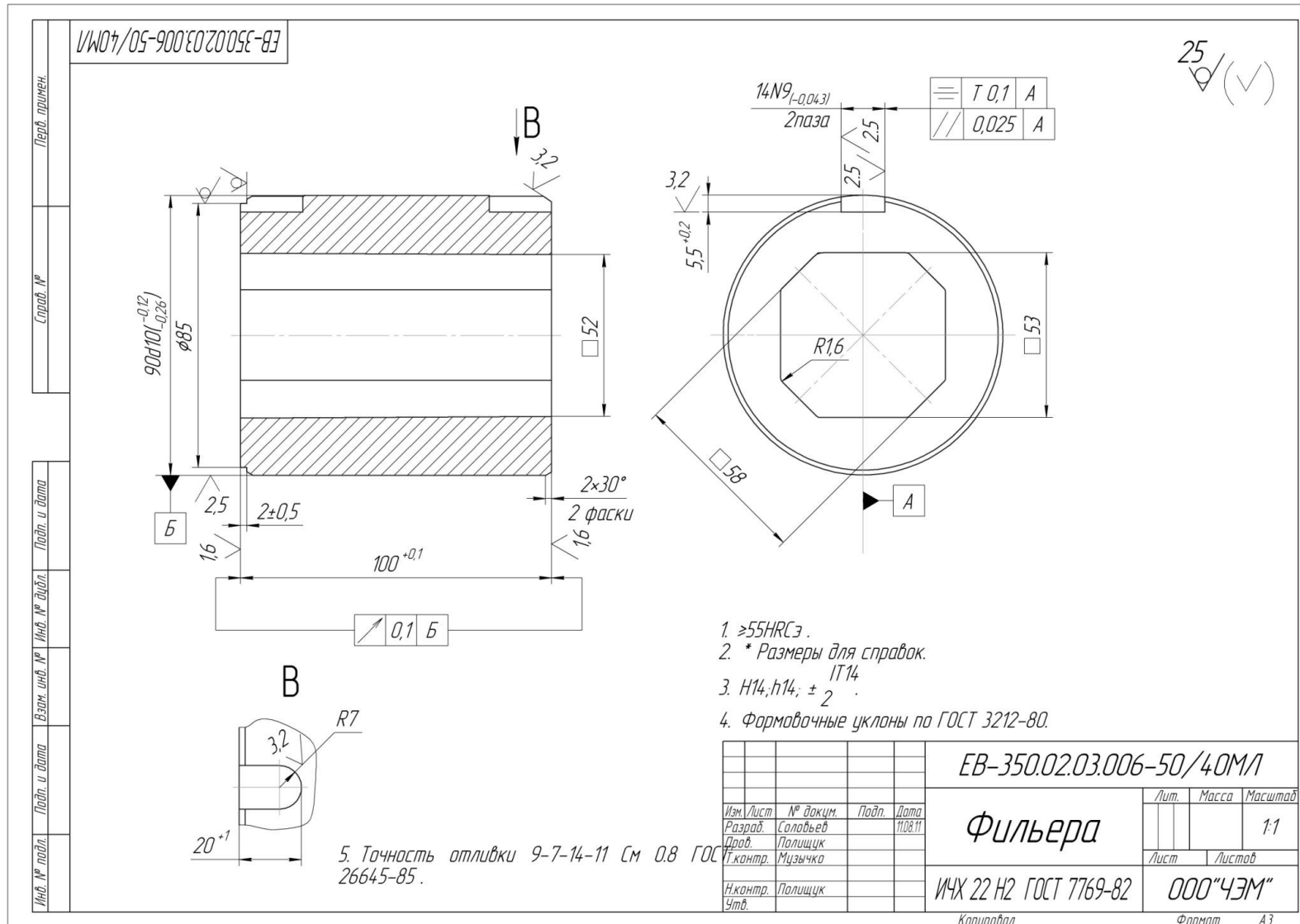
Рис. А8 – Філь’єра EB-350.02.03.006-50/40МЛ
