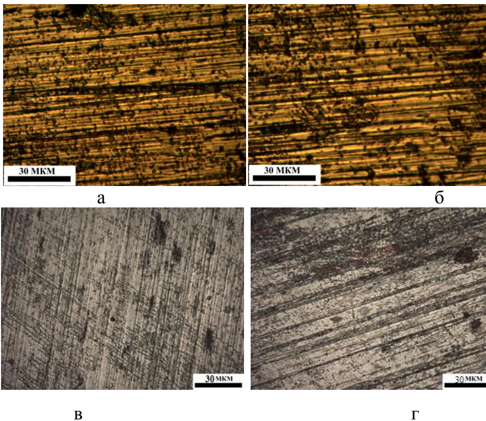
Рис. 5.2 – Мікрофотографії поверхонь тертя сталей при використанні слабокислого середовища, рН 5 та 10% абразиву (x600): а – сталь 40Х; б – чавун ЧХ22Н2; в – сталь 95Х18; г – чавун ЧХ32
