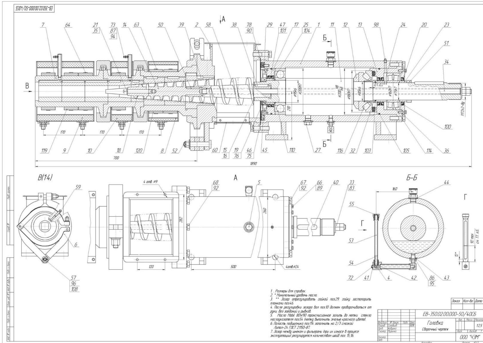
Рис. А1 – Головка. Складальные кресления экструдера ЭБ-350
