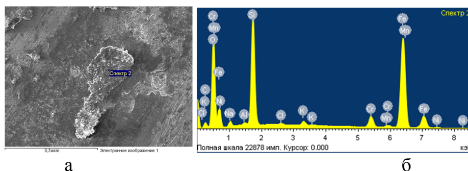
Рис. Б.2 – Хімічний аналіз поверхні тертя базового чавуна ЧХ22Н2 при рН 5 та абразивності 10% спектр 2:
