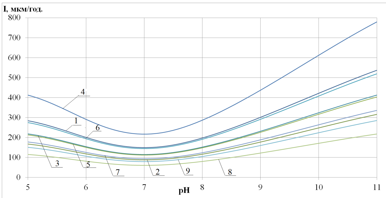
Рис. 3.4 – Теоретичні залежності швидкості зношування трібосистем від рівня активної кислотності при постійній абразивності 0% та навантаженню 1000 Н:
