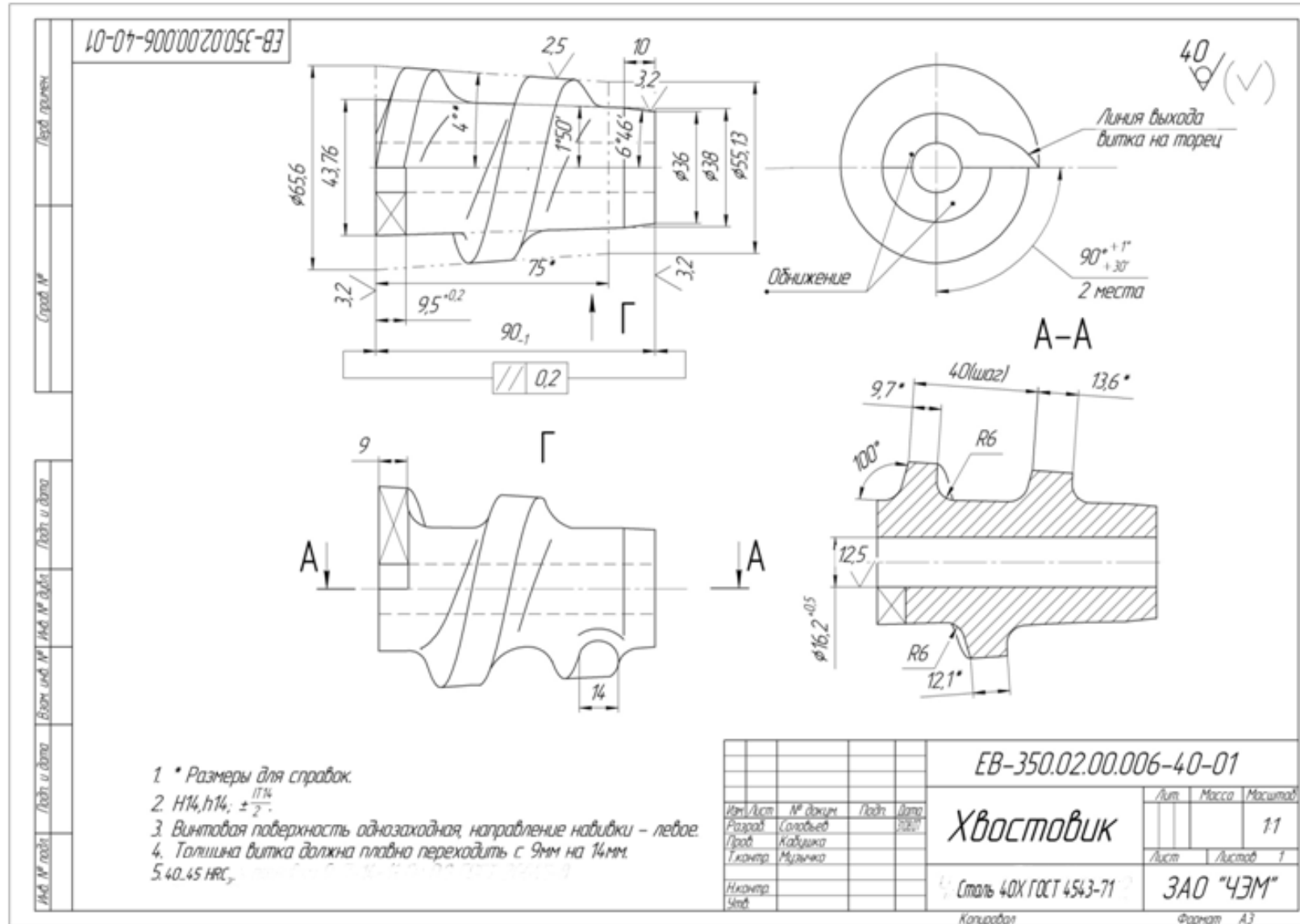
Рис. А2 – Хвостовик EB-350.02.03.006-40-01
