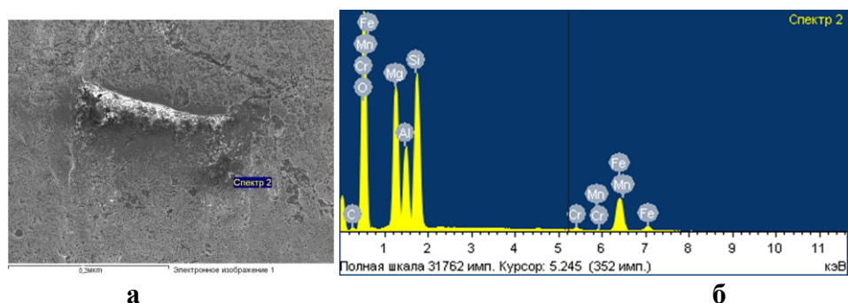
Рис. Б.15 – Хімічний аналіз поверхні тертя базової сталі 40X при рН 5 та абразивності 10% спектра 2:
