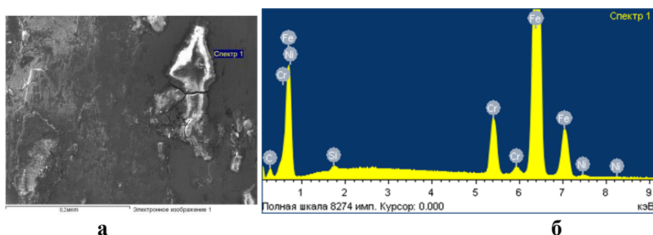
Рис. Б.30 – Хімічний аналіз поверхні тертя чавуна ЧХ32 при рН 8 та абразивності 10% спектр 1: а – мікрофотографія поверхні тертя при збільшенні 0,2 мкм; б – металографічна діаграма
