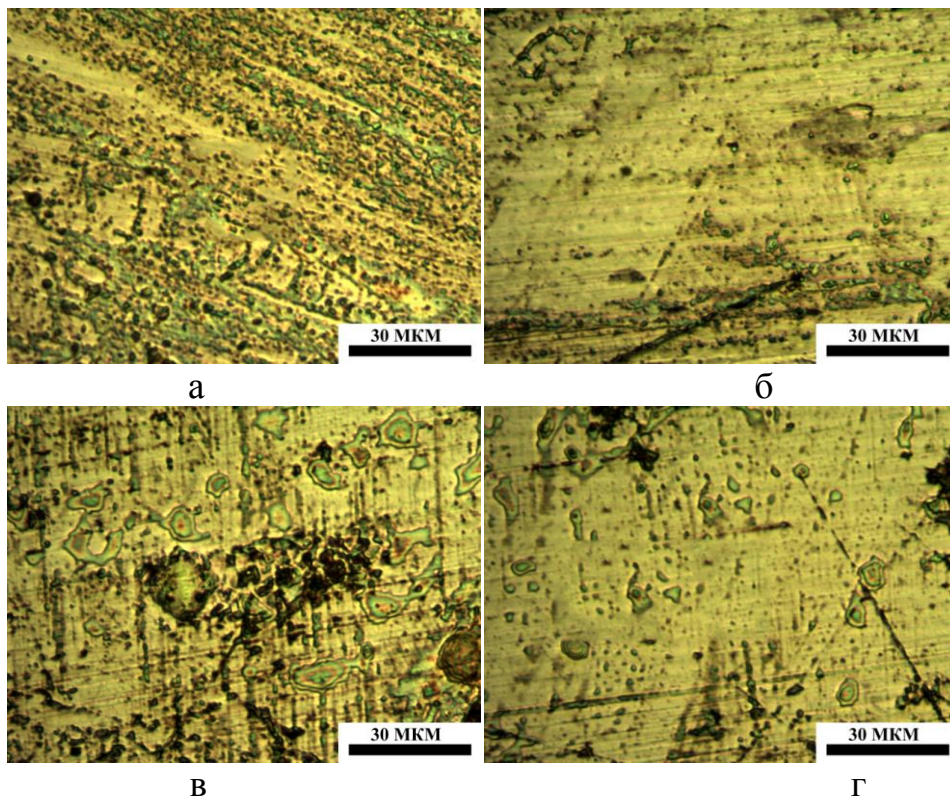
Рис. 5.5– Мікрофотографії поверхонь тертя сталей при використанні сильнолужного середовища, рН 11, без абразиву (x600): а – сталь 40Х; б – чавун ЧХ22Н2; в – сталь 95Х18; г – чавун ЧХ32
