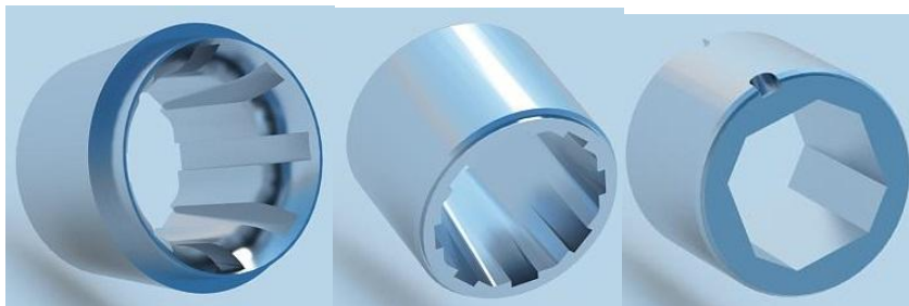
Рис. 2.10 – Зворотна трібосистема за матеріалами та геометрією «шнек конічний + філь'єра №1, 2 та 3»
