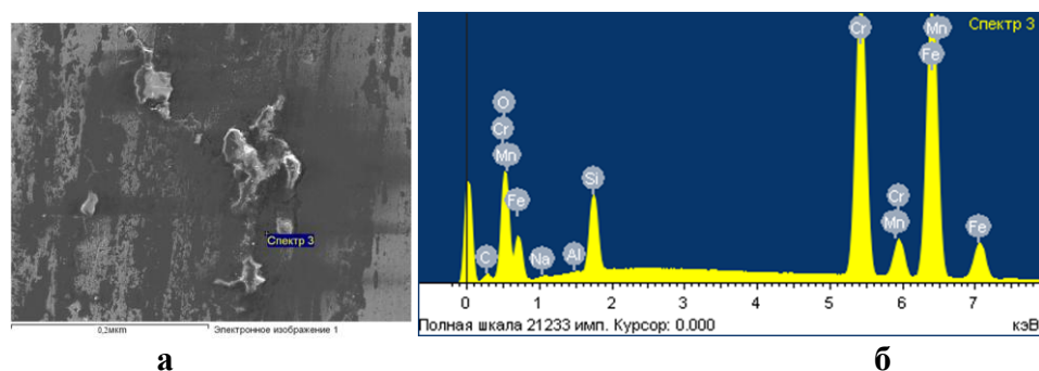
Рис. Б.11 – Хімічний аналіз поверхні тертя підбраного чавуна ЧХ32 при рН 5 та абразивності 10% спектр 3:
