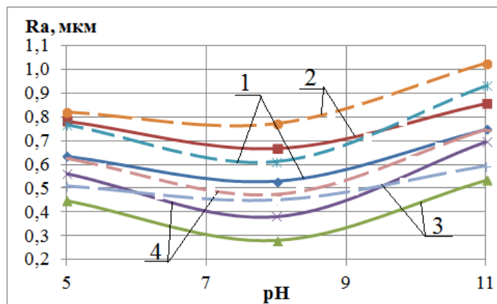
Рис. 5.8 – Залежності шорсткості робочих поверхонь тертя зразків модельних трібосистем екструдера ЕВ-350 та ЕВ-350М від рівня активної кислотності:
