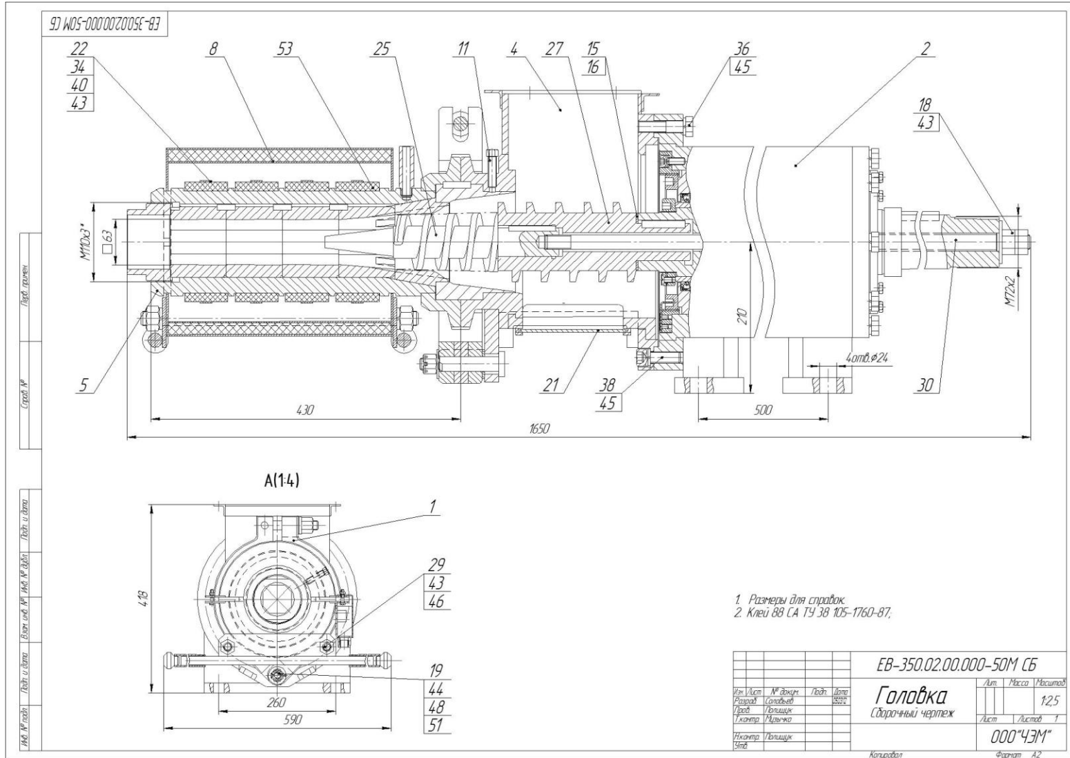
Рис. А12 – Головка. Складальне креслення екструдера EB-350M
