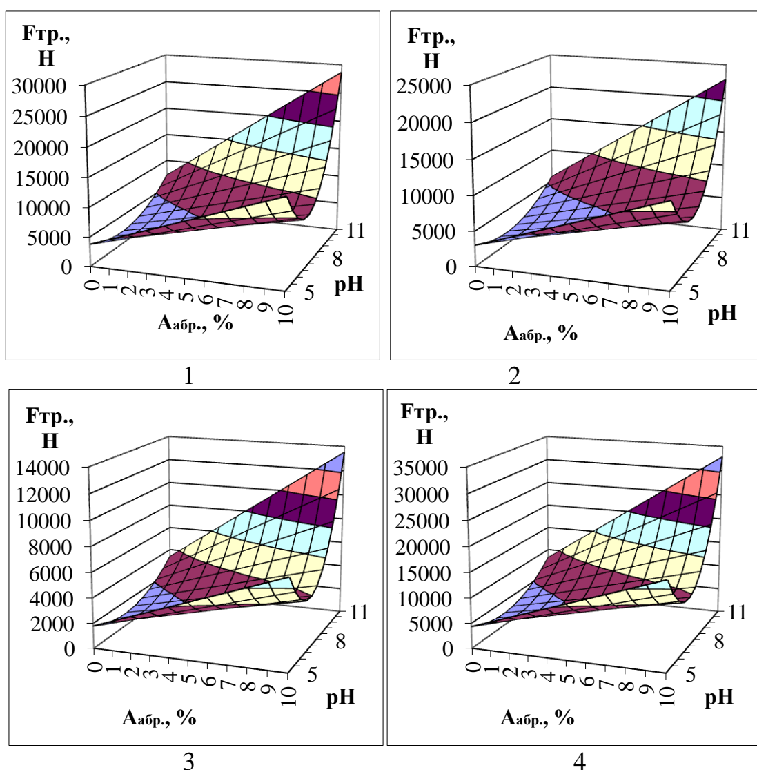
Рис. 4.7 – Розрахункові значення сили тертя натурної трібосистеми екструдера ЕВ-350, «шнек конічний – філь’єра №1, 2 та 3»:
