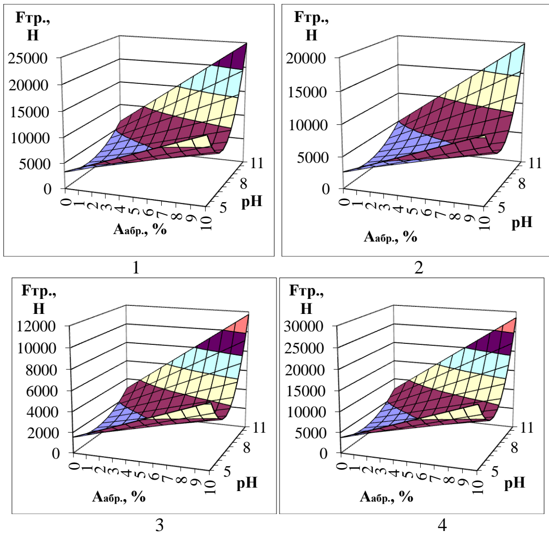
Рис. 4.8 – Розрахункові сили тертя натурної трібосистеми екструдера ЕВ-350М, «шнек конічний – філь’єра №1, 2 та 3»:
