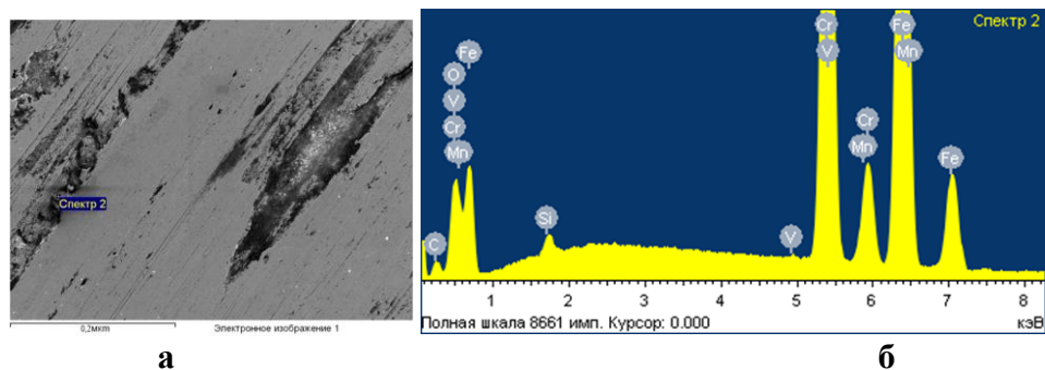
Рис. Б.20 – Хімічний аналіз поверхні тертя підбраної сталі 95X18 при рН 5 та абразивності 10% спектр 2:
