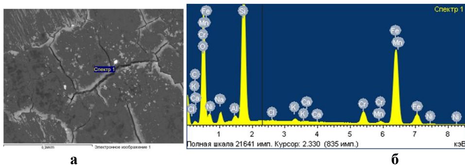
Рис. Б.8 – Хімічний аналіз поверхні тертя базового чавуна ЧХ22Н2 при рН 5 та абразивності 10% спектр 1:
