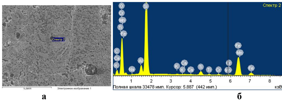
Рис. Б.18 – Хімічний аналіз поверхні тертя базової сталі 40X при рН 5 та абразивності 10% спектр 2:
