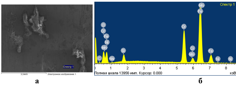
Рис. Б.41 – Хімічний аналіз поверхні тертя чавуна ЧХ32 при рН 11 та абразивності 10% спектр 1:
