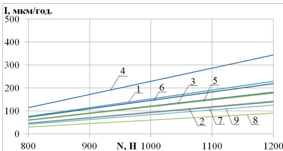
Рис. 3.6 – Теоретичні залежності швидкості зношування трібосистем від навантаження при постійній активній кислотності рН 8 та абразивності 0%:
