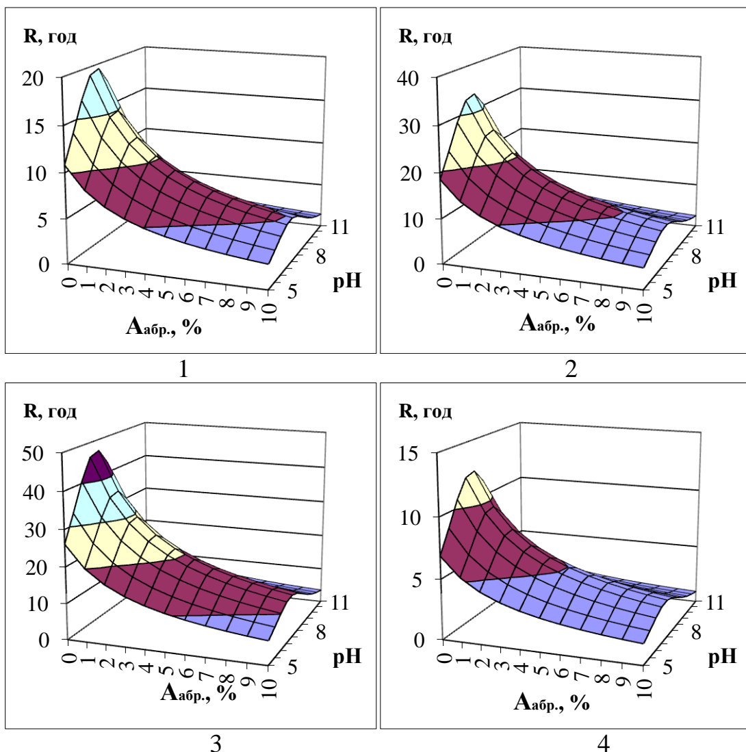
Рис. 4.10 – Розрахункові значення ресурсу натурної трібосистеми екструдера ЕВ-350, «хвостовик – філь’єра №4»:
