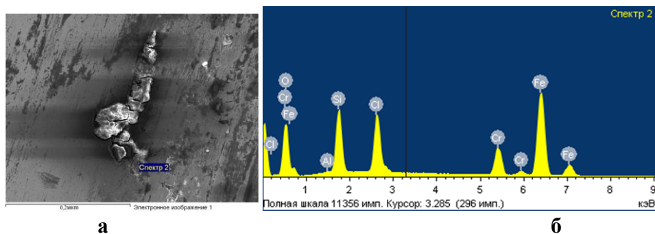
Рис. Б.26 – Хімічний аналіз поверхні тертя сталі 95X18 при рН 8 та абразивності 10% спектр 2:
