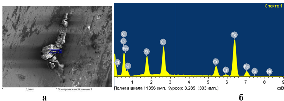
Рис. Б.25 – Хімічний аналіз поверхні тертя базової сталі 40X при рН 5 та абразивності 10% спектр 1:
