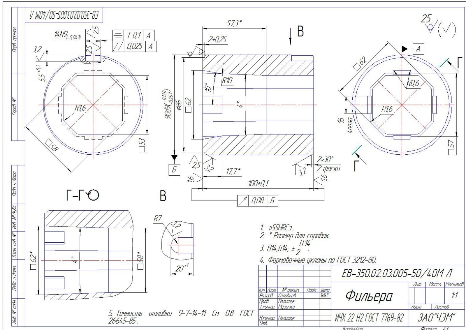
Рис. 7А – Філь'єра EB-350.02.03.005-50/40ML
