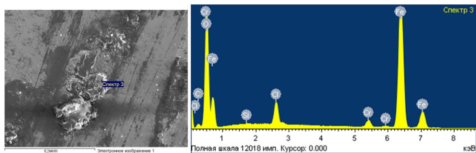
Рис. Б.35 – Хімічний аналіз поверхні тертя підбраної сталі 95X18 при рН 11 та абразивності 10% спектр 3:
