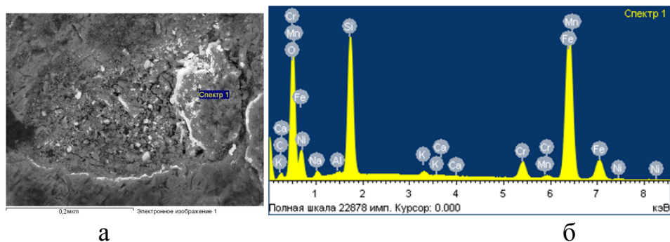
Рис. Б.4 – Хімічний аналіз поверхні тертя базового чавуна ЧХ22Н2 при рН 5 та абразивності 10% спектр 1:
