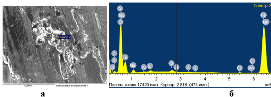
Рис. Б.37 – Хімічний аналіз поверхні тертя базової сталі 40X при рН 11 та абразивності 10% спектр 2:
