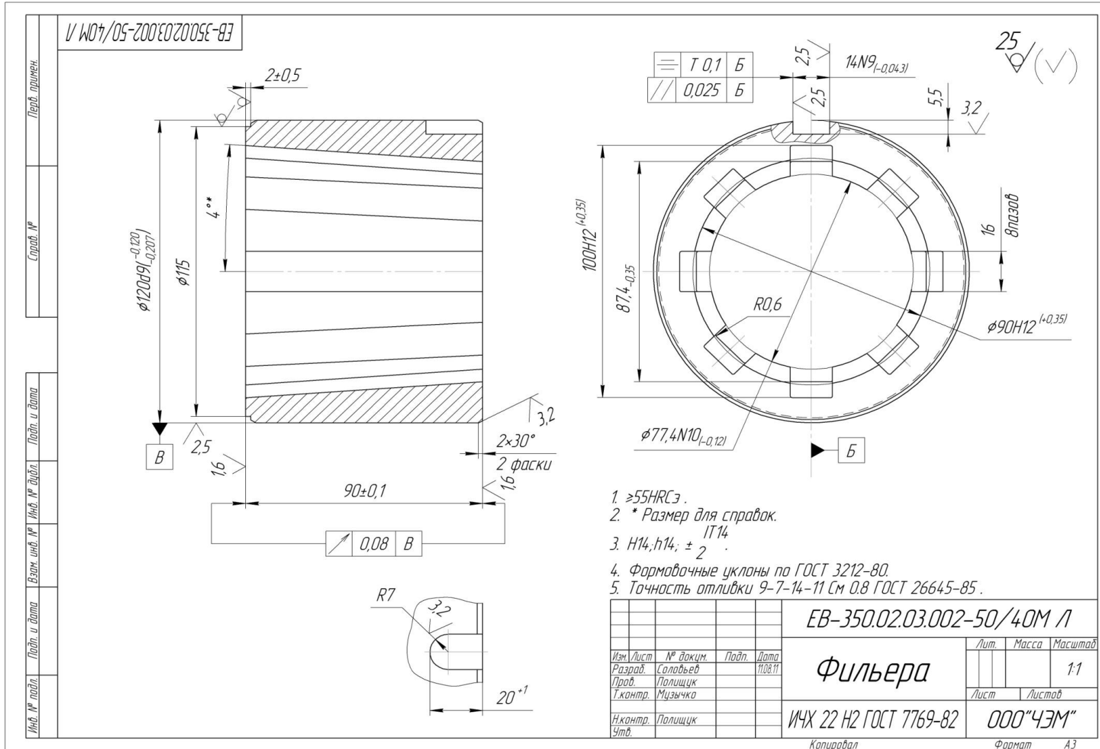
Рис. А4 – Філь'ера EB-350.02.03.002-50/40МЛ
