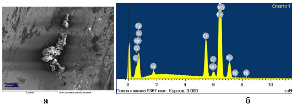
Рис. Б.27 – Хімічний аналіз поверхні тертя сталі 95X18 при рН 8 та абразивності 10% спектр 1:
