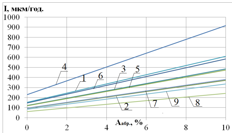
Рис. 3.5 – Теоретичні залежності швидкості зношування трібосистем від абразивності при постійній активній кислотності рН 8 та навантаженню 1000 Н:
