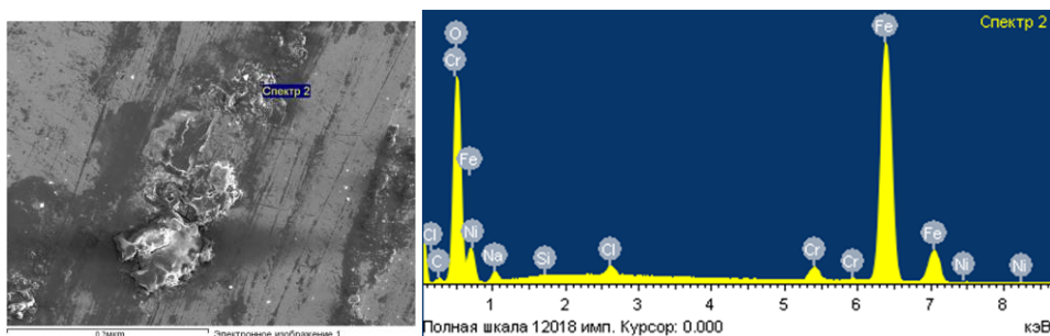
Рис. Б.34 – Хімічний аналіз поверхні тертя підбраної сталі 95X18 при рН 11 та абразивності 10% спектр 2:
