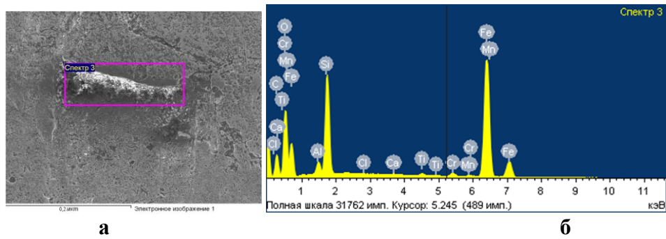
Рис. Б.16 – Хімічний аналіз поверхні тертя базової сталі 40X при рН 5 та абразивності 10% спектр 3:
