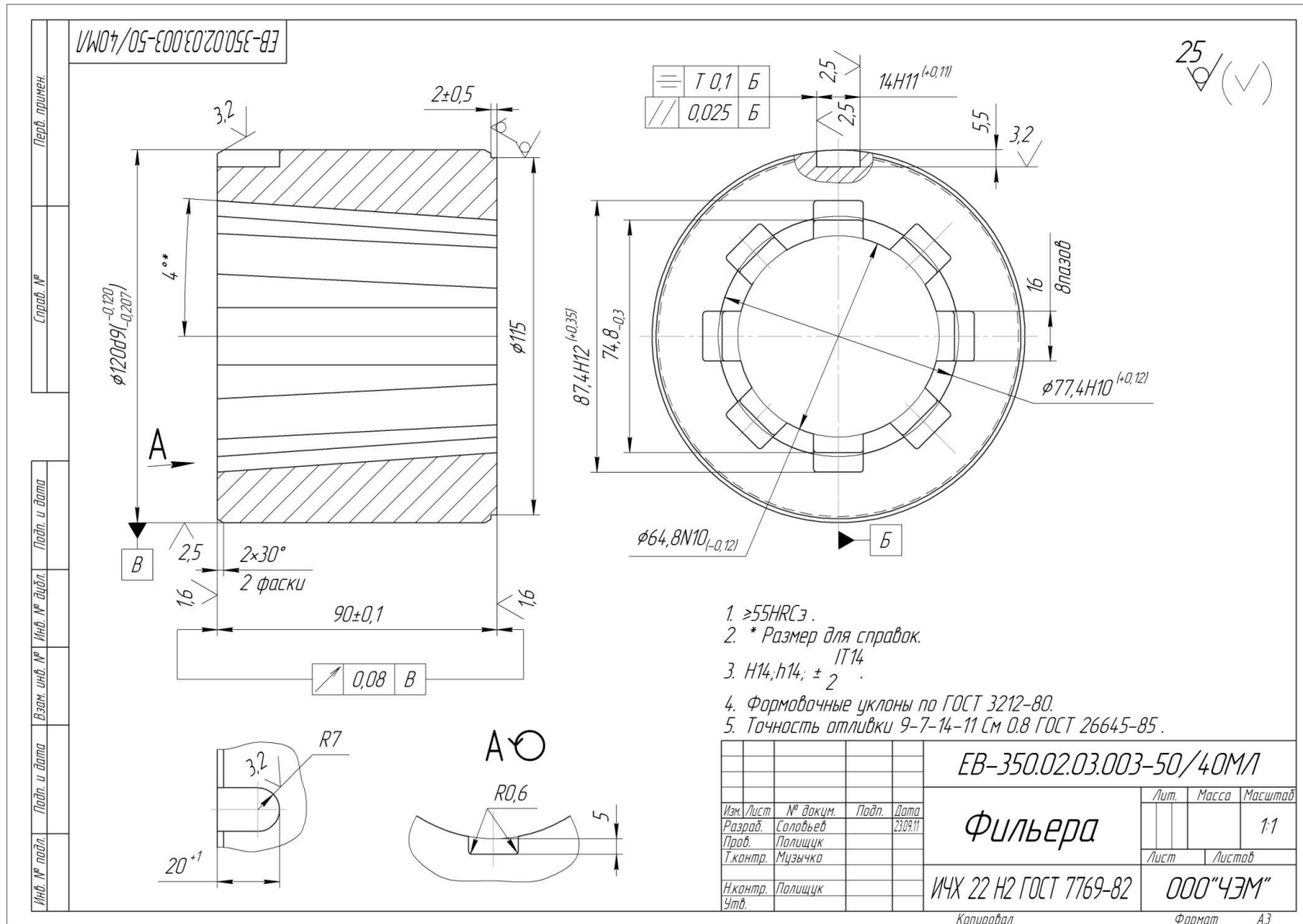
Рис. А5 – Філь'єра EB-350.02.03.003-50/40МЛ
