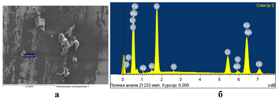
Рис. Б.13 – Хімічний аналіз поверхні тертя підбраного чавуна ЧХ32 при рН 5 та абразивності 10% спектра 5:
