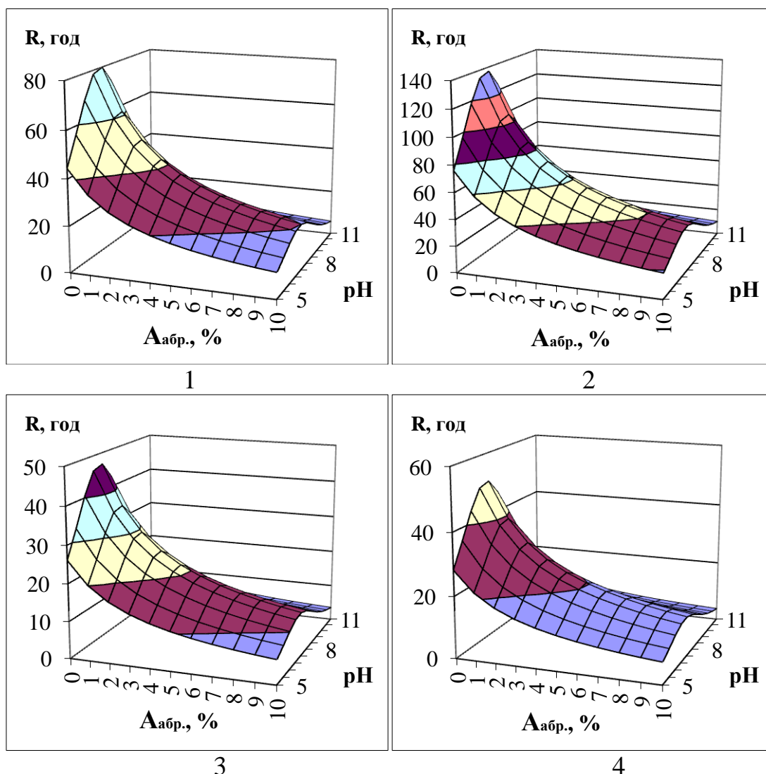
Рис. 4.11 – Розрахункові значення ресурсу натурної трібосистеми екструдера ЕВ-350, «шнек конічний – філь’єра №1, 2 та 3»:
