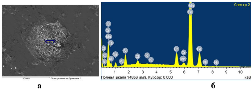
Рис. Б.40 – Хімічний аналіз поверхні тертя базового чавуна ЧХ22Н2 при рН 11 та абразивності 10% спектр 2:
