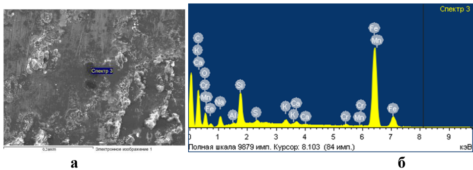
Рис. Б.24 – Хімічний аналіз поверхні тертя базової сталі 40X при рН 5 та абразивності 10% спектр 3:
