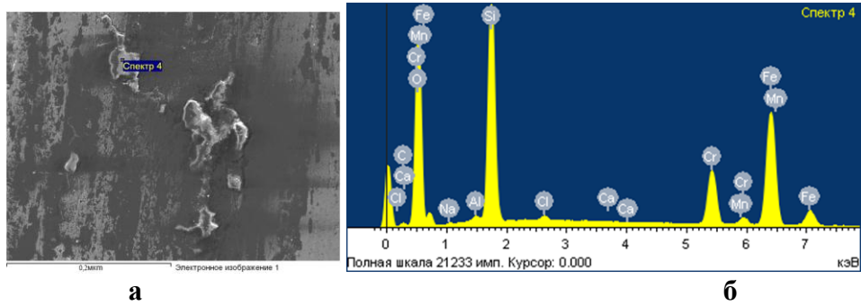
Рис. Б.12 – Хімічний аналіз поверхні тертя підбраного чавуна ЧХ32 при рН 5 та абразивності 10% спектра 4:
