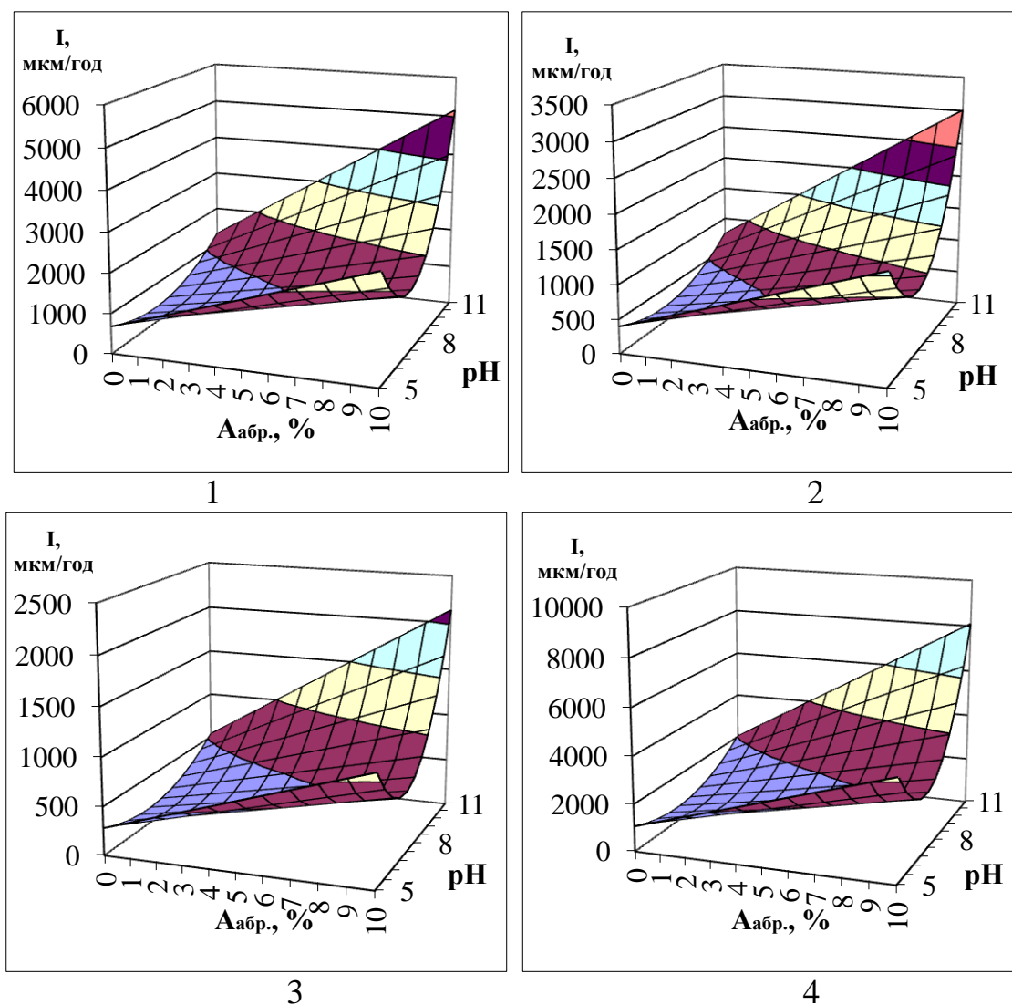
Рис. 4.1. Розрахункові значення швидкості зношування натурної трібосистеми екструдера EB-350, «наконечник – філь’єра №5»:
