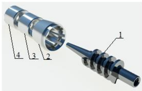
Рис. 2.2. Зовнішній вигляд основної трібосистем EB-350M:
