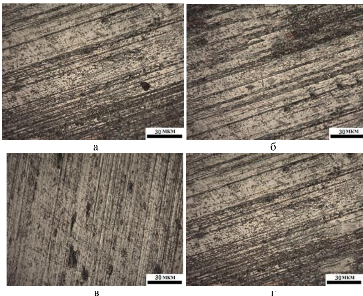
Рис. 5.6 – Мікрофотографії поверхонь тертя чавунів при використанні сильнолужного середовища, рН 11 та 10% абразиву (х600):
