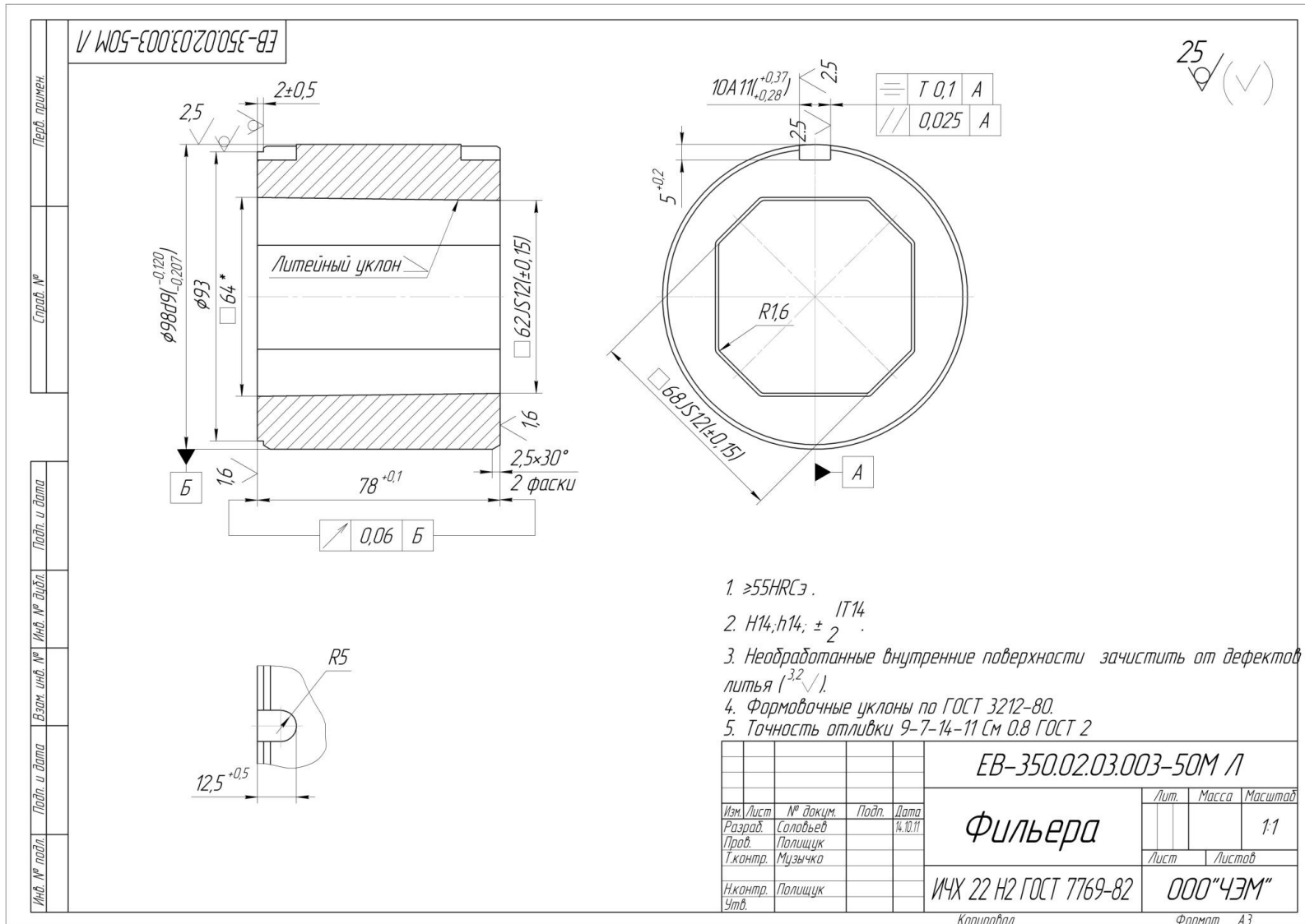
Рис. А15 – Филь’ера EB-350.02.03.003-50M Л
