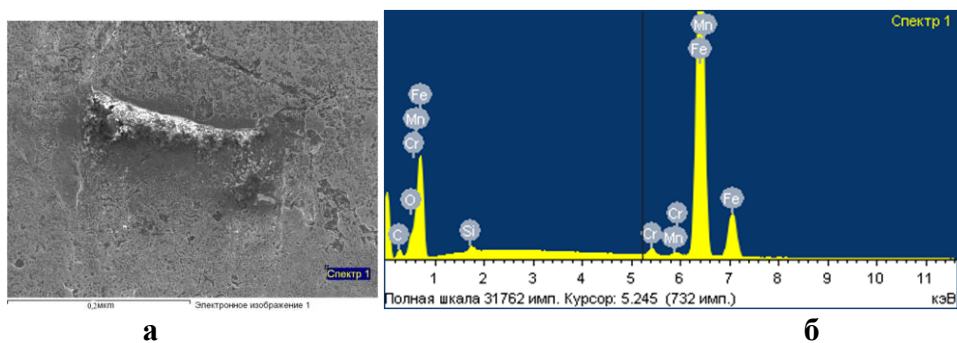
Рис. Б.14 – Хімічний аналіз поверхні тертя базової сталі 40X при рН 5 та абразивності 10% спектра 1:
