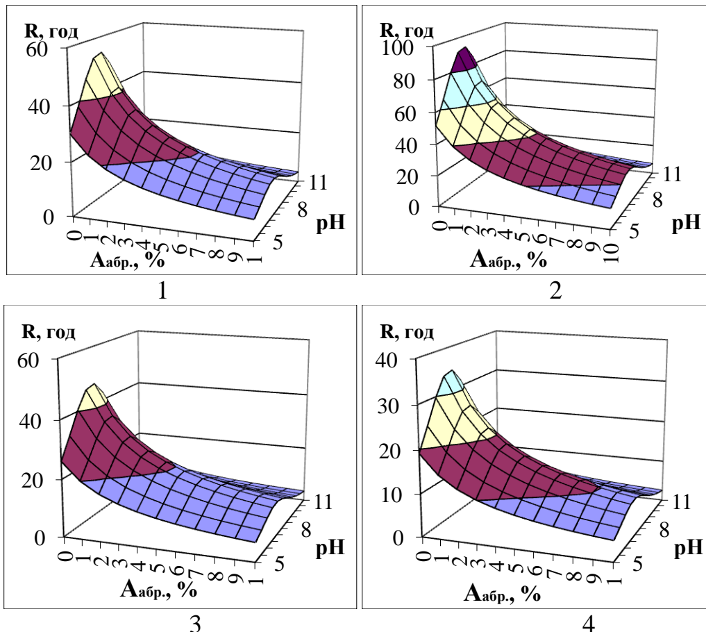
Рис. 4.12 – Розрахункові значення ресурсу натурної трібосистеми екструдера ЕВ-350М, «шнек конічний – філь’єра №1, 2 та 3»:
