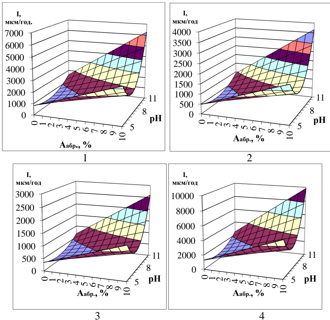
Рис. 4.4 – Розрахункові значення швидкості зношування натурної трібосистеми екструдера ЕВ-350М, «шнек конічний – філь’єра №1, 2 та 3»:
