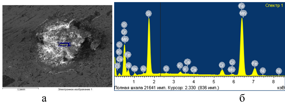
Рис. Б.7 – Хімічний аналіз поверхні тертя базового чавуна ЧХ22Н2 при рН 5 та абразивності 10% спектр 1:
