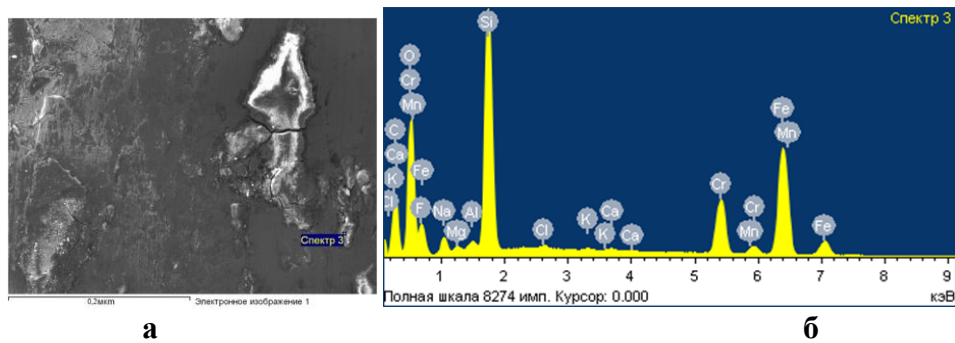
Рис. Б.32 – Хімічний аналіз поверхні тертя чавуна ЧХ32 при рН 8 та абразивності 10% спектр 3:
