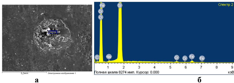
Рис. Б.28 – Хімічний аналіз поверхні тертя базового чавуна ЧХ22Н2 при рН 8 та абразивності 10% спектр 2: а – мікрофотографія поверхні тертя при збільшенні 0,2 мкм; б – металографічна діаграма
