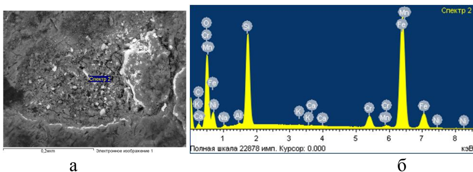
Рис. Б.5 – Хімічний аналіз поверхні тертя базового чавуна ЧХ22Н2 при рН 5 та абразивності 10% спектр 2:
