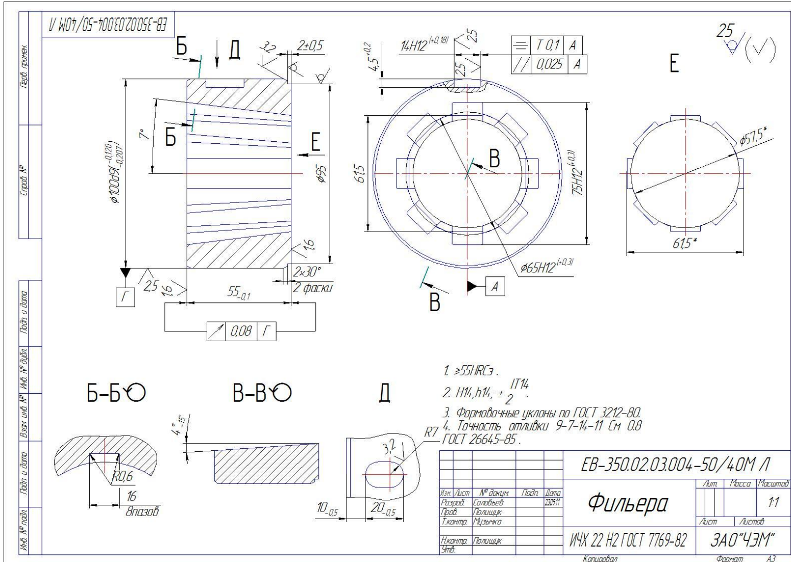
Рис. А6 – Філь'єра EB-350.02.03.004-50/40M L
