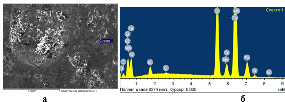
Рис. Б.29 – Хімічний аналіз поверхні тертя базового чавуна ЧХ22Н2 при рН 8 та абразивності 10% спектр 1: а – мікрофотографія поверхні тертя при збільшенні 0,2 мкм; б – металографічна діаграма
