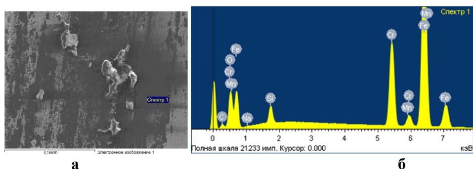
Рис. Б.9 – Хімічний аналіз поверхні тертя підбраного чавуна ЧХ32 при рН 5 та абразивності 10% спектр 1:
