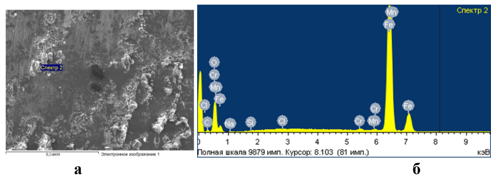
Рис. Б.23 – Хімічний аналіз поверхні тертя базової сталі 40X при рН 8 та абразивності 10% спектр 2:
