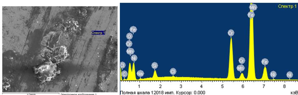
Рис. Б.33 – Хімічний аналіз поверхні тертя підбраної сталі 95X18 при рН 11 та абразивності 10% спектр 1:
