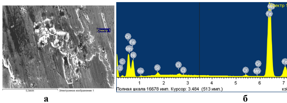
Рис. Б.36 – Хімічний аналіз поверхні тертя базової сталі 40X при рН 11 та абразивності 10% спектр 1:
