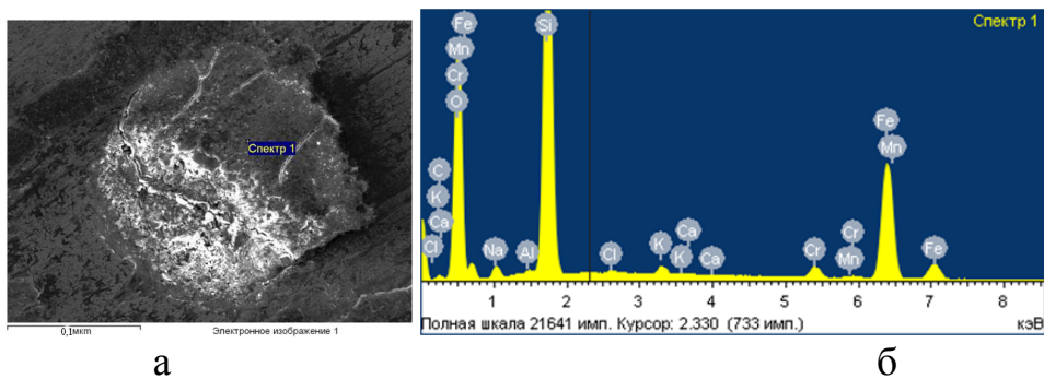
Рис. Б.6 – Хімічний аналіз поверхні тертя базового чавуна ЧХ22Н2 при рН 5 та абразивності 10% спектр 1:
