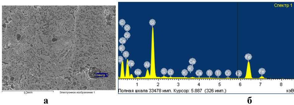
Рис. Б.17 – Хімічний аналіз поверхні тертя базової сталі 40X при рН 5 та абразивності 10% спектр 1:
