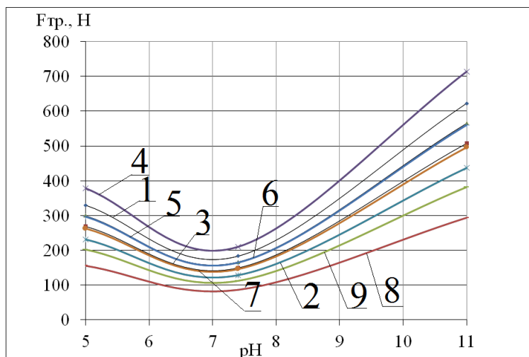
Рис. 3.10 – Залежності сили тертя трібосистем від рівня активної кислотності при постійному навантаженні та абразивності:
