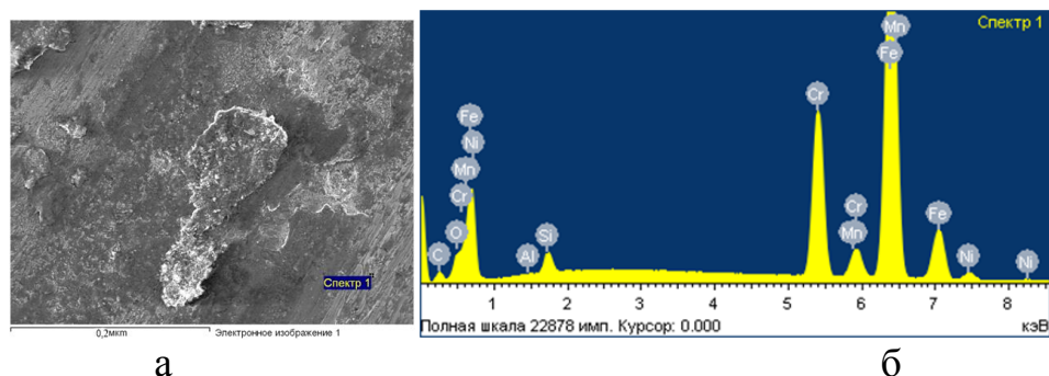
Рис. Б.1 – Хімічний аналіз поверхні тертя базового чавуна ЧХ22Н2 при рН 5 та абразивності 10% спектр 1:
