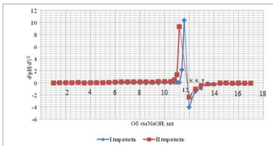
Рис. 3.3. Диференціальна крива титрування II порядку деревинної жижки 0,1 нормальним розчином гідроксиду натрію
