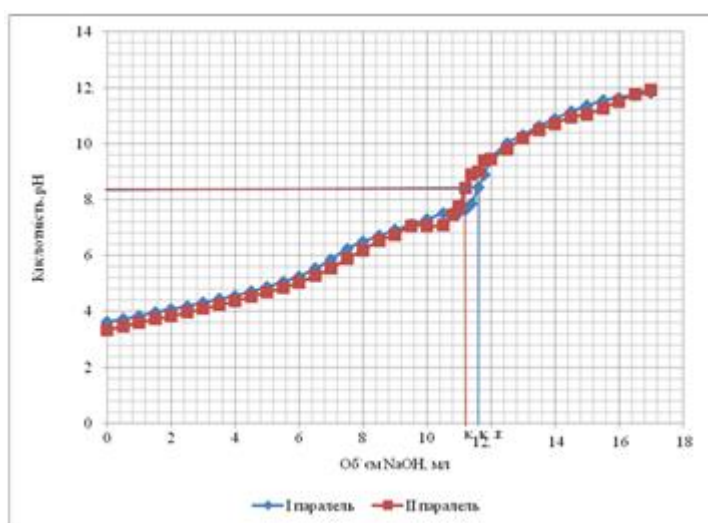
Рис. 3.1 – Інтегральна крива титрування деревинної жишки 0,1 нормальним розчином гідроксиду натрію
