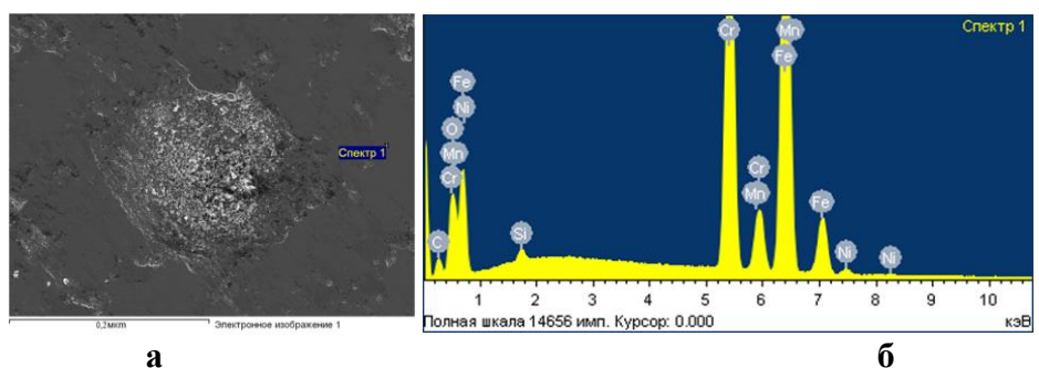
Рис. Б.39 – Хімічний аналіз поверхні тертя базового чавуна ЧХ22Н2 при рН 11 та абразивності 10% спектр 1:
