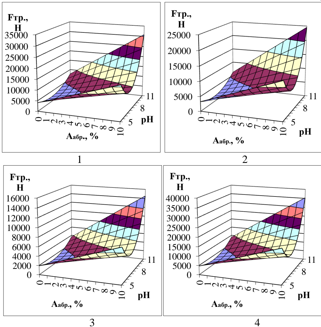
Рис. 4.6 – Розрахункові значення сили тертя натурної трібосистеми екструдера ЕВ-350, «хвостовик – філь’ера №4»:
