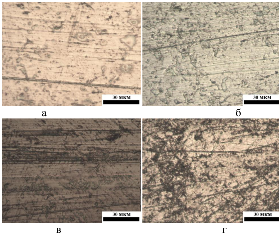
Рис. 5.1 – Мікрофотографії поверхонь тертя сталей при використанні слабокислого середовища, рН 5, без абразиву (x600): а – сталь 40Х; б – чавун ЧХ22Н2; в – сталь 95Х18; г – чавун ЧХ32
