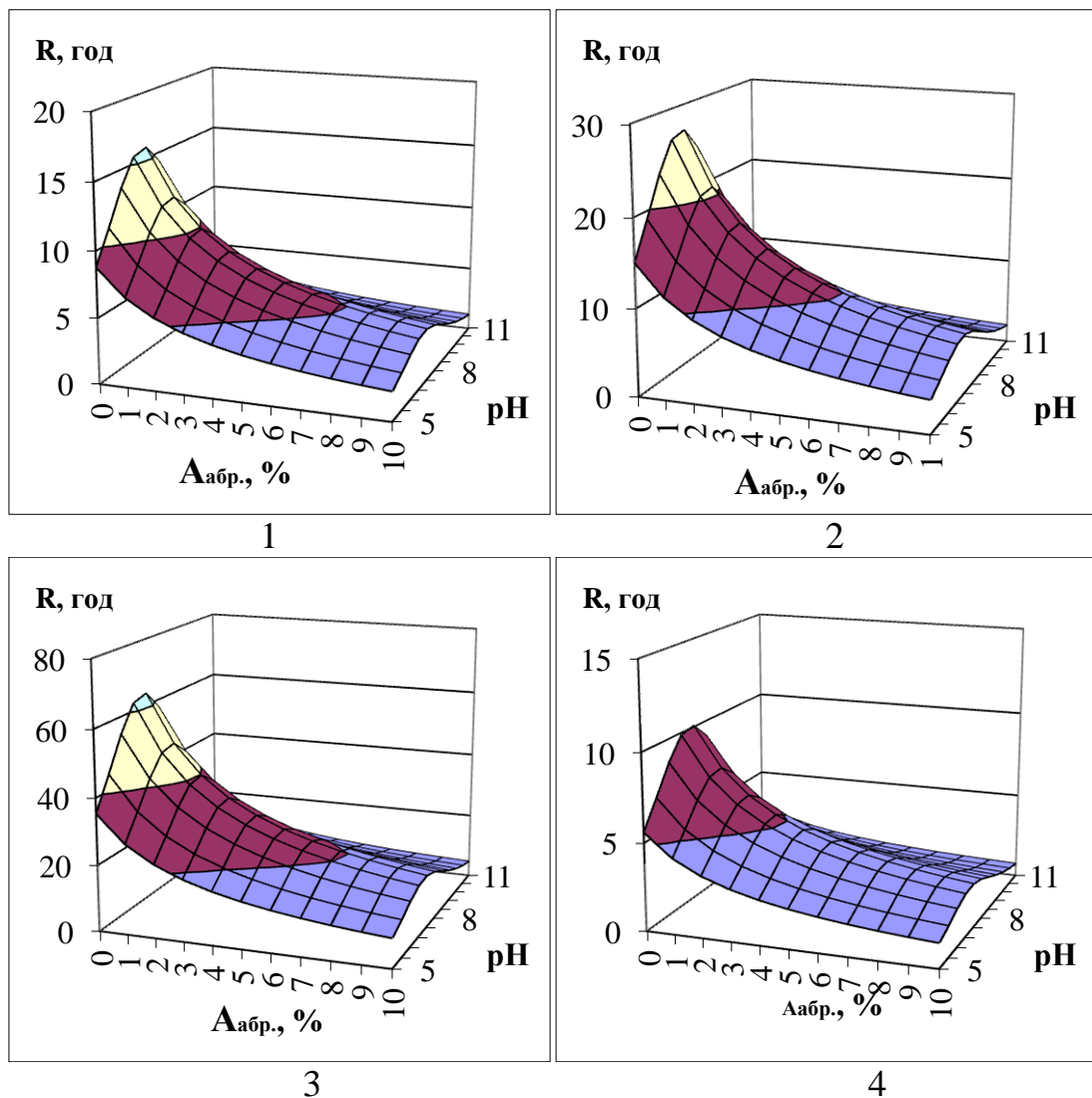
Рис. 4.9 – Розрахункові значення ресурсу натурної трібосистеми екструдера ЕВ-350, «наконечник – філь'єра №5»:
