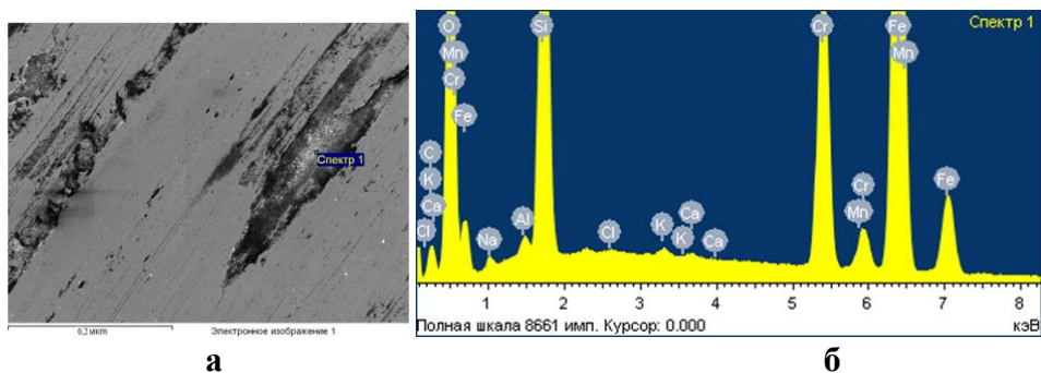
Рис. Б.19 – Хімічний аналіз поверхні тертя підбіраної сталі 95X18 при рН 5 та абразивності 10% спектр 1:
