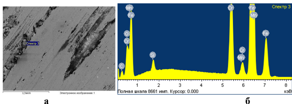
Рис. Б.21 – Хімічний аналіз поверхні тертя підбраної сталі 95X18 при рН 5 та абразивності 10% спектр 3:
