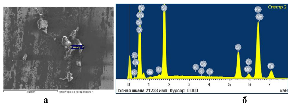
Рис. Б.10 – Хімічний аналіз поверхні тертя підбраного чавуна ЧХ32 при рН 5 та абразивності 10% спектр 2:
