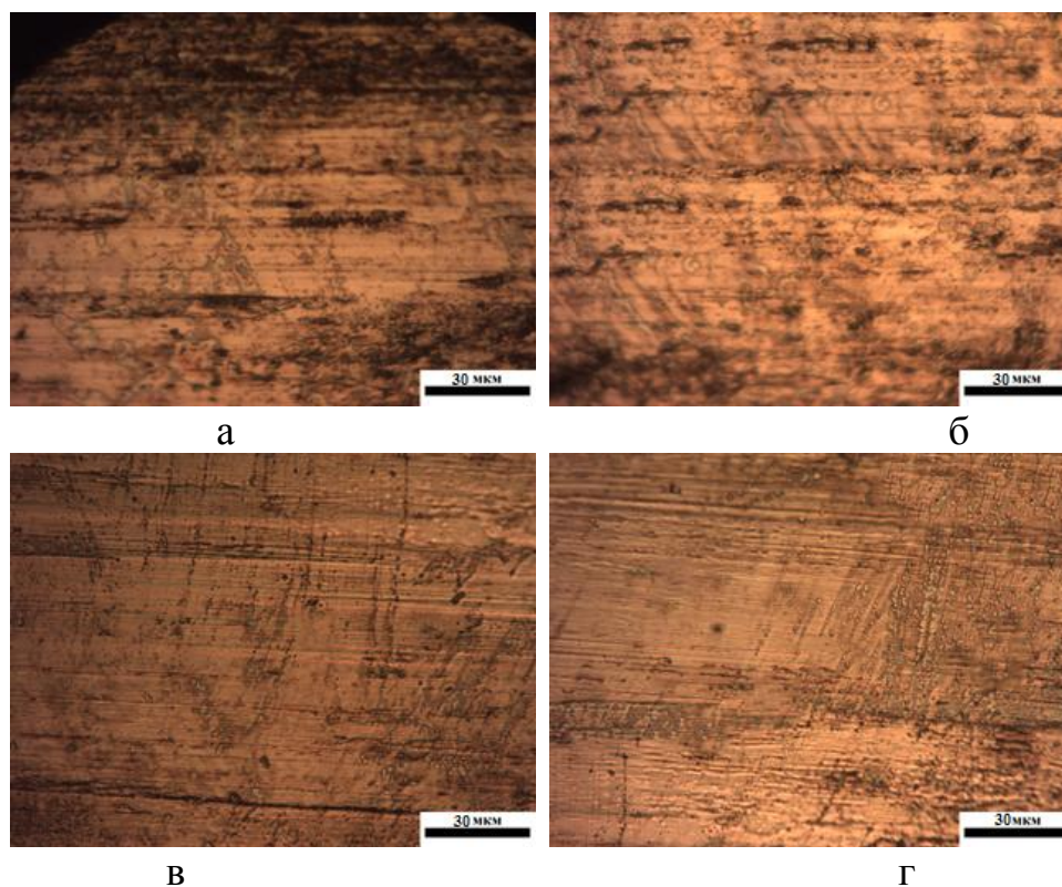
Рис. 5.3 – Мікрофотографії поверхонь тертя сталей при використанні слаболужного середовища, рН 8, без абразиву (х600):
