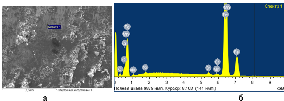
Рис. Б.22 – Хімічний аналіз поверхні тертя базової сталі 40X при рН 8 та абразивності 10% спектр 1:
