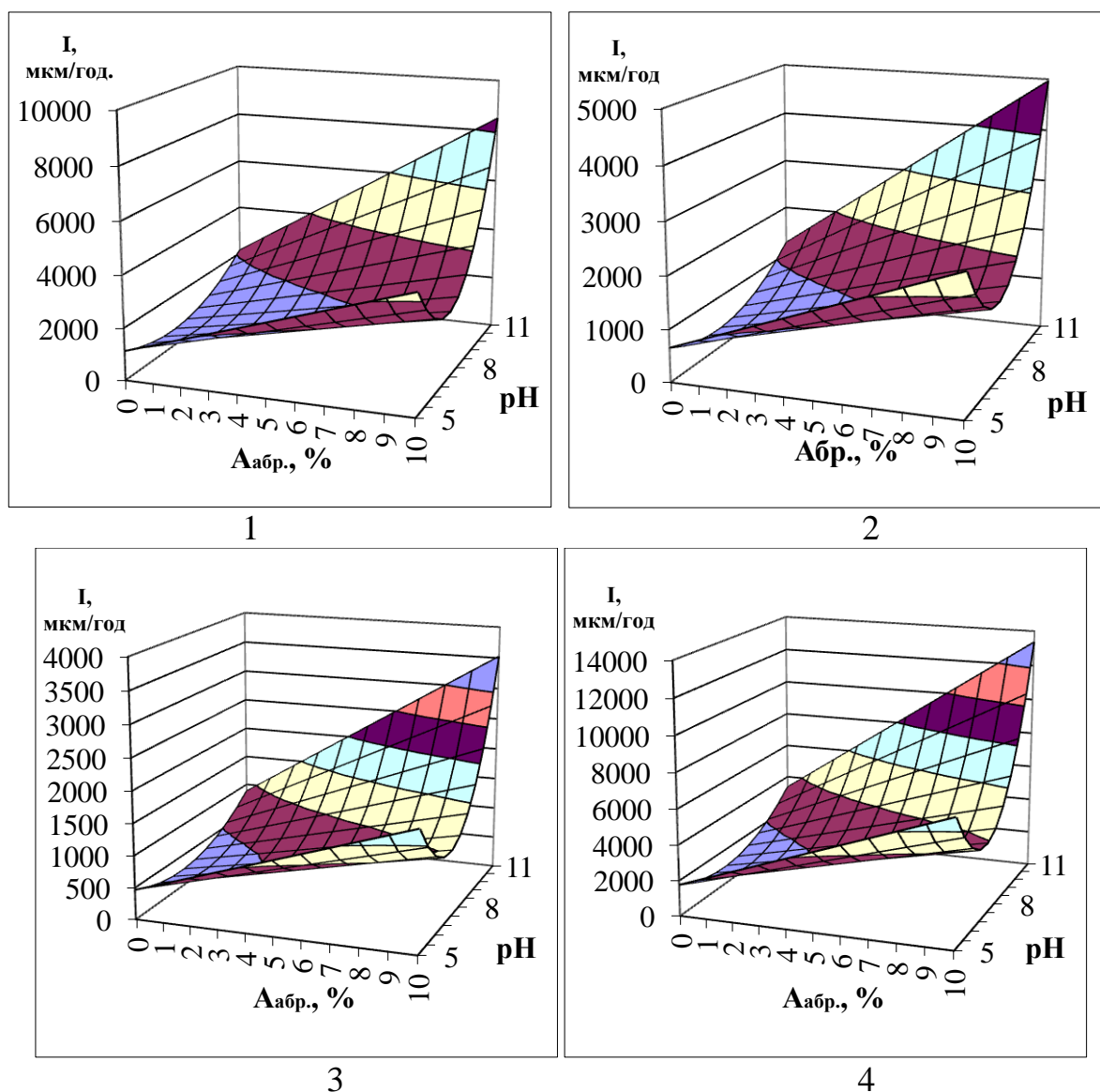
Рис. 4.3 – Розрахункові значення швидкості зношування натурної трібосистеми екструдера ЕВ-350, «шнек конічний – філь’єра №1, 2 та 3»:
